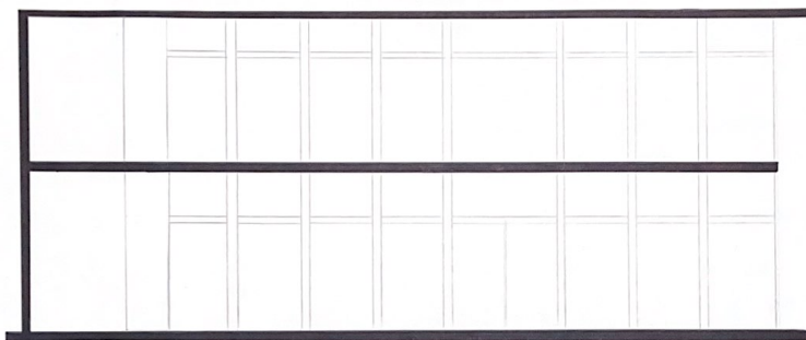
CORTE LONGITUDINAL esc. 1:50
