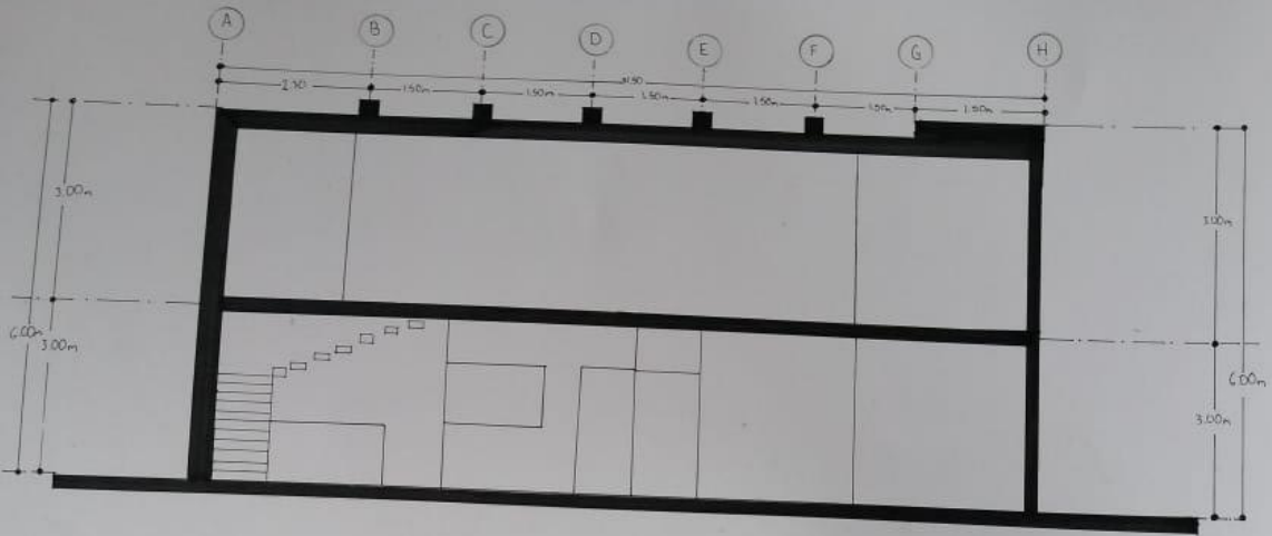
CORTE LONGITUDINAL ESC. 1:50
