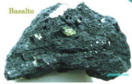
3. Rocas ígneas, sedimentarias y metamórficas
