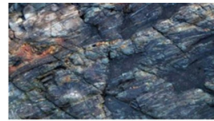
Sienita. Muy parecida al granito, pero con muy poca cantidad de cuarzo.
