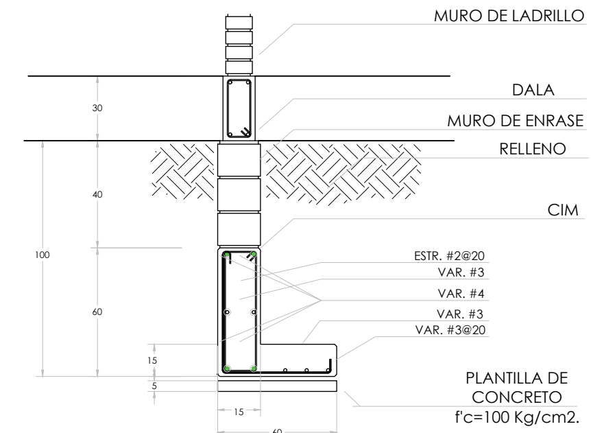
ZAPATA COLINDANTE EXT. ZC-1
