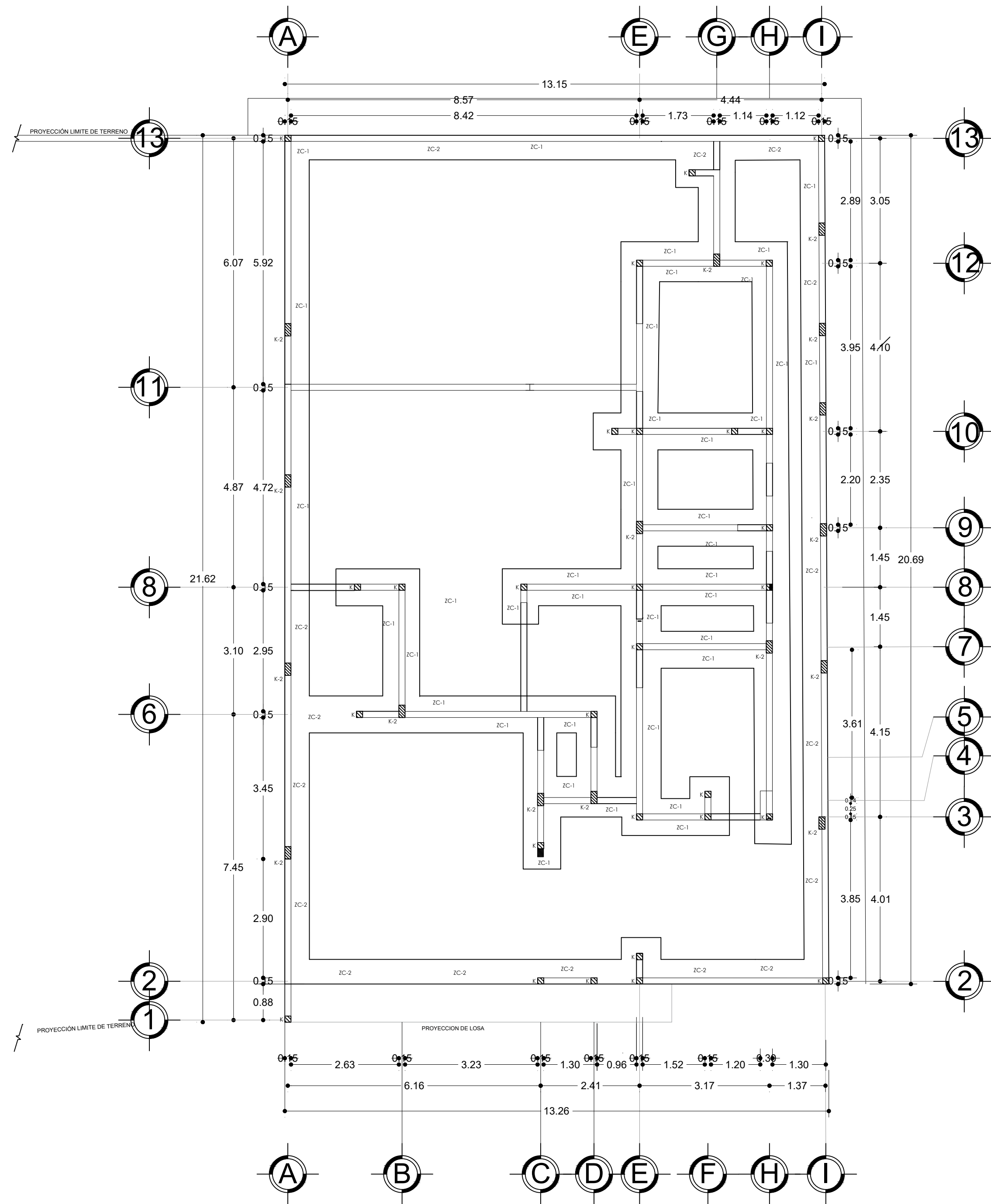
PLANO DE CIMENTACION PLANTA BAJA ESC: 1:75
