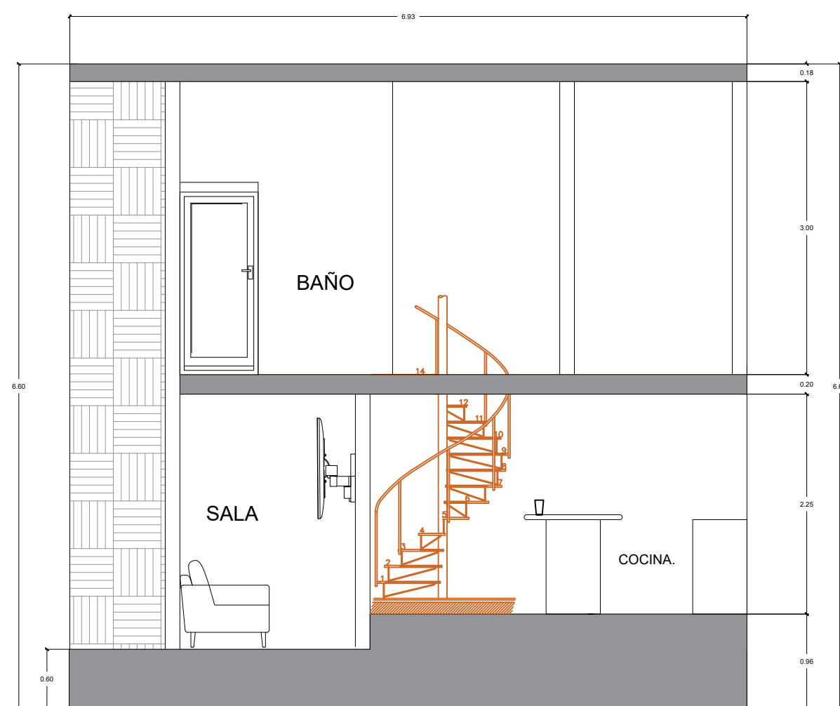
CORTE Y-1
