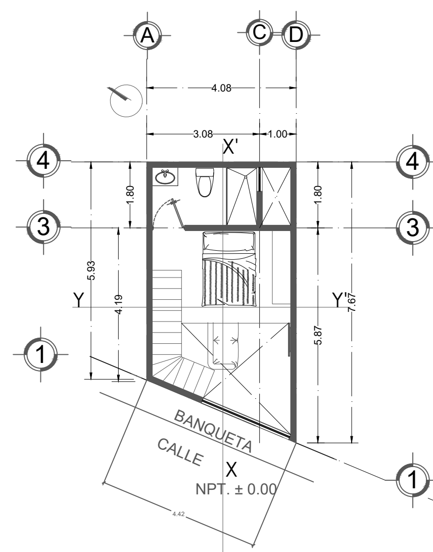
Planta Arquitectónica Planta Alta
