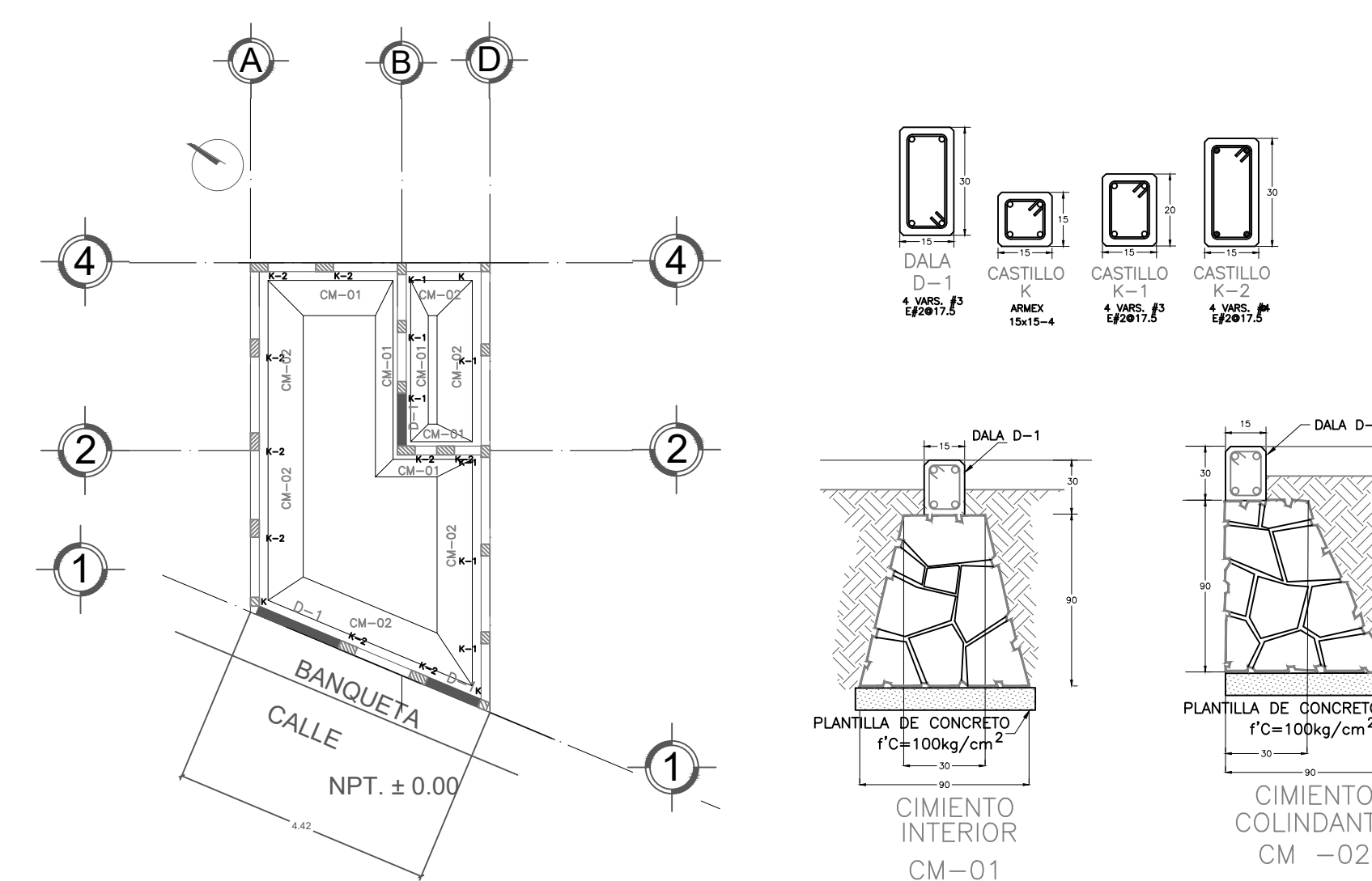
Plano de cimentación
