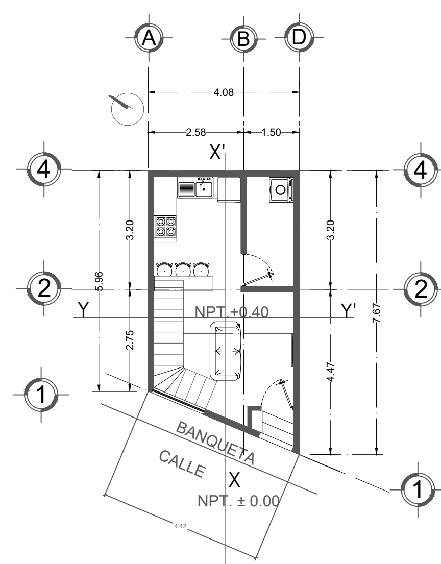
Planta Arquitectónica Planta Baja
