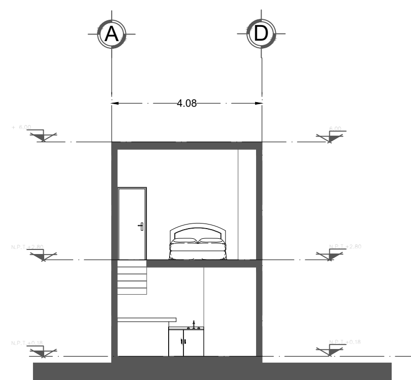
CORTE Y - Y'
