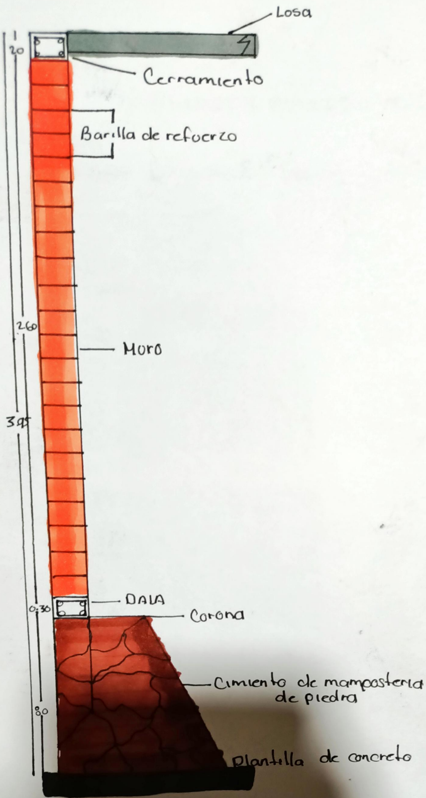
Muro de Block Cimiento de piedra
