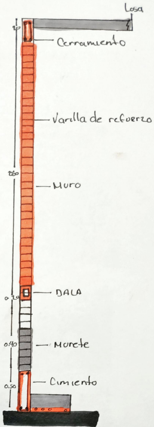
ZAPATA CORIDA - Ladrillo Plantilla de cerramiento
