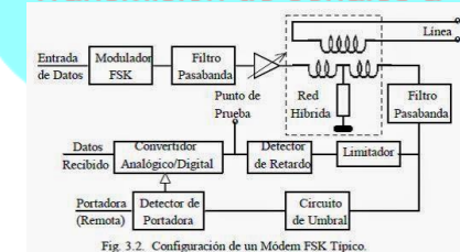
Fig. 3.2. Configuración de un Módem FSK Típico.
