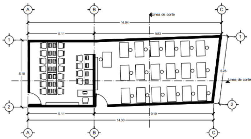
PLANTA ARQUITECTÓNICA ESC. 1:50
