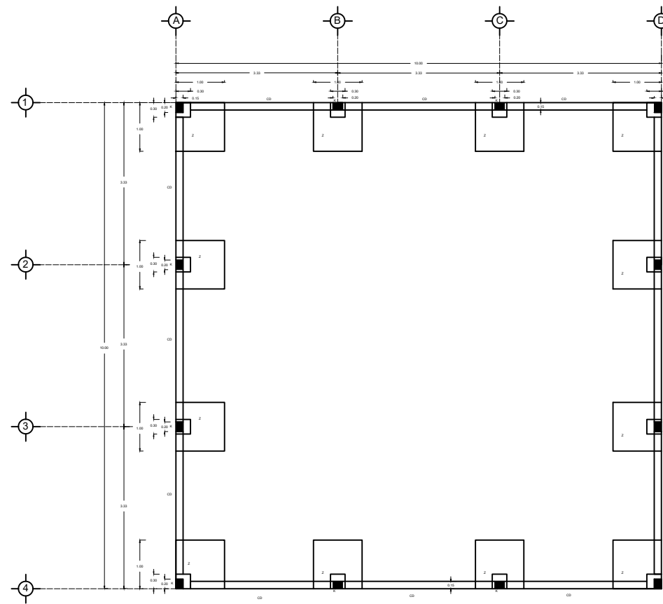
PLANTA ARQUITECTONICA
