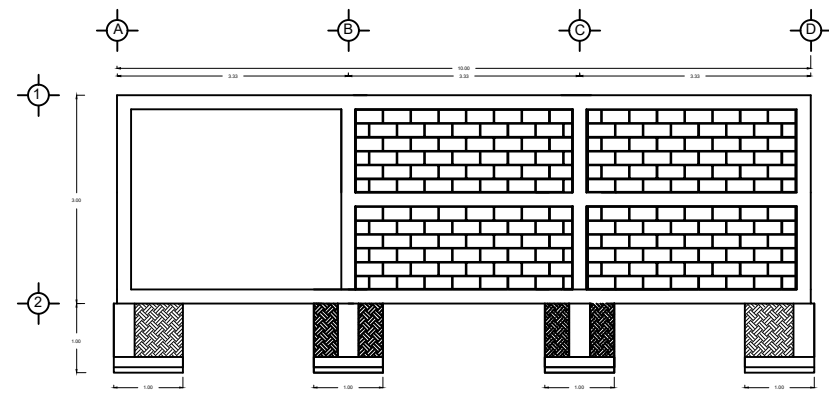
FACHADA POSTERIOR
