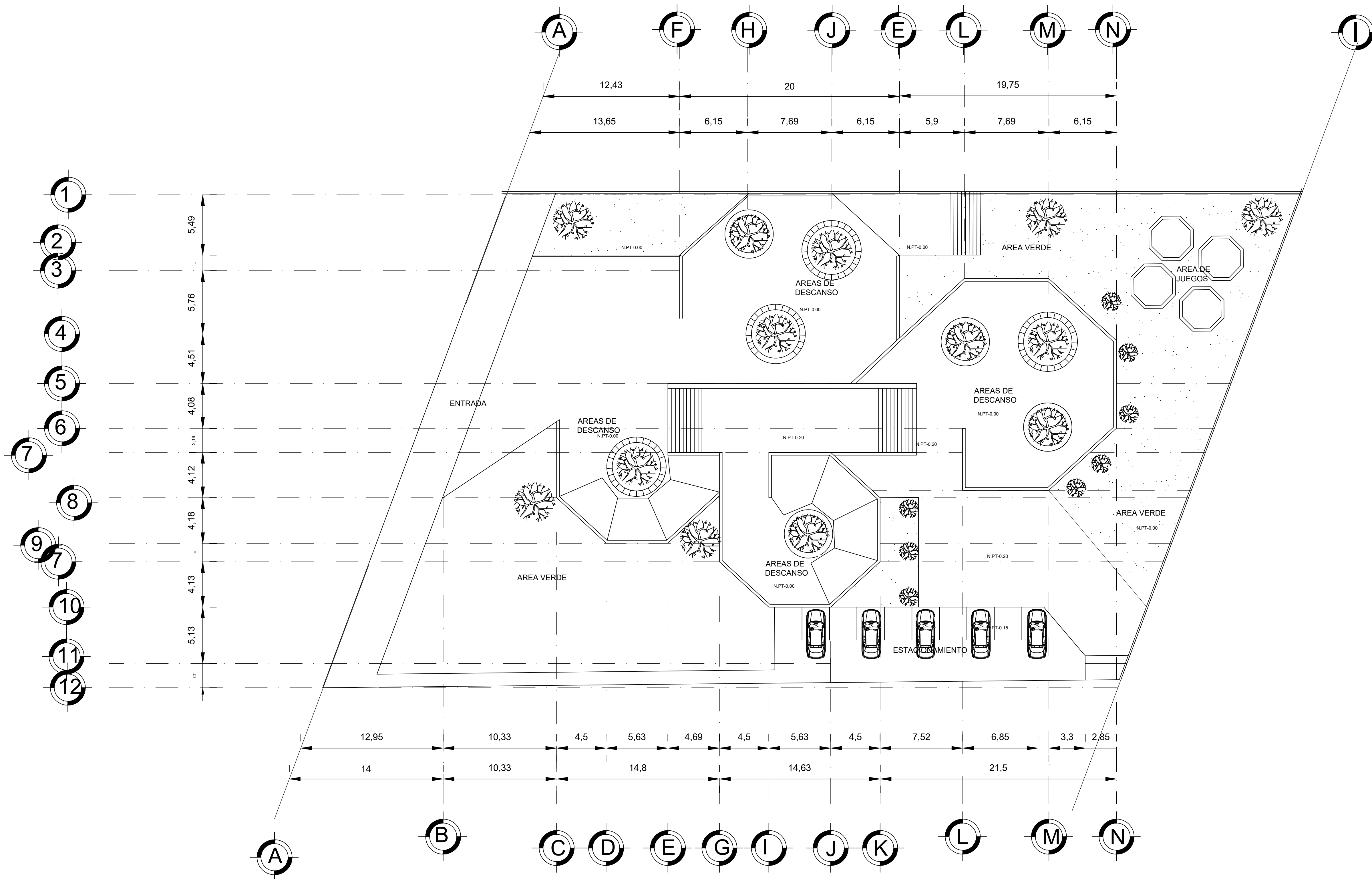
PLANTA ARQUITECTONICA.....ESC: 1.100
