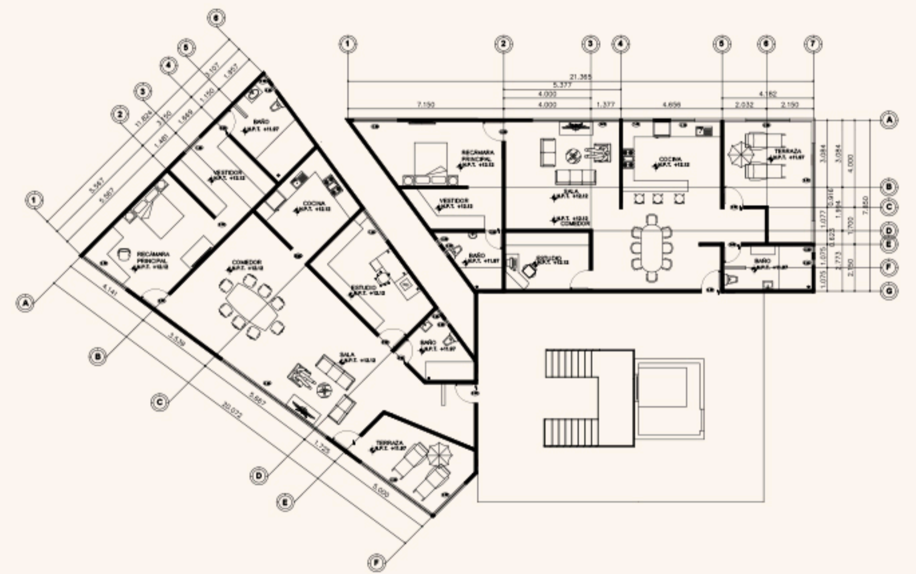
PLANTA BAJA
