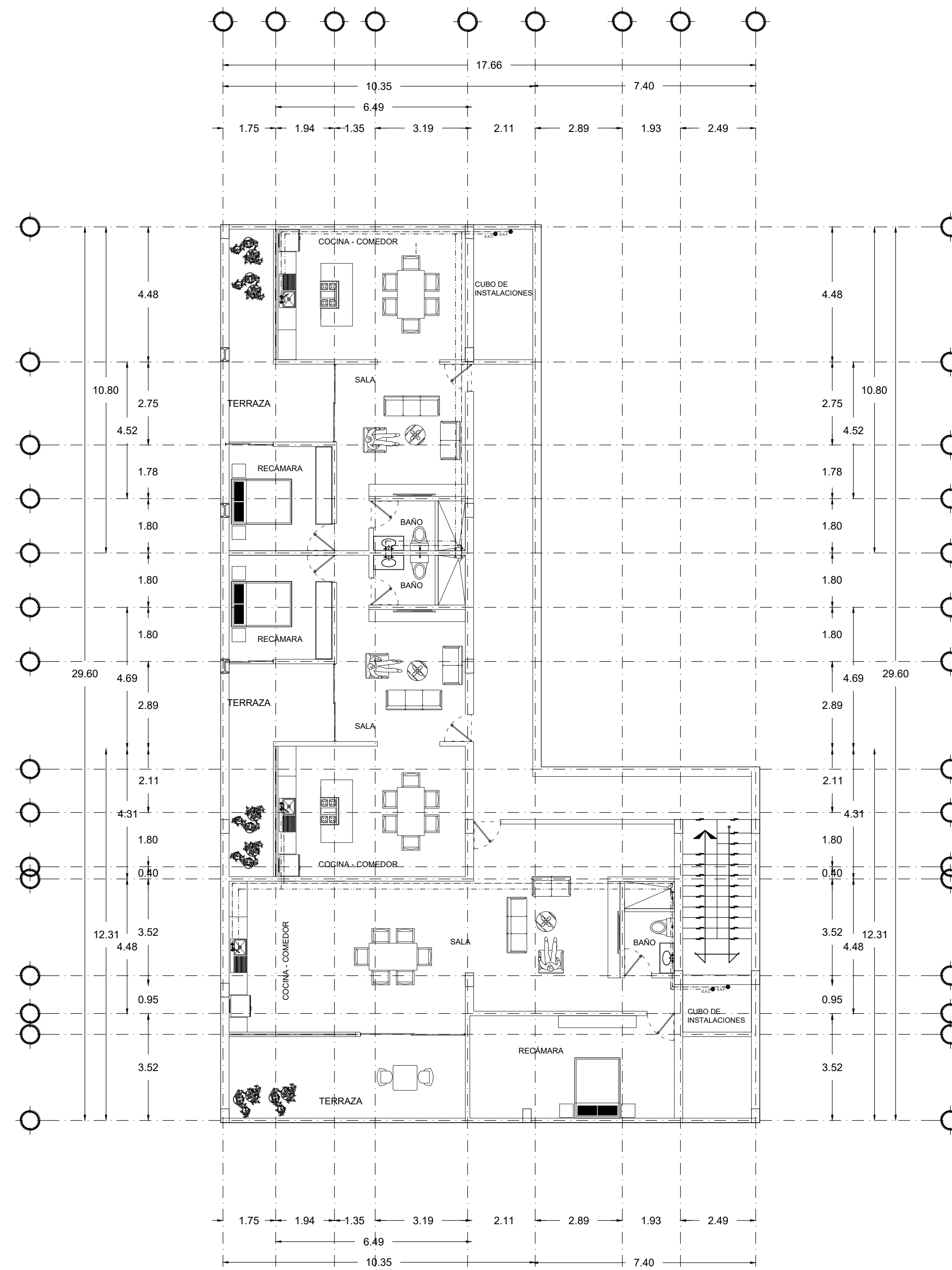
Planta Arquitectónica Departamentos Para parejas
