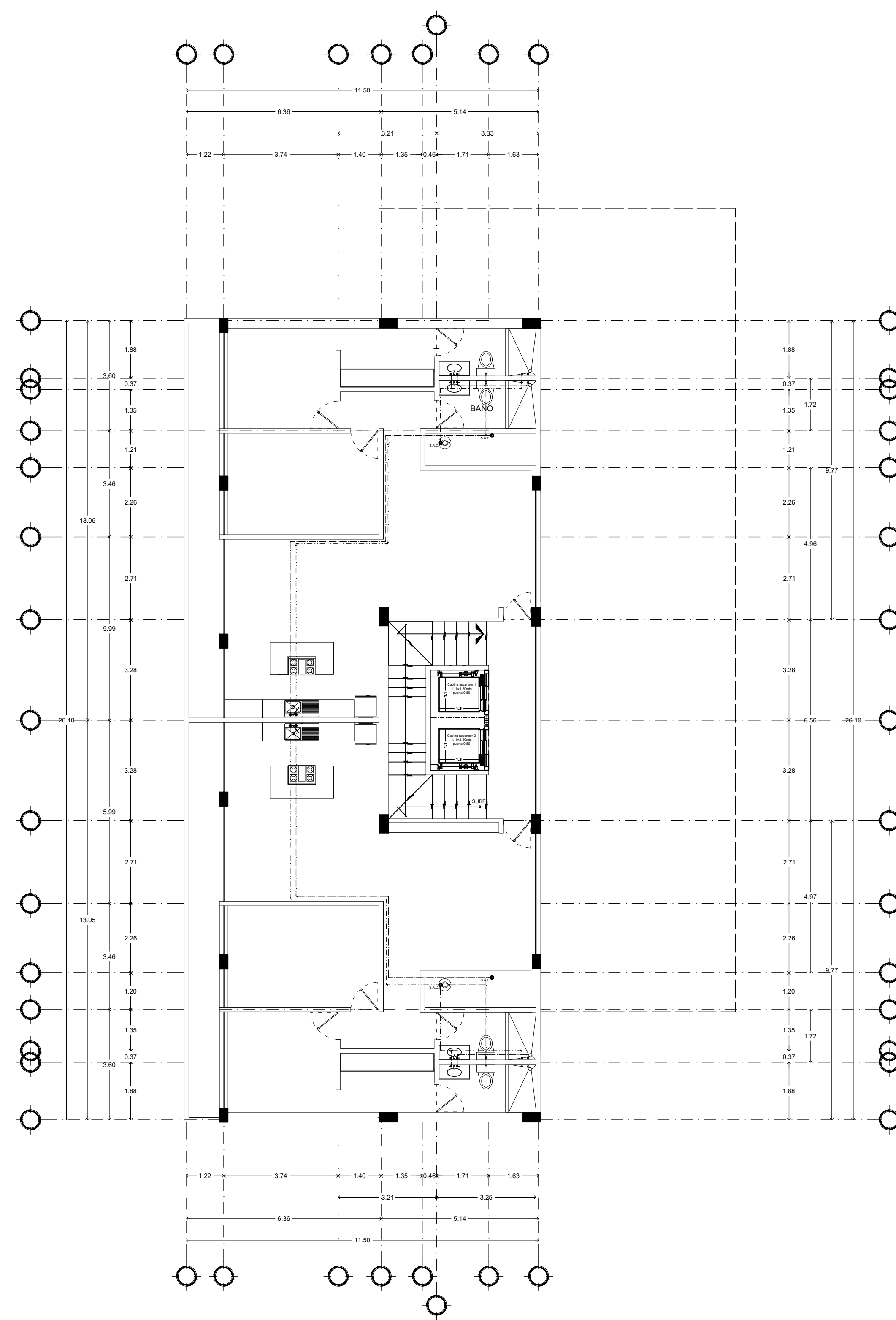
Planta Hidráulica Departamentos Familiares Tipo 3 Esc. 1:100
