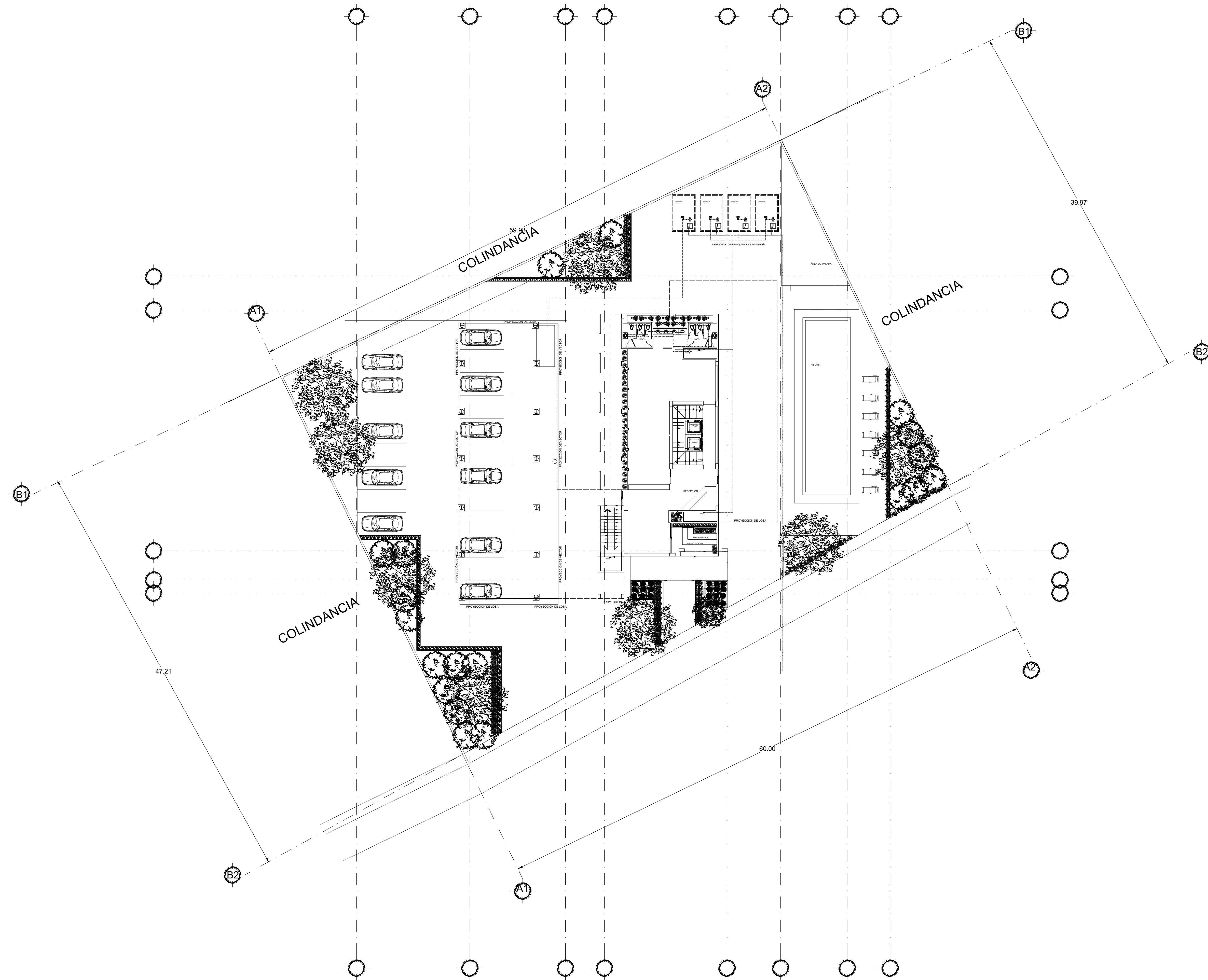
Planta Hidráulica recepción
