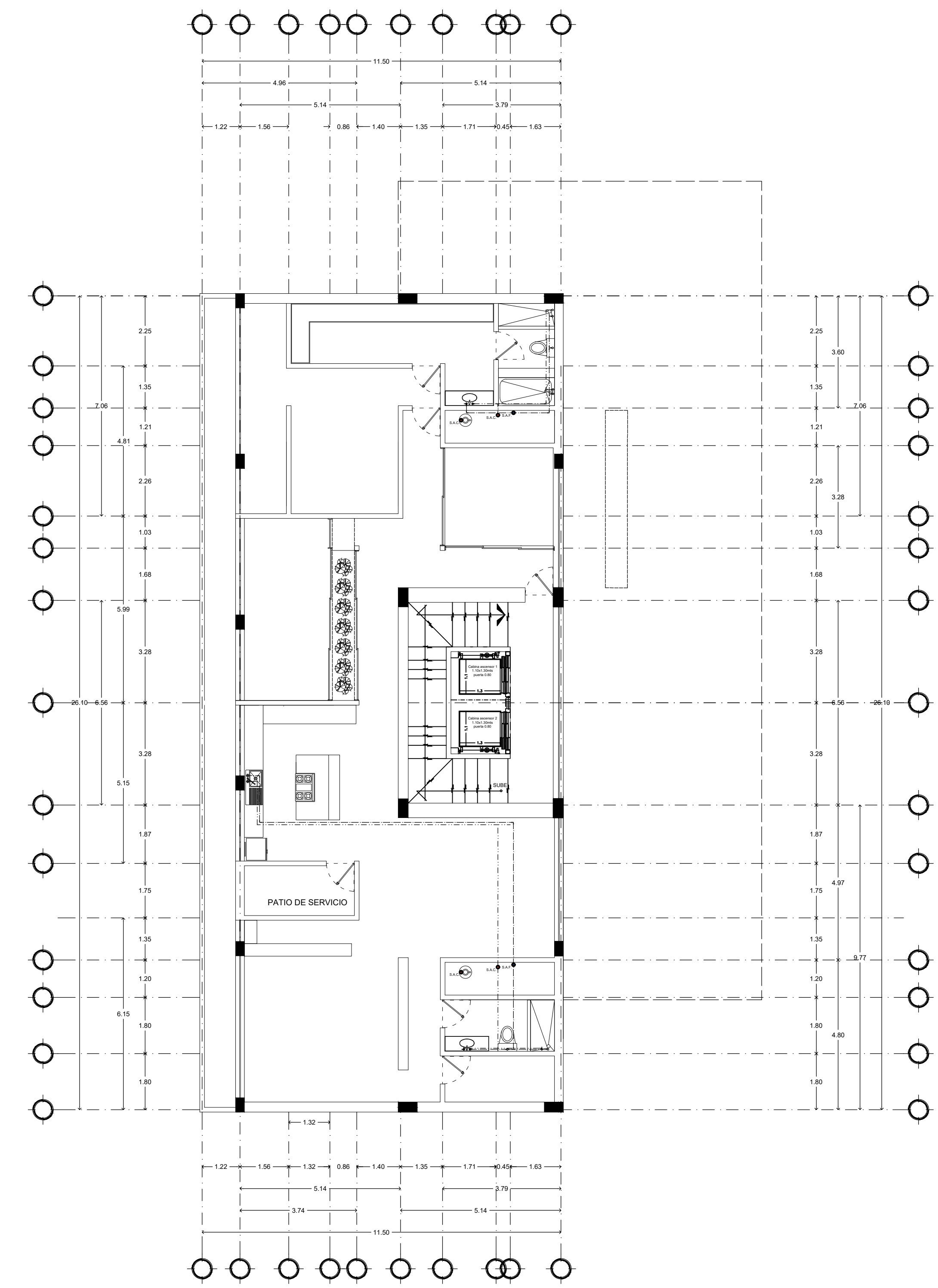
Planta Hidráulica Departamento de Lujo 1 Esc. 1:100
