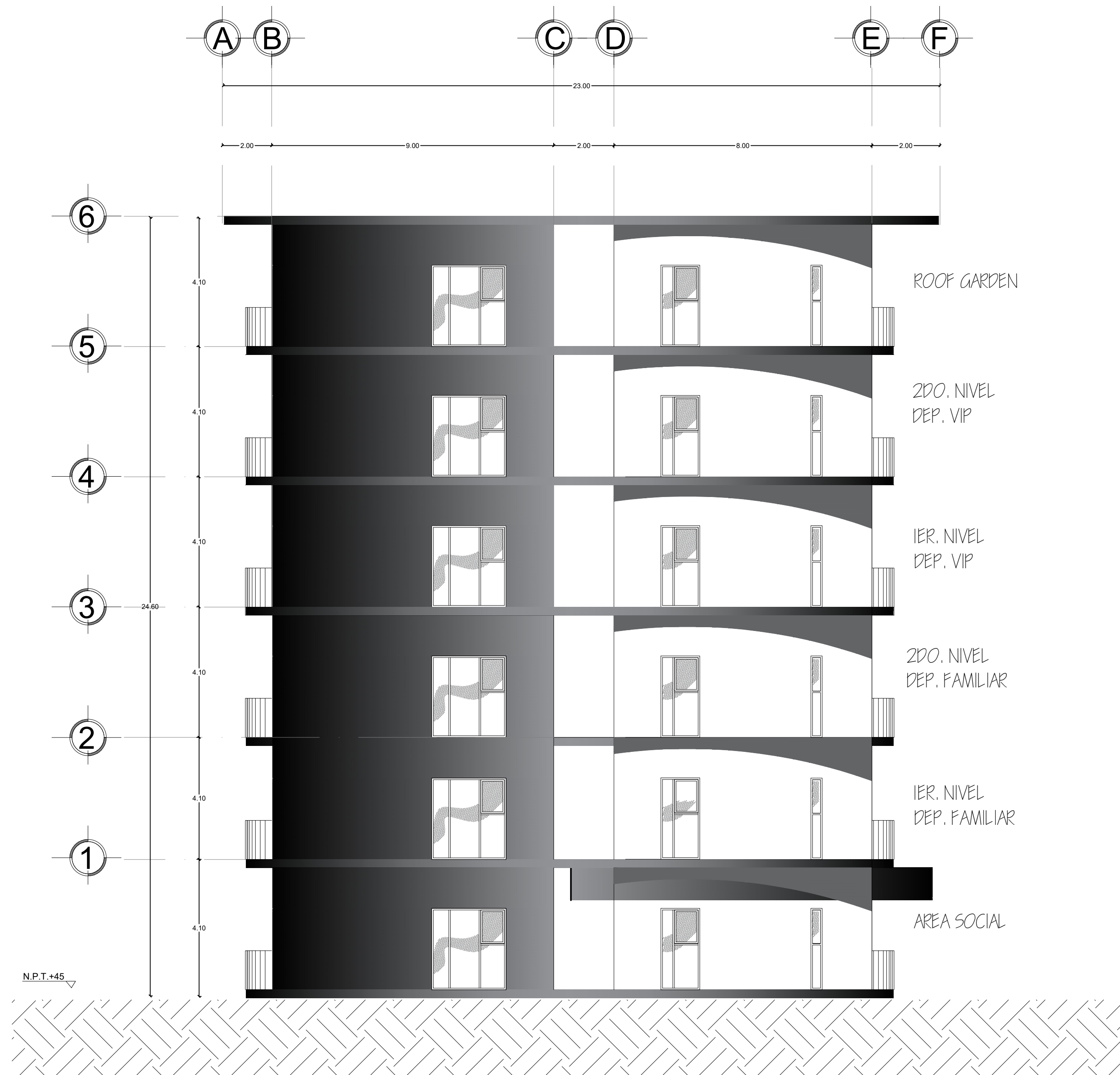
FACHADA ESC 1:100
