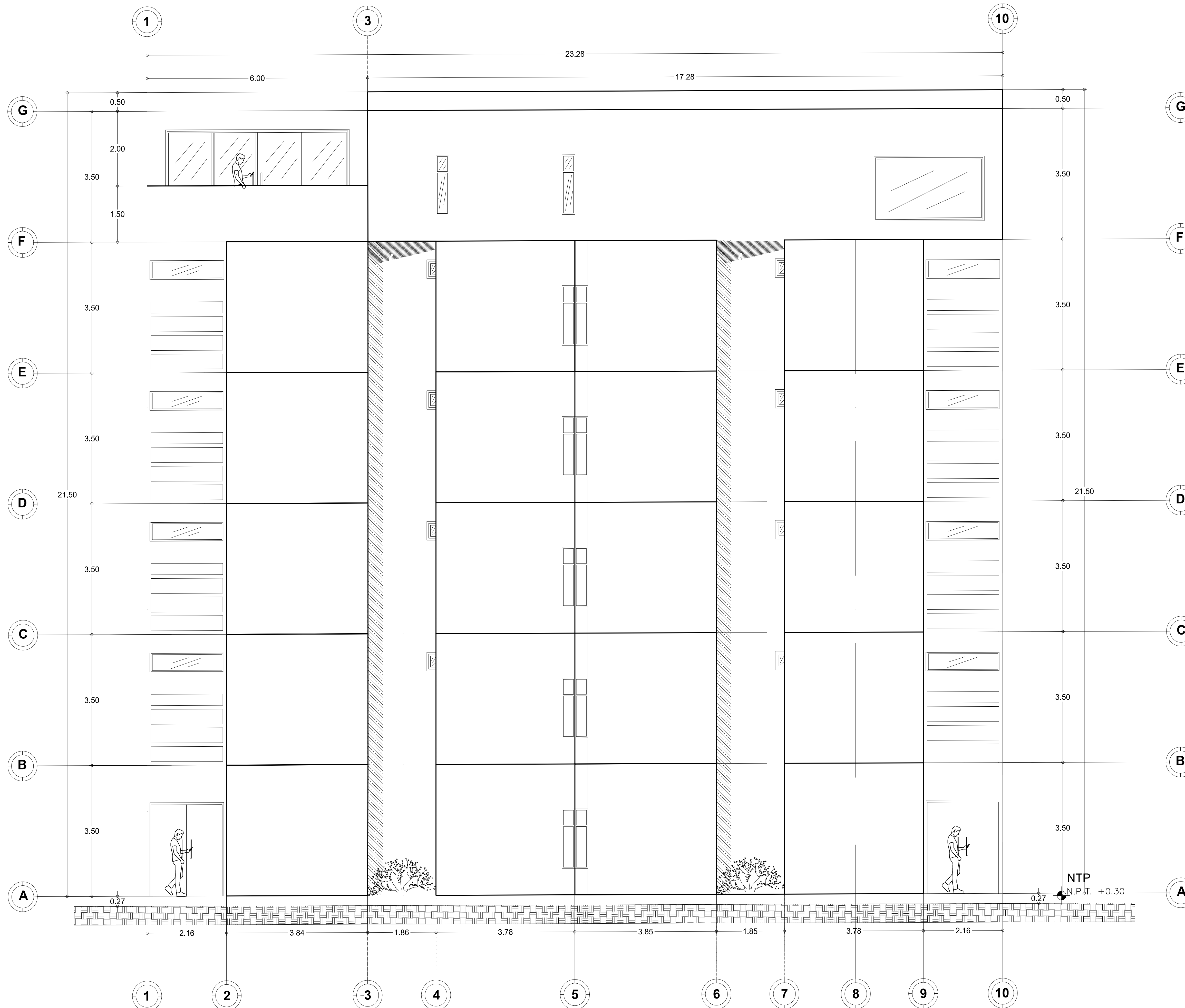
FACHADA PRINCIPAL Esc. 1:50
