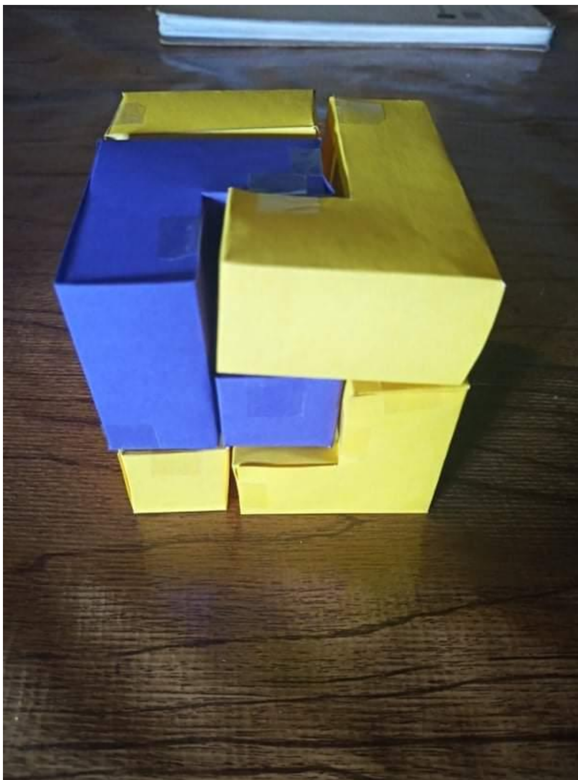
Figura: Cubo 3x3x3
