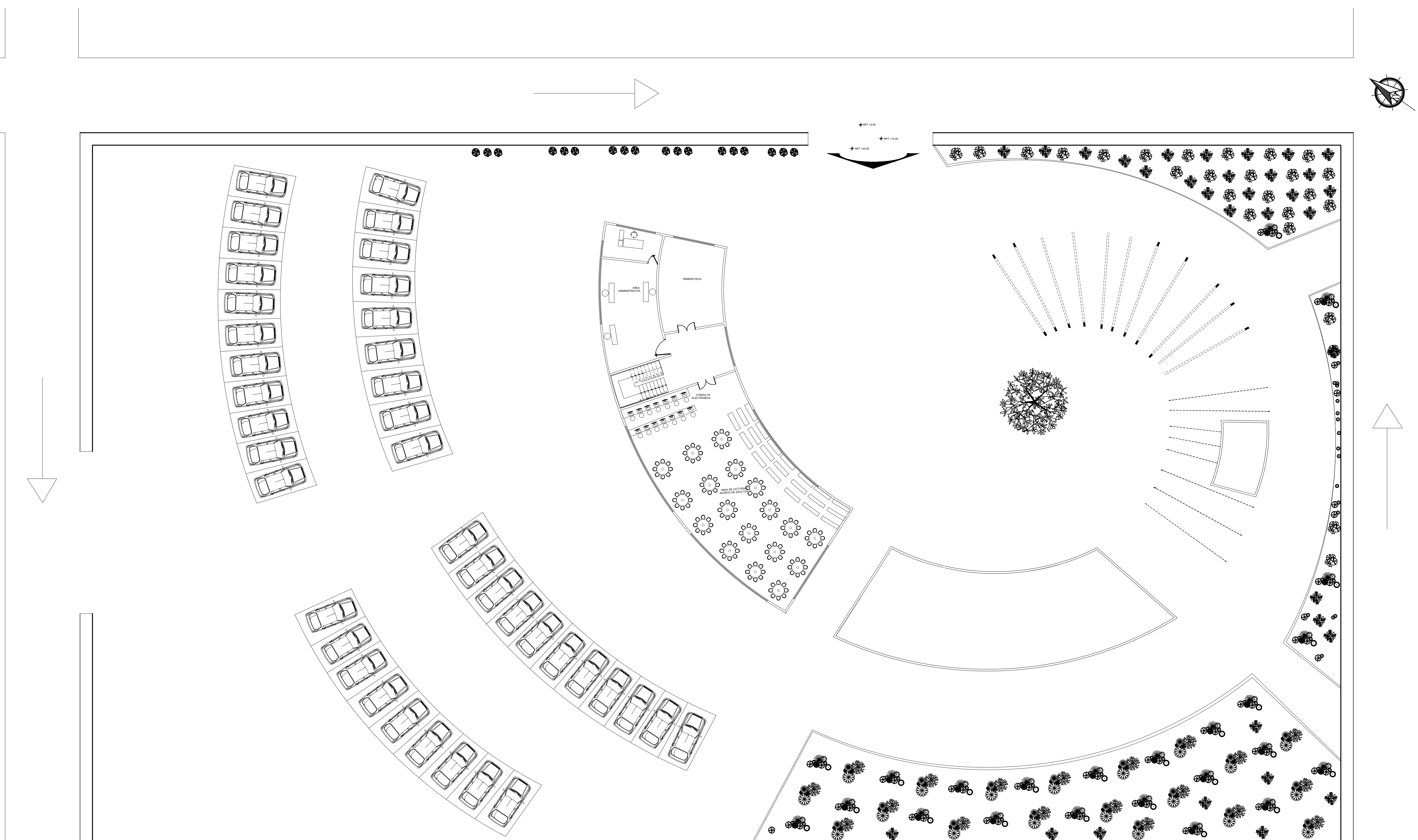
PLANTA ARQUITECTONICA DE CONJUNTO ESC: 1:200
