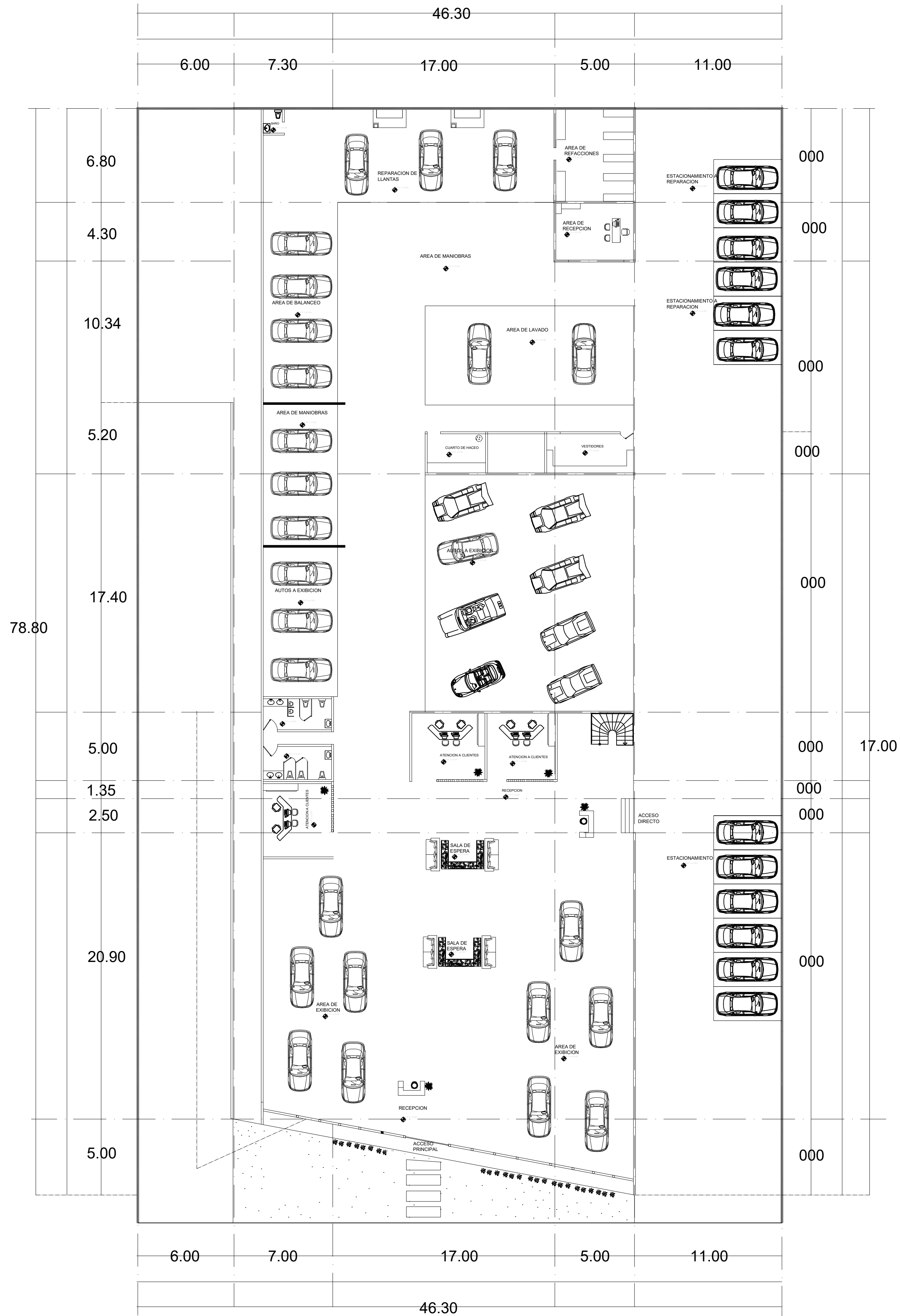
PLANTA ARQUITECTONICA BAJA ESC.....1.100
