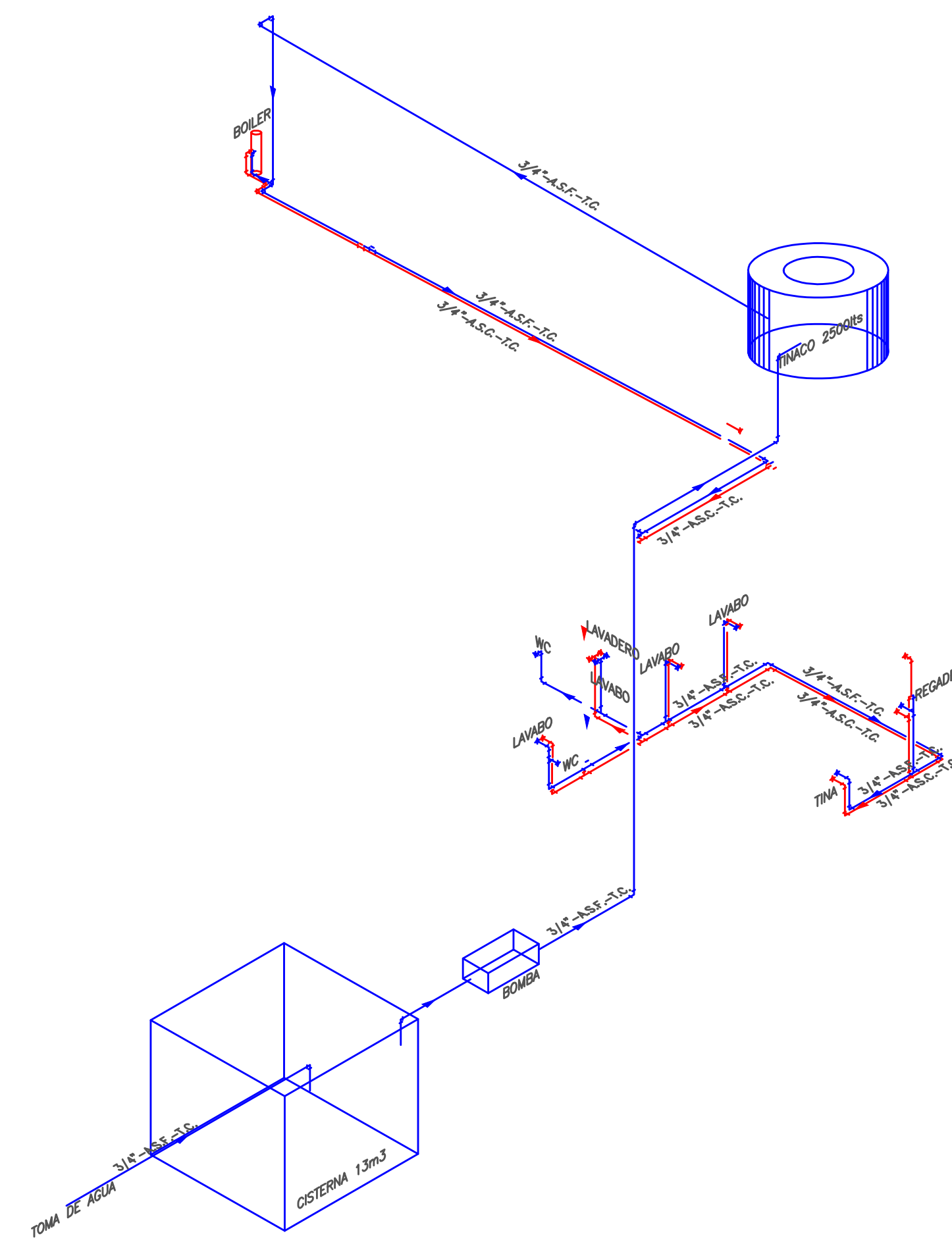
ISOMETRICO INSTALACION HIDRAULICA
