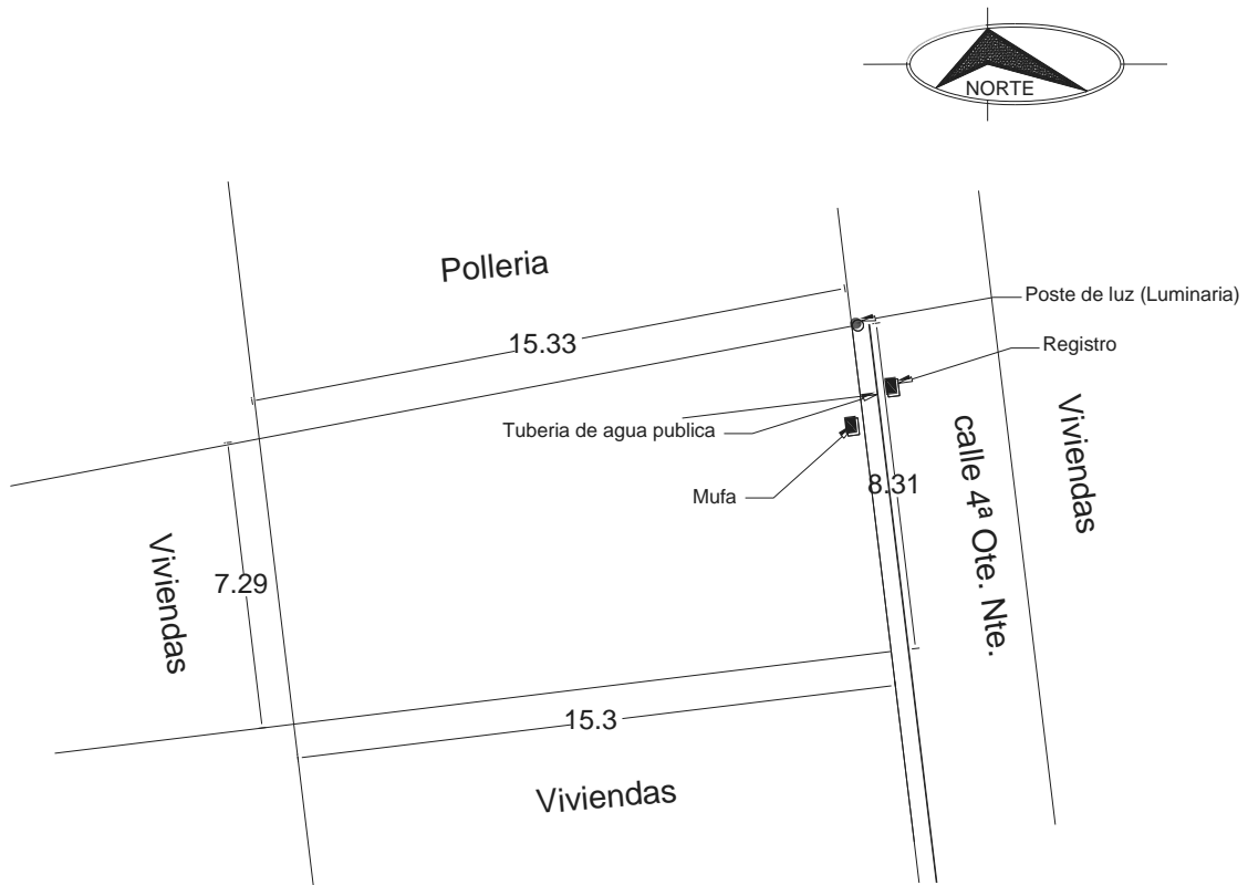
Imagen 33: Plano de servicios públicos
