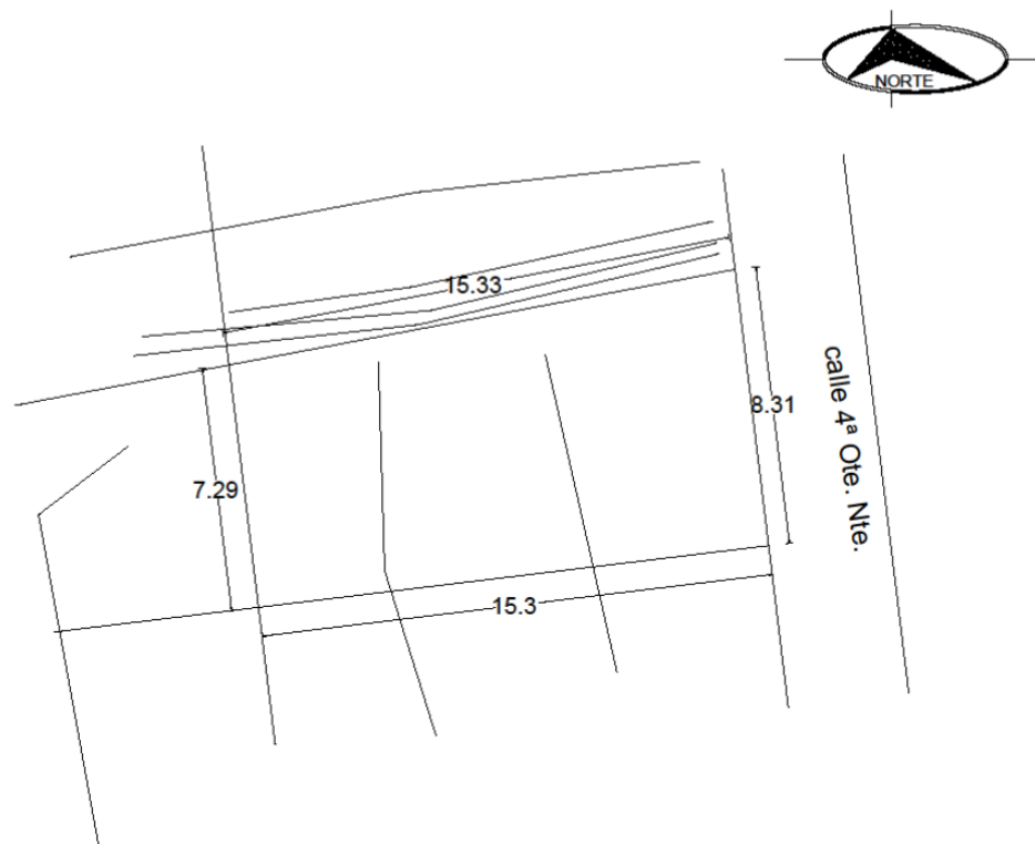
Imagen 24: Plano de curvas de nivel del predio.
