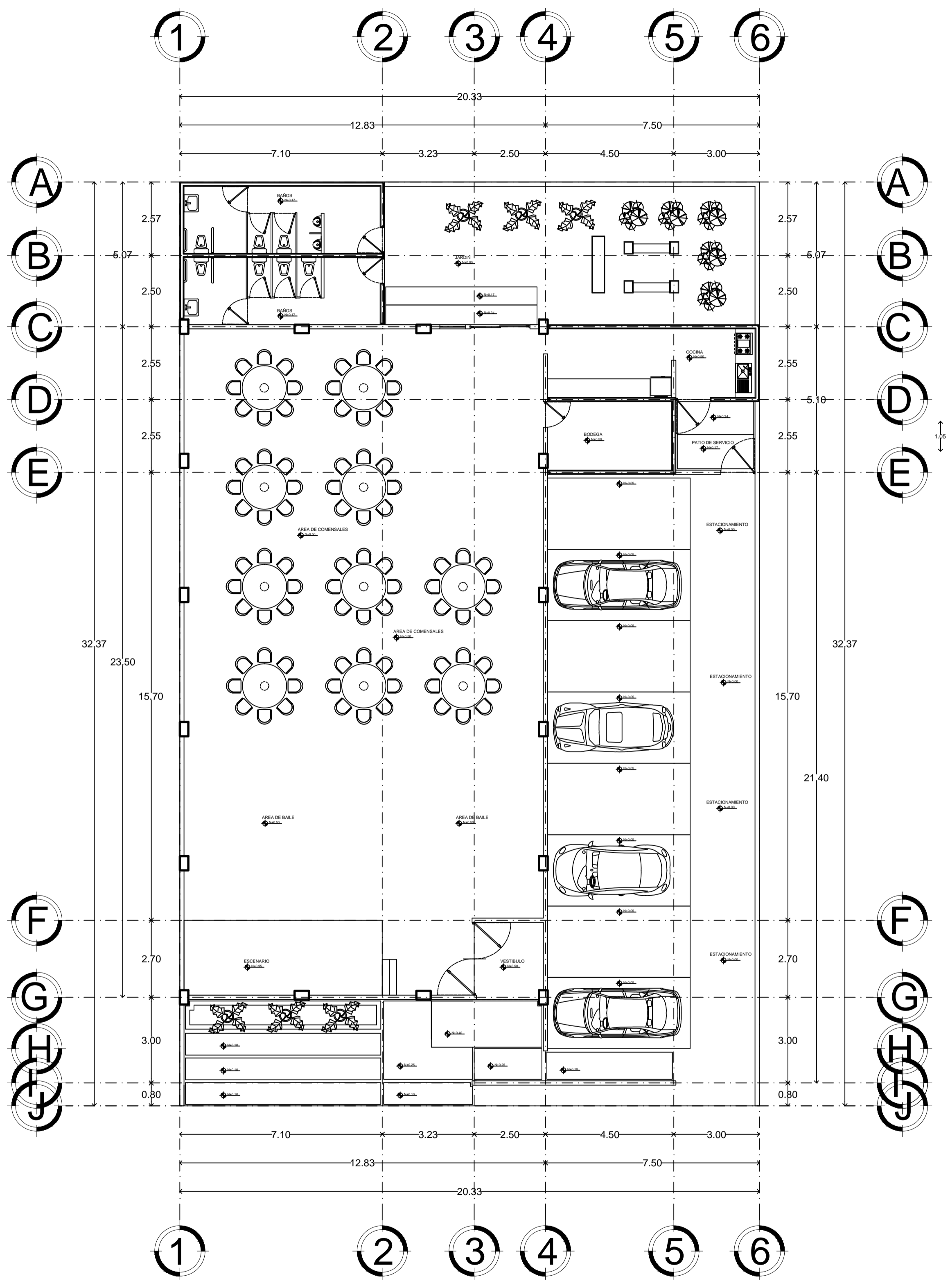
PLANTA ARQUITECTÓNICA
