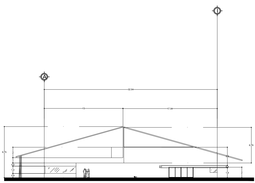
FACHADA TRASERA Esc..... 1:100
