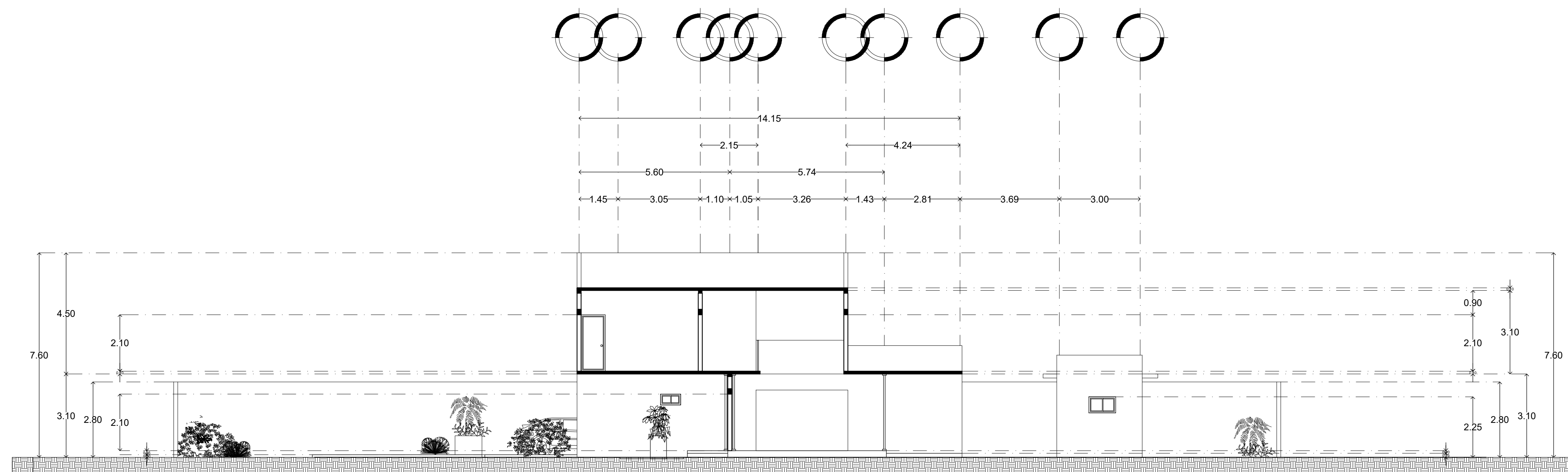
CORTE TRANSVERSAL Y - Y'
