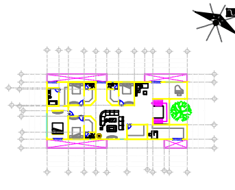
PLANTA ALTA
