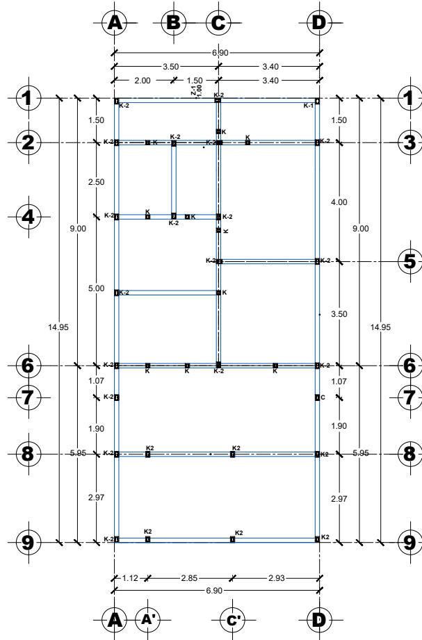
PLANTA DE CASTILLOS
