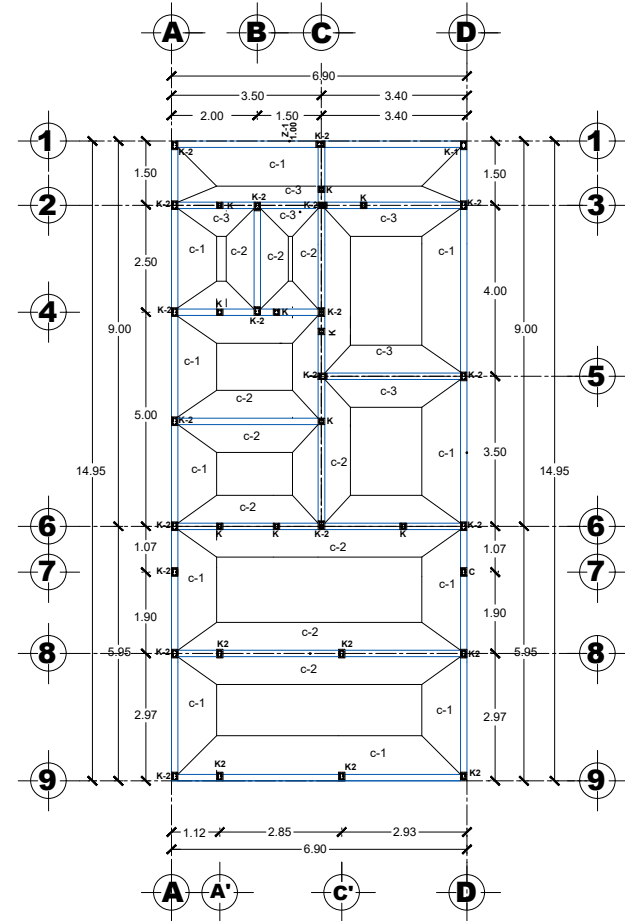
PLANTA DE CIMENTACIONES ZAPATAS
