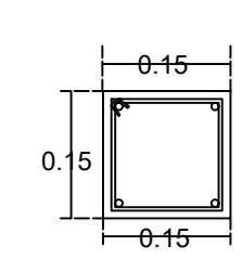
K-1 15X15X0.01=2.25 4 var. #3 Est. #2 @0.075 cm
