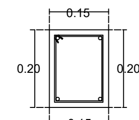
K-2 15X20X0.01=3 4 var. #4 Est. #2 @10 cm
