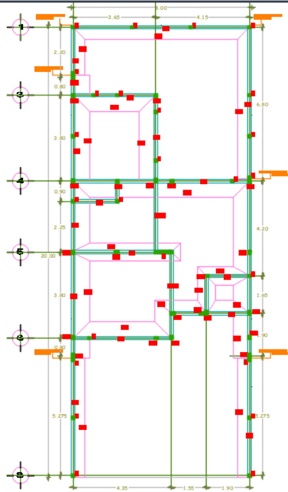
PLANTA DE CIMENTACIÓN
