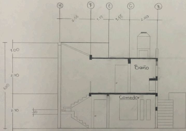
Corte transversal
