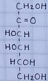
D-tagatosa
