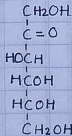
D-fructosa
