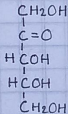
D-ribulosa
