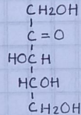
D-xilulosa
