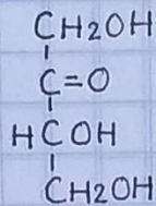
D-eritrosulosa
