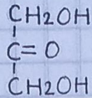
Dihidroxiacetona
