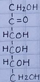
D-psicosa
