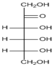
D-(+)-Psicosa
