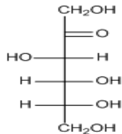
D-(-)-Fructosa
