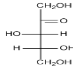
D-(+)-Xilulosa
