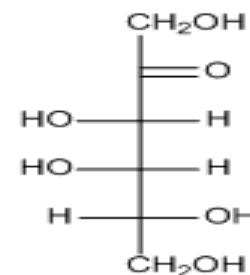
D-(-)-Tagatosa
