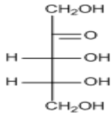
D-(+)-Ribulosa
