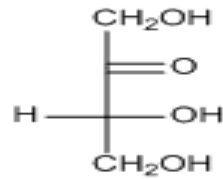
D-(-)-Eritrulosa
