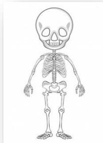
Estructura esquelética
