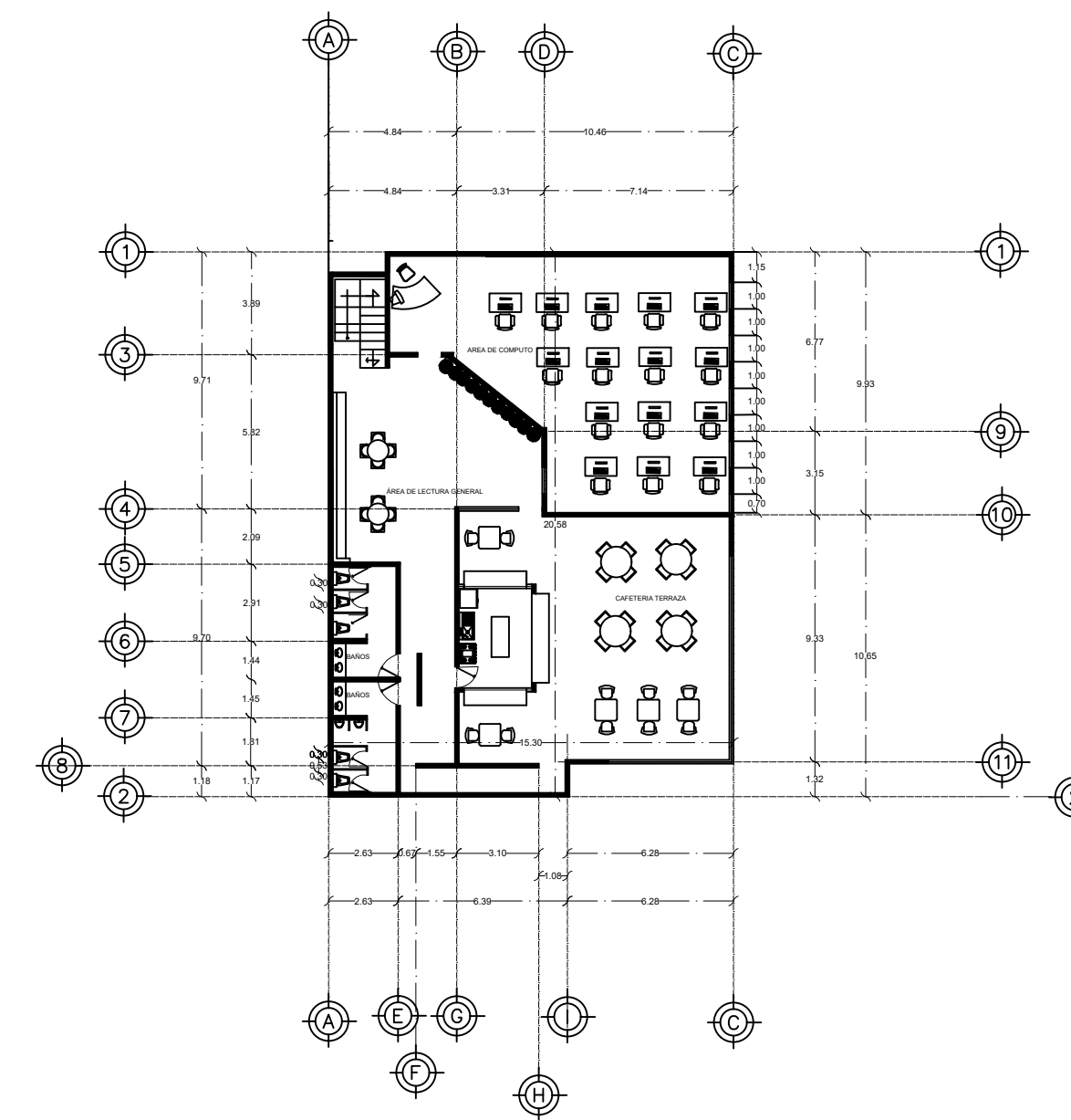
PLANTA ALTA
