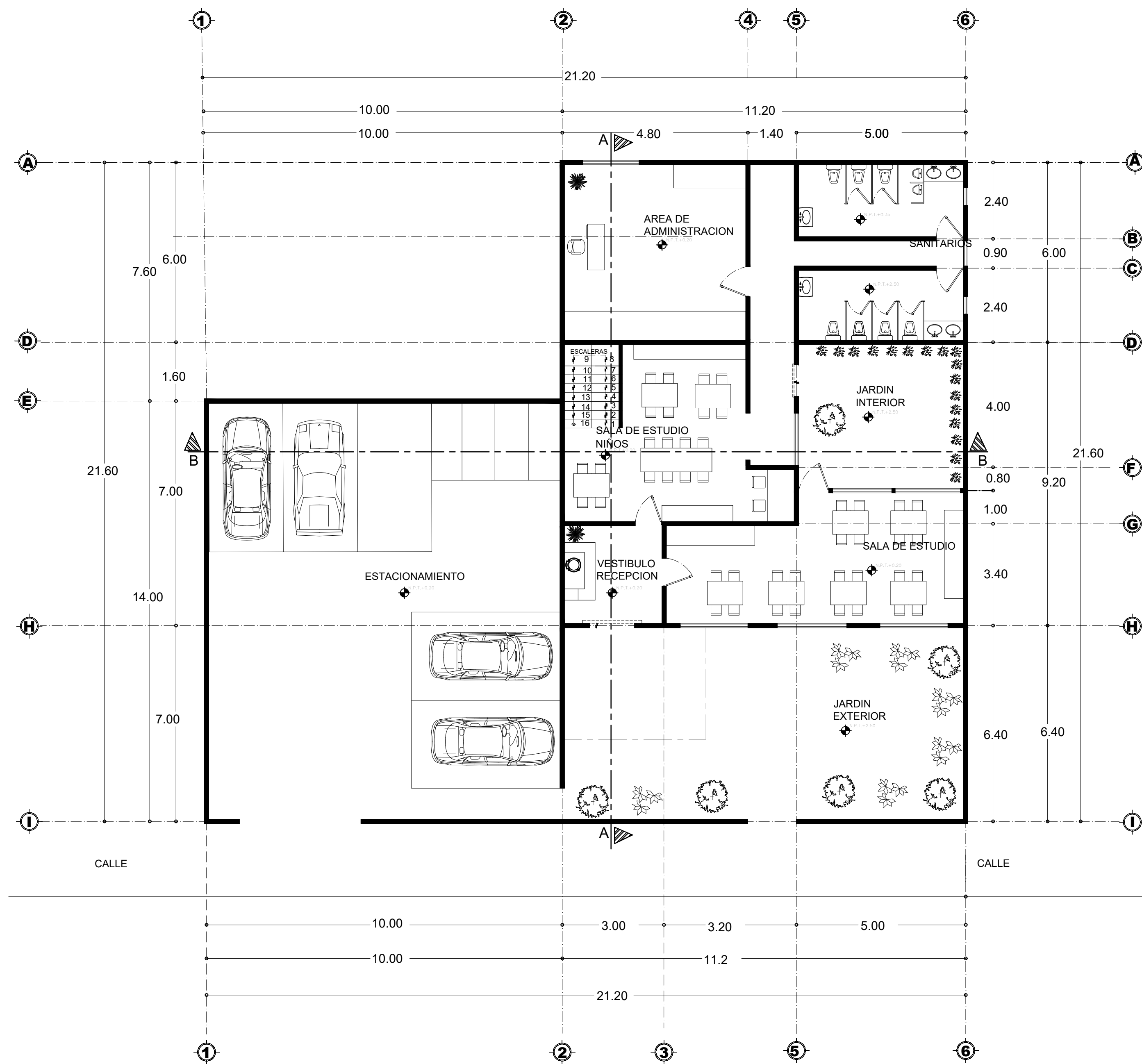
PLANTA ARQUITECTONICA BAJA ESC.....1.100
