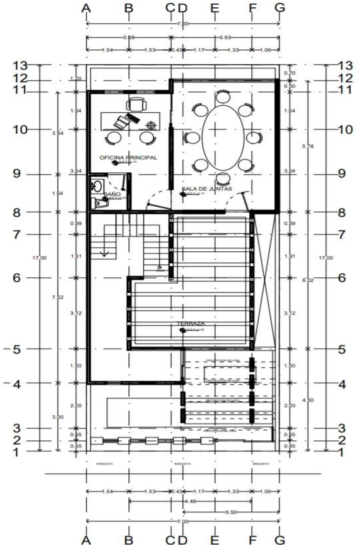
PLANTA ARQUITECTONICA ALTA
