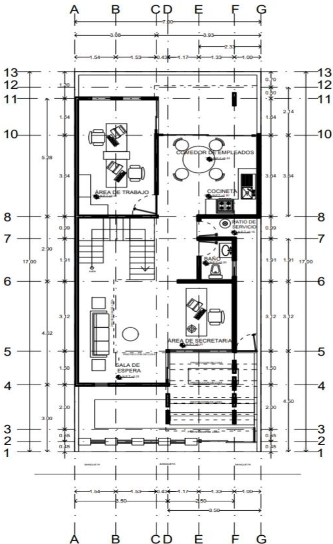
PLANTA ARQUITECTONICA BAJA
