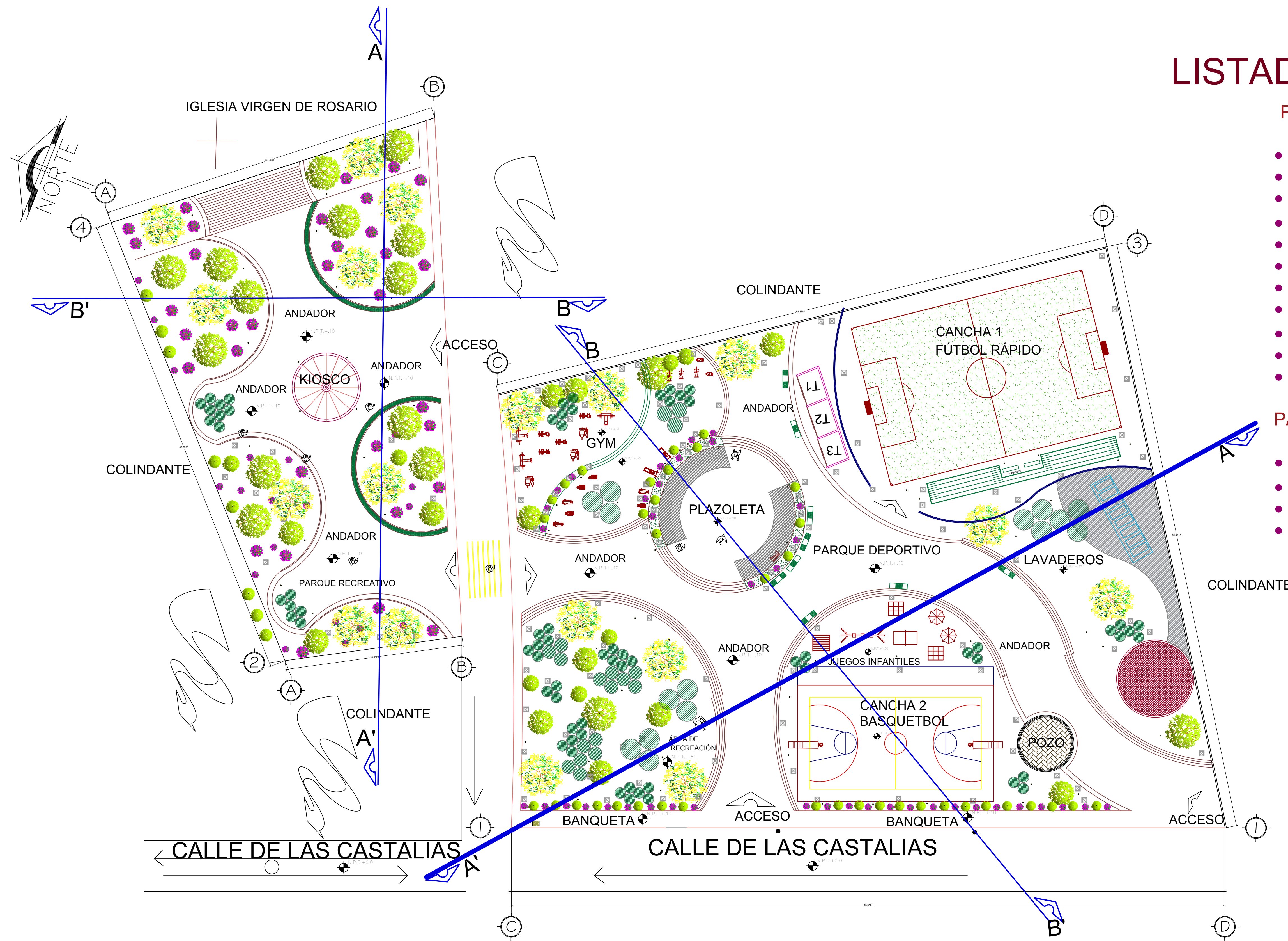
PLANTA ARQUITECTÓNICA ESC.....1:75
