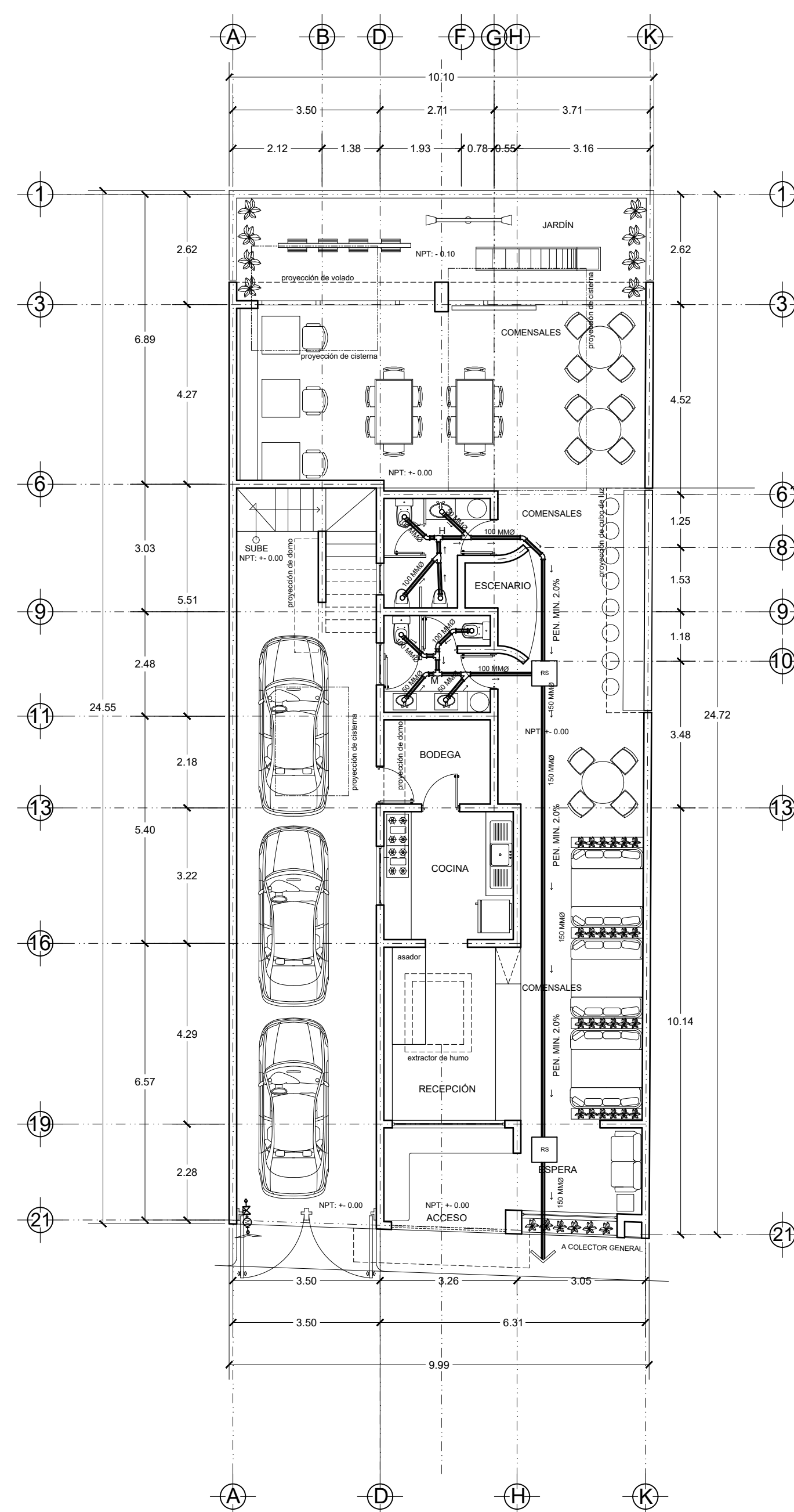
PLANTA ARQUITECTONICA BAJA INSTALACION SANITARIA
