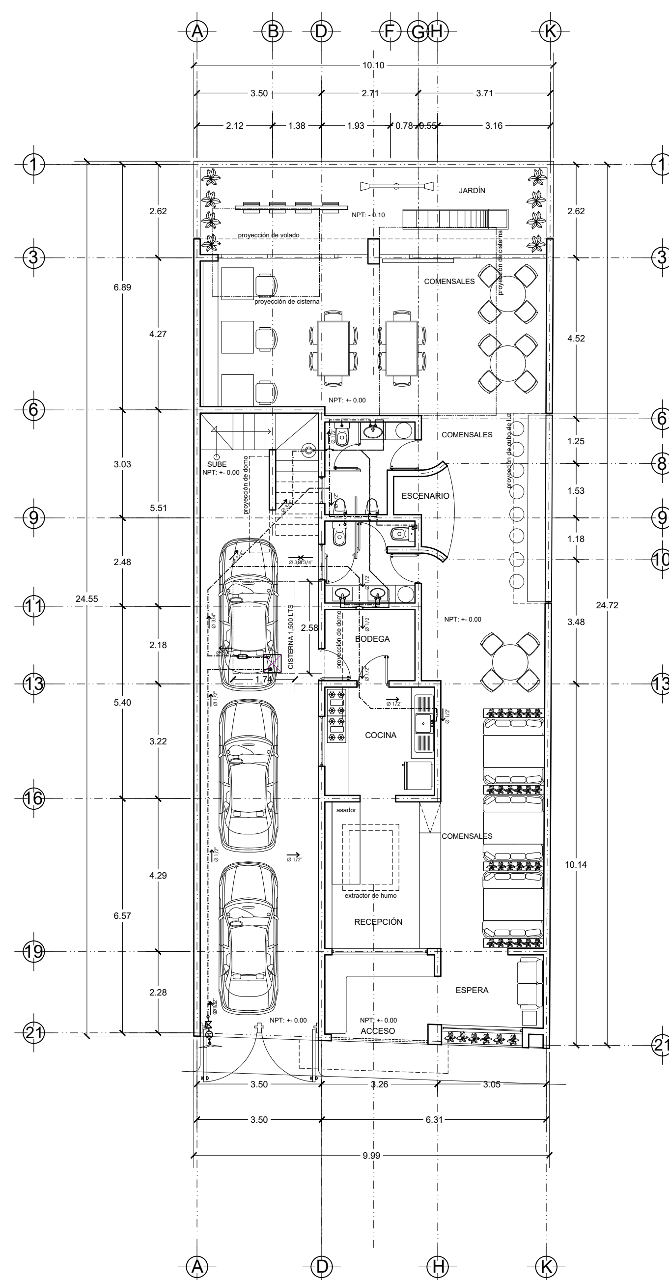
PLANTA ARQUITECTONICA BAJA INSTALACION HIDRAULICA
