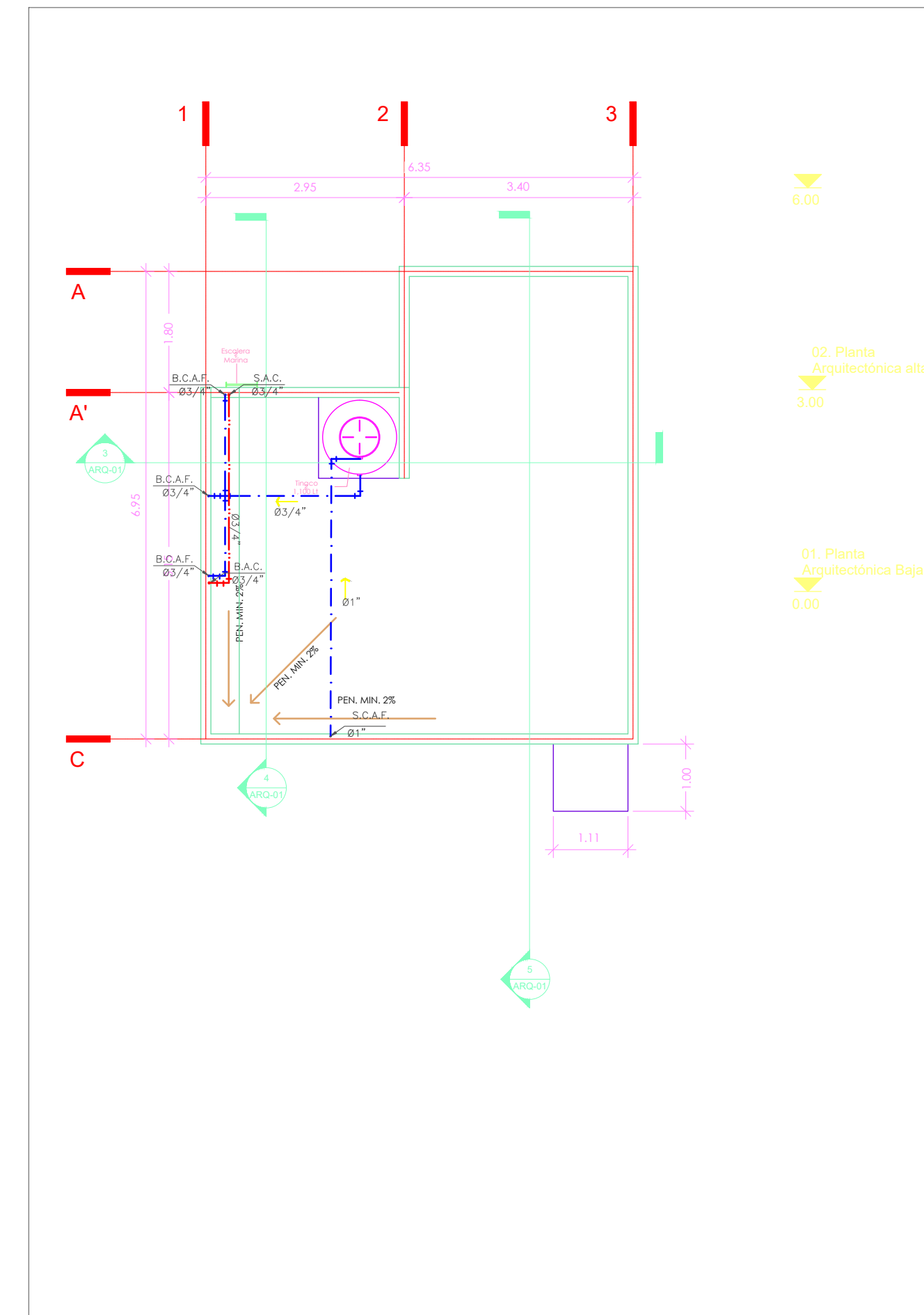
PLANTA HIDRAÚLICA AZOTEA ESC 1.75
