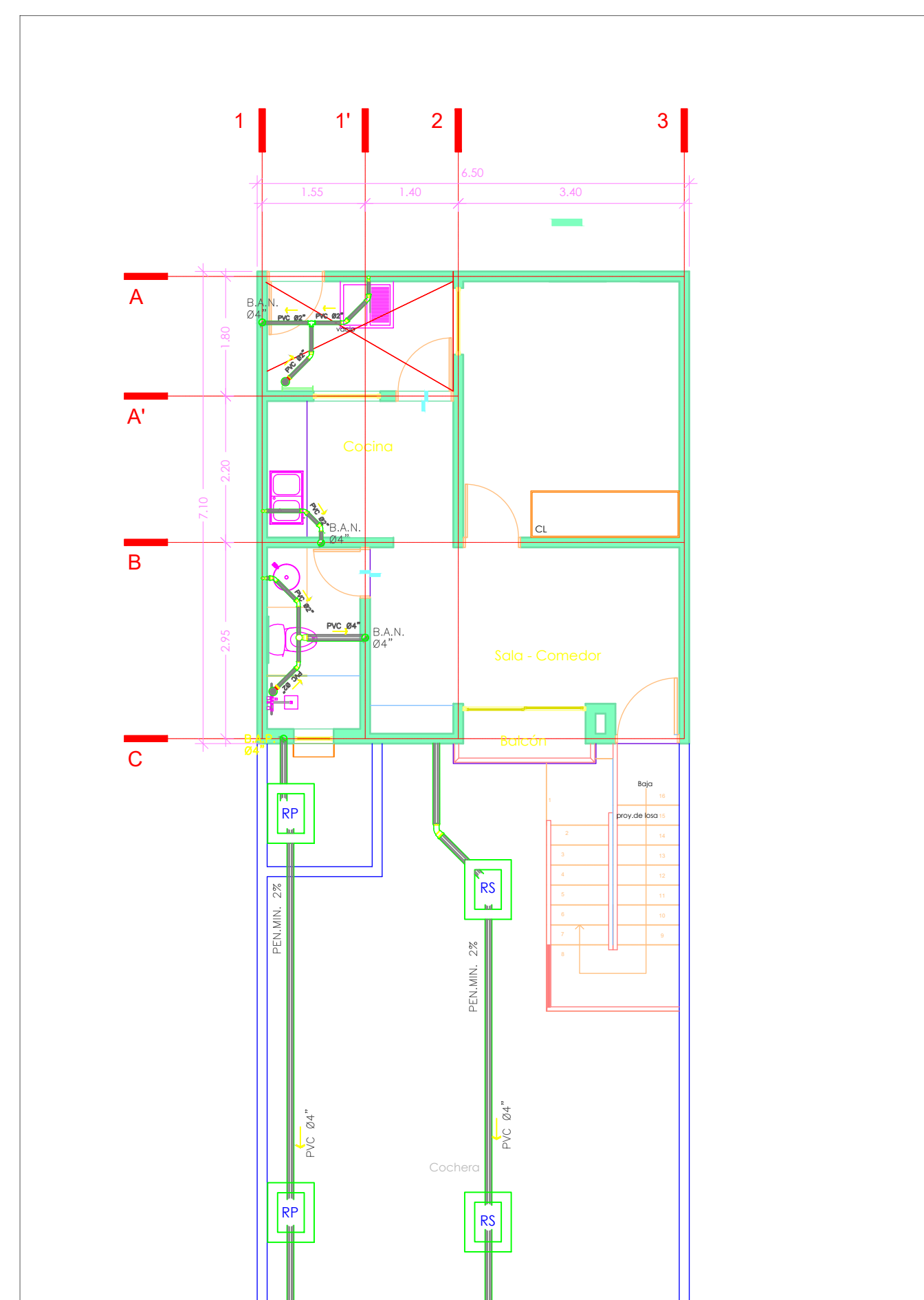
PLANTA SANITARIA Y BAJADAS PLUVIALES ESC 1.75
