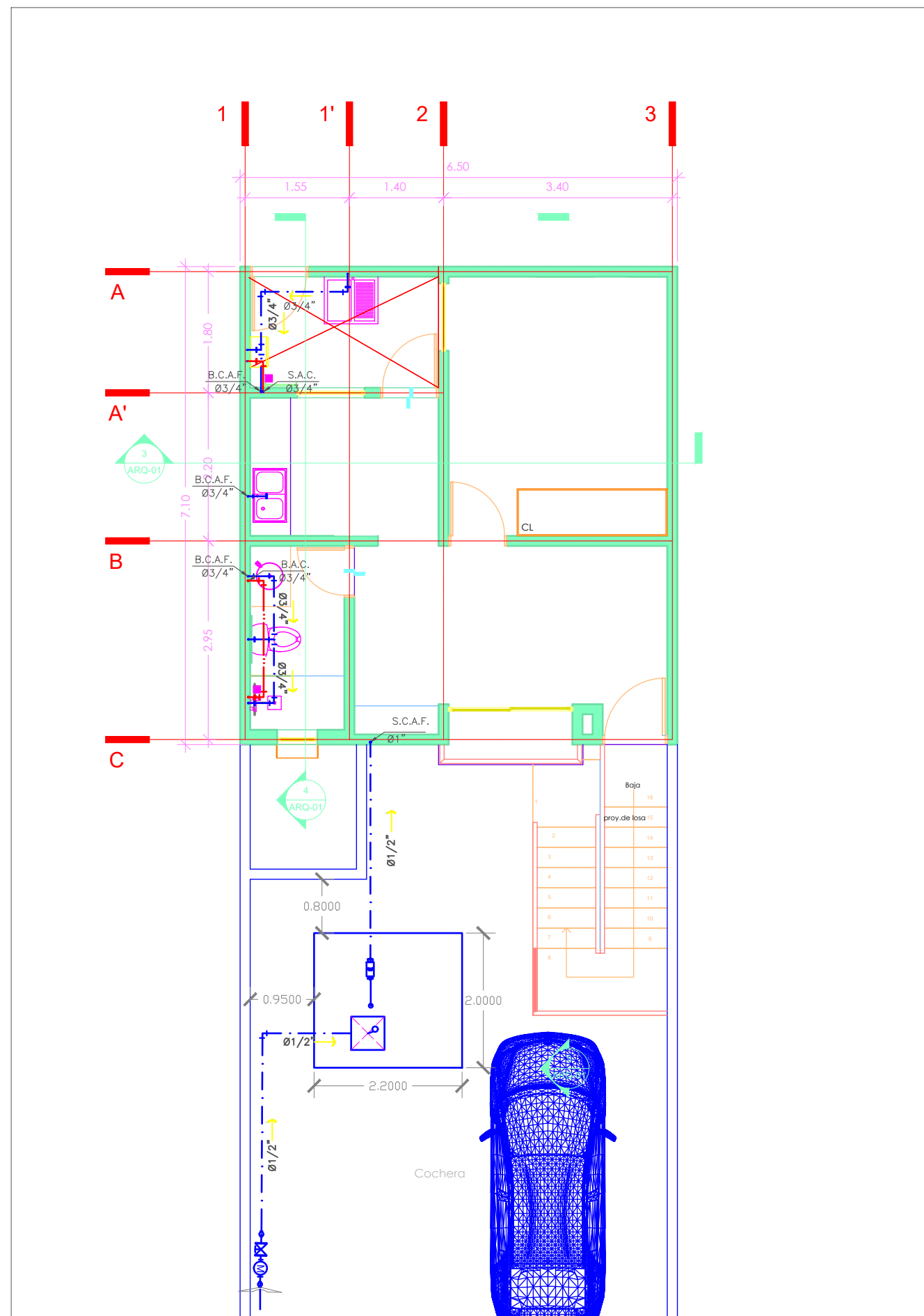
PLANTA HIDRAÚLICA ESC 1.75
