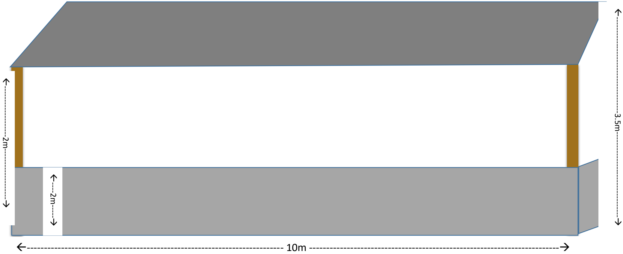
Vista lateral de instalaciones
