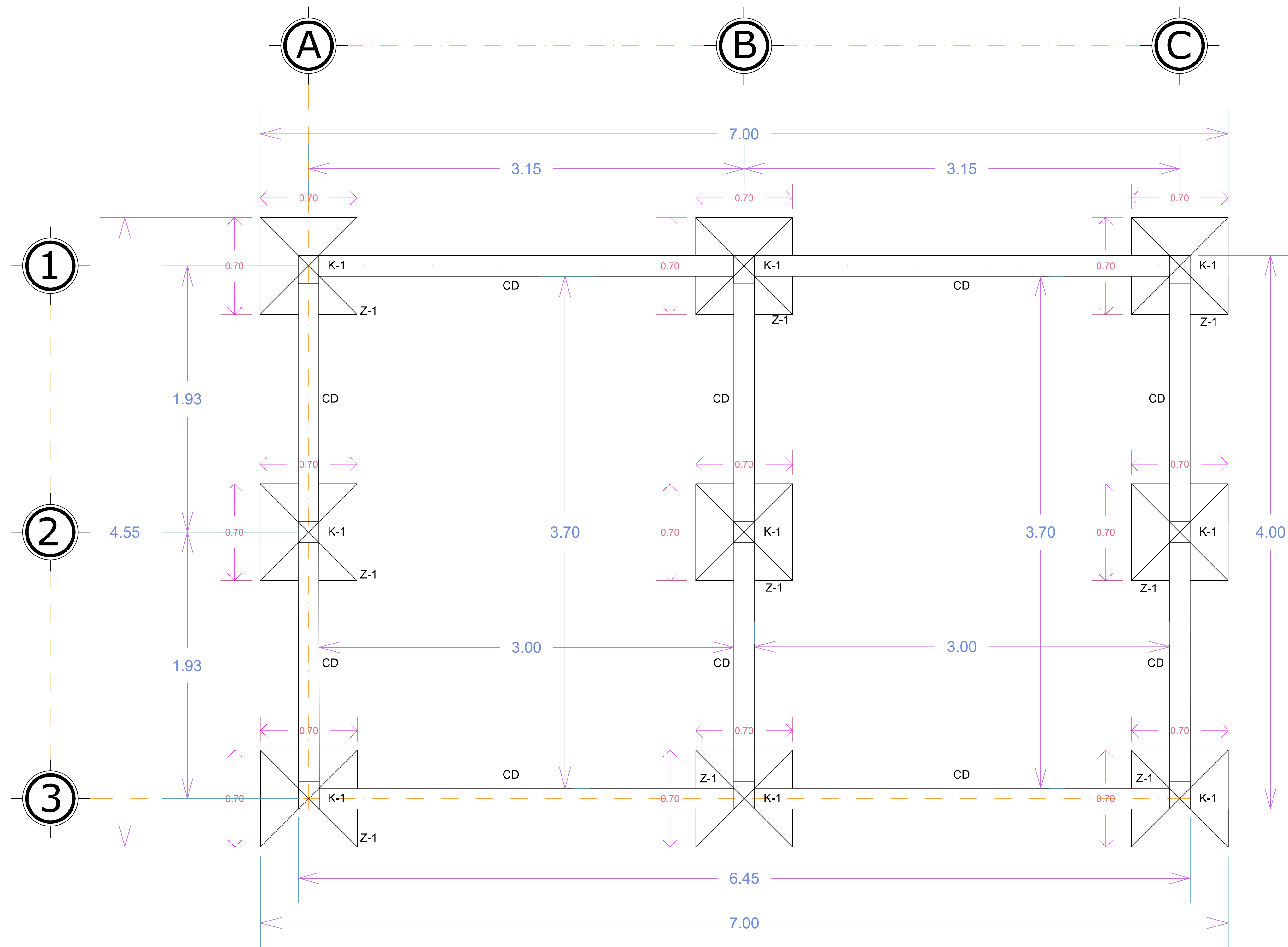
PLANTA DE CIMENTACION
