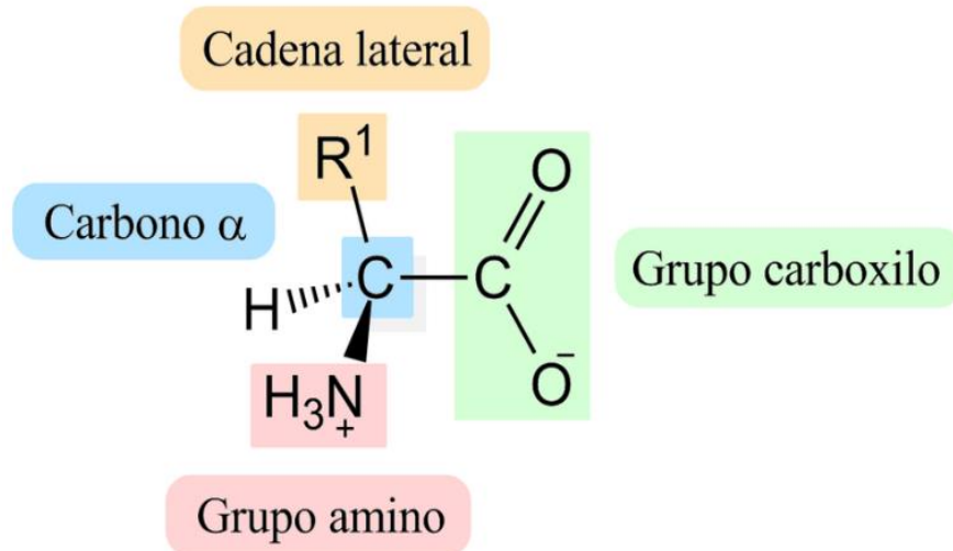
Estructura básica de un aminoácido
