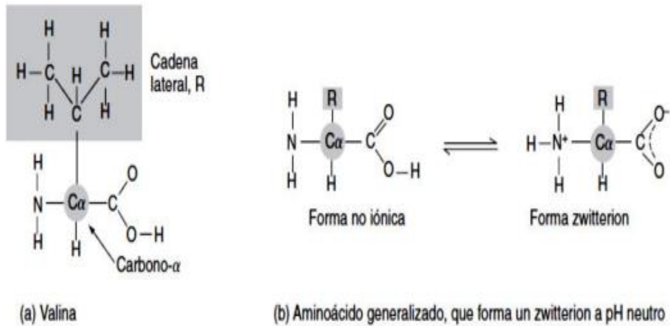
Figura 3.1 Estructura de los \alpha aminoácidos. 99
