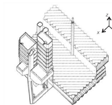
perspectiva planométrica
