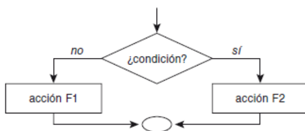
Figura 3.4. Bifurcación condicional.
