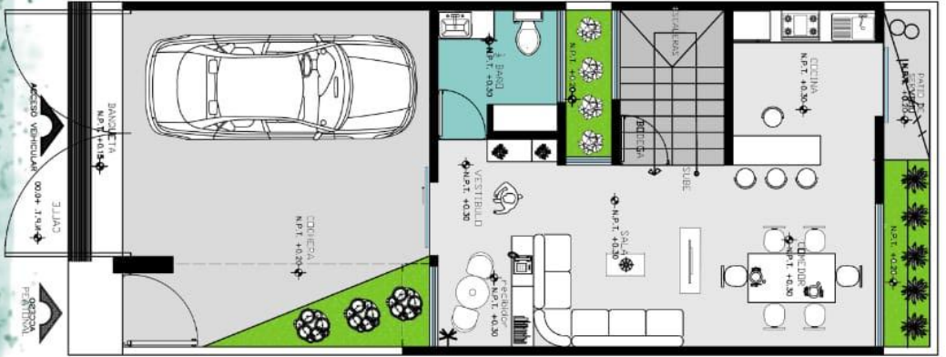
planta arquitectonica primer nivel
