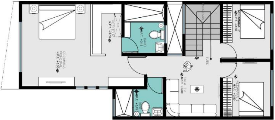
planta arquitectonica segundo nivel
