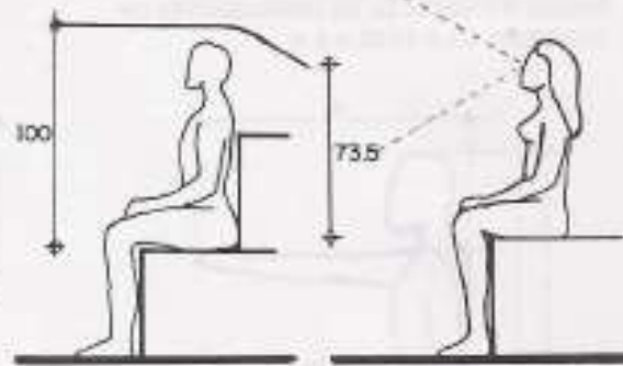
1.6.(B) Límite mínimo para la distancia de la superficie de un asiento al techo (más 10 cm. para sombreros o peinados).
