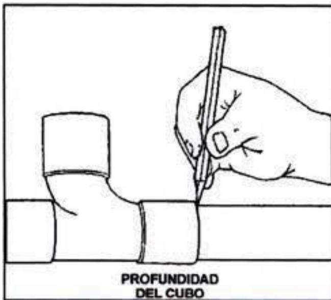
3.- MARCAR LA PROFUNDIDAD DEL TUBO EN EL CUBO O CONDUCTOR
