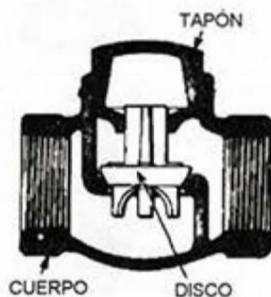
VÁLVULA DE SELLO ELEVADOR
