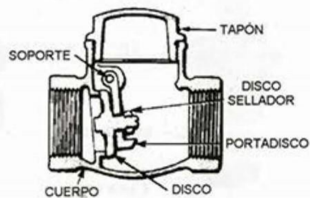
VÁLVULA DE SELLO OSCILANTE
