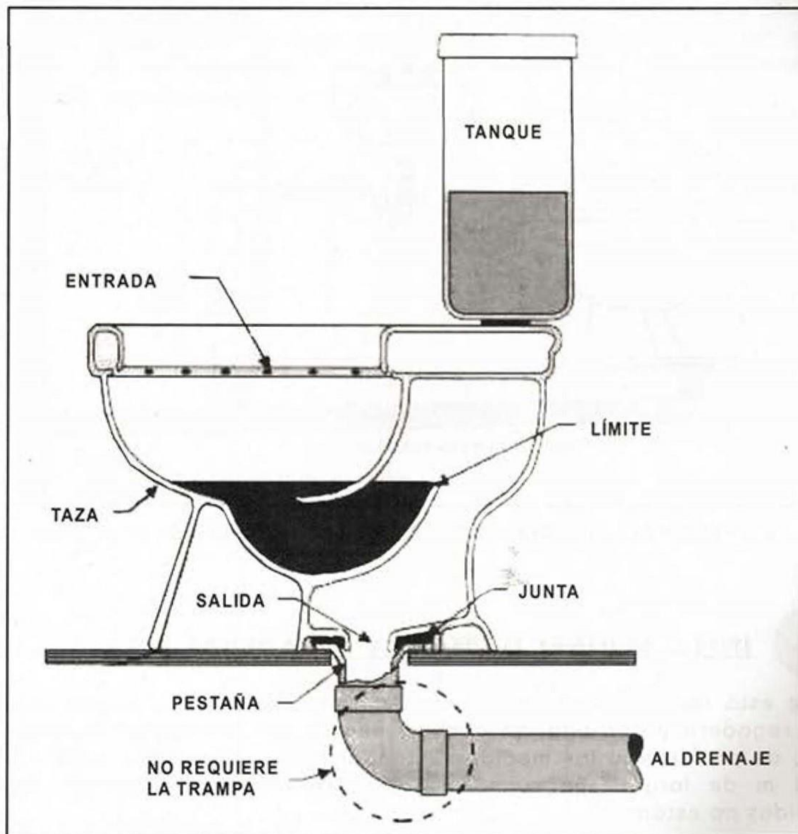
DETALLE DE LA SALIDA DE UN TOILET
