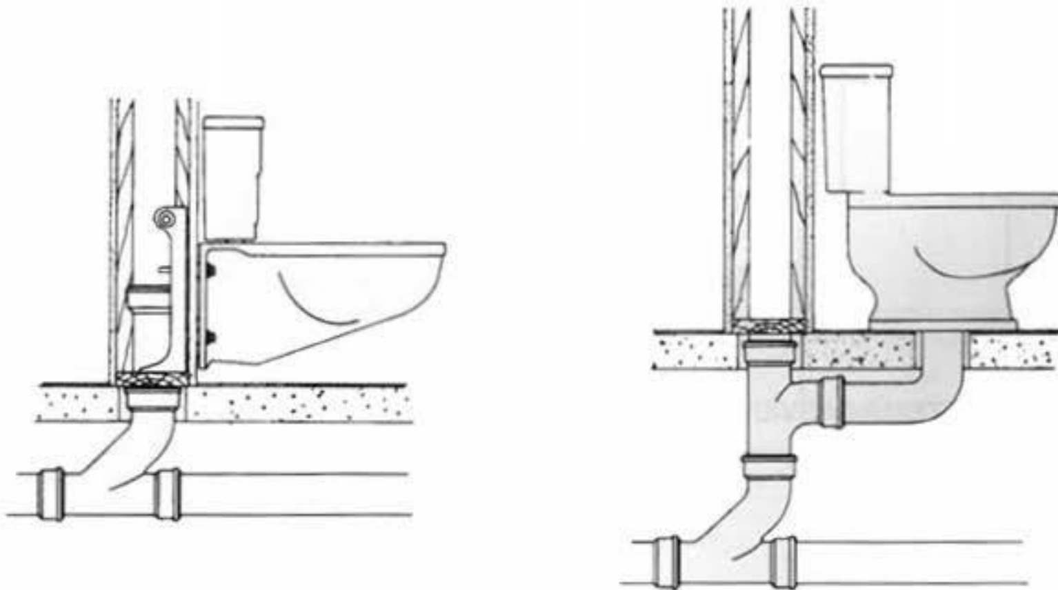
VARIANTES DE INSTALACIÓN DE W.C. (INODORO)
