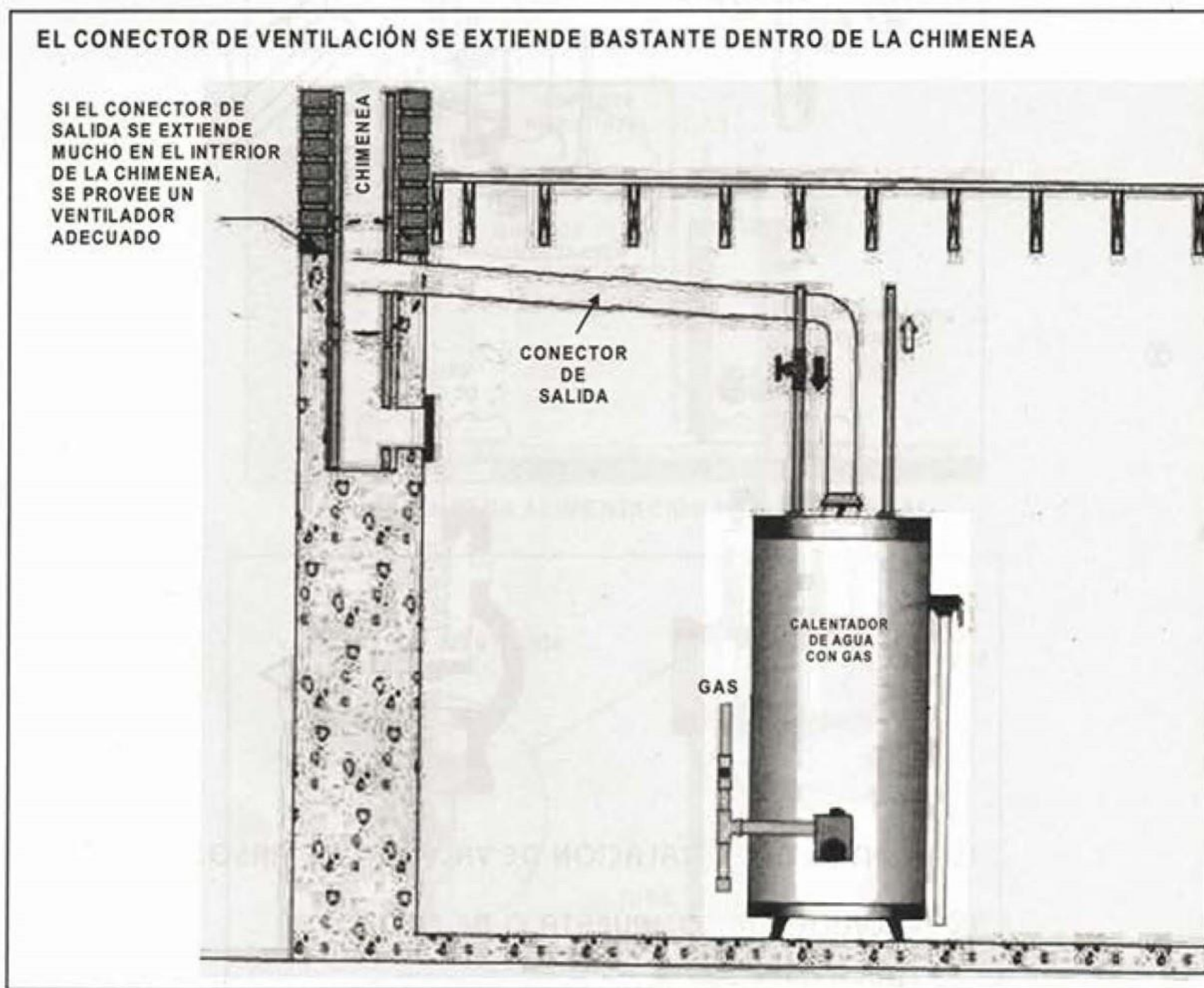
INSTALACIÓN DE CALENTADORES DE GAS
