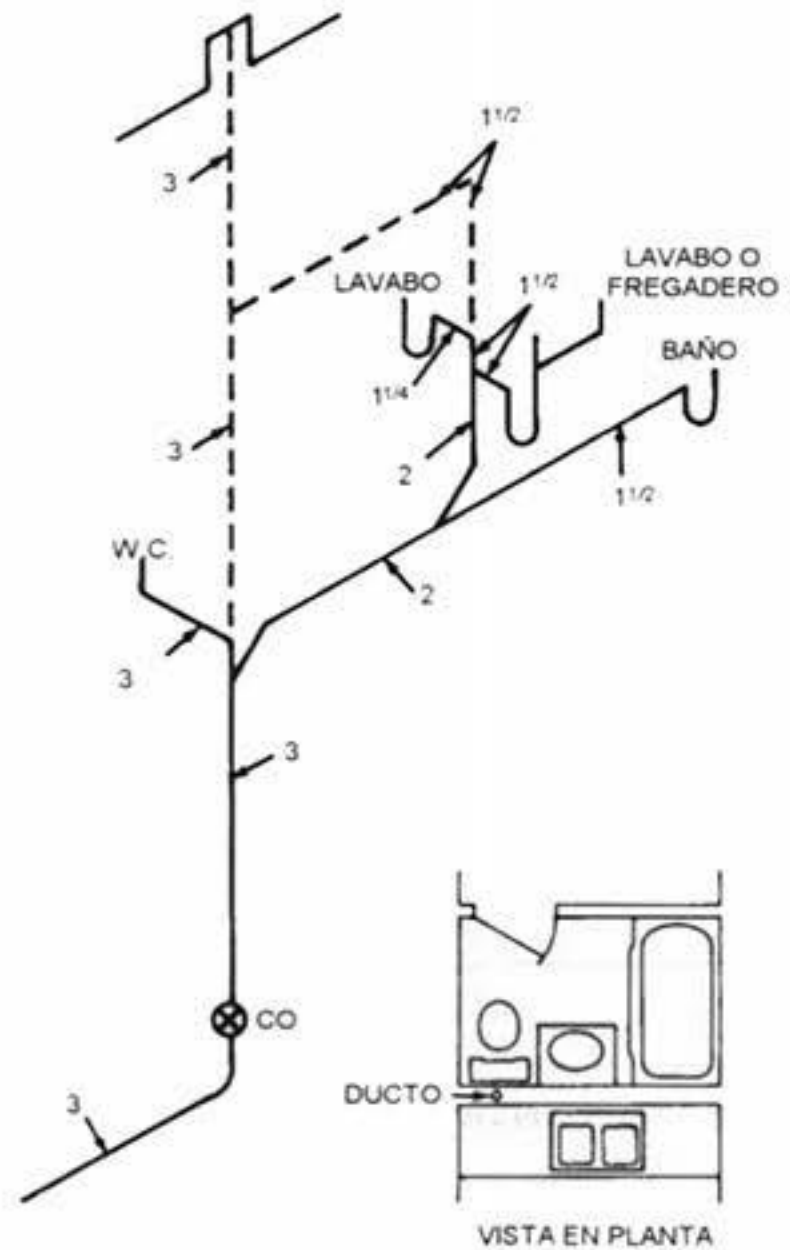
INSTALACIÓN DE VENTILACIÓN PARA BAÑO Y COCINA
