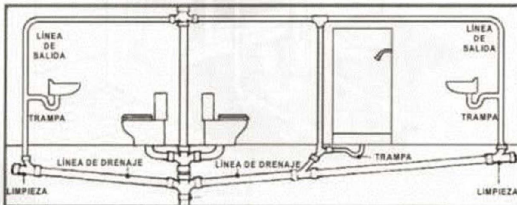
LÍNEA DE SALIDA DE TOILETS, REGADERA Y LAVABOS
