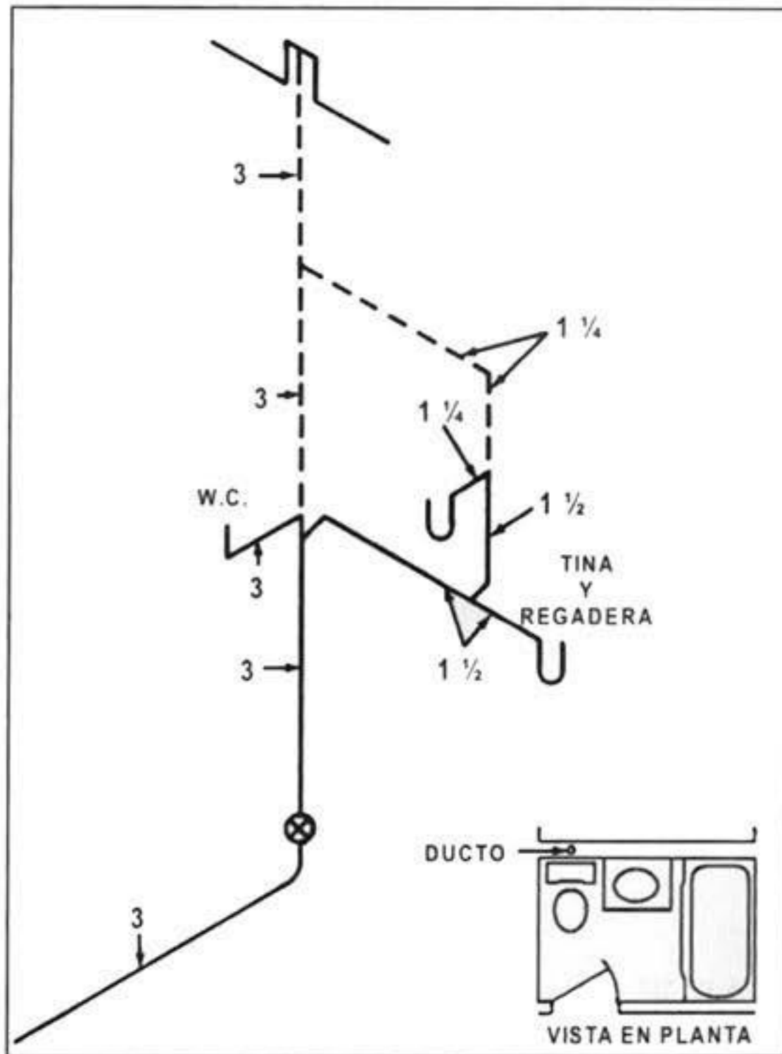
INSTALACIÓN DE VENTILACIÓN PARA UN BAÑO Y DIMENSIONES RECOMENDADAS PARA TUBOS
