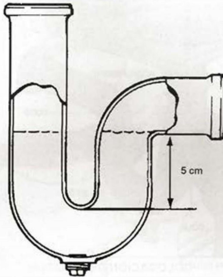
TRAMPA DE SIFÓN
