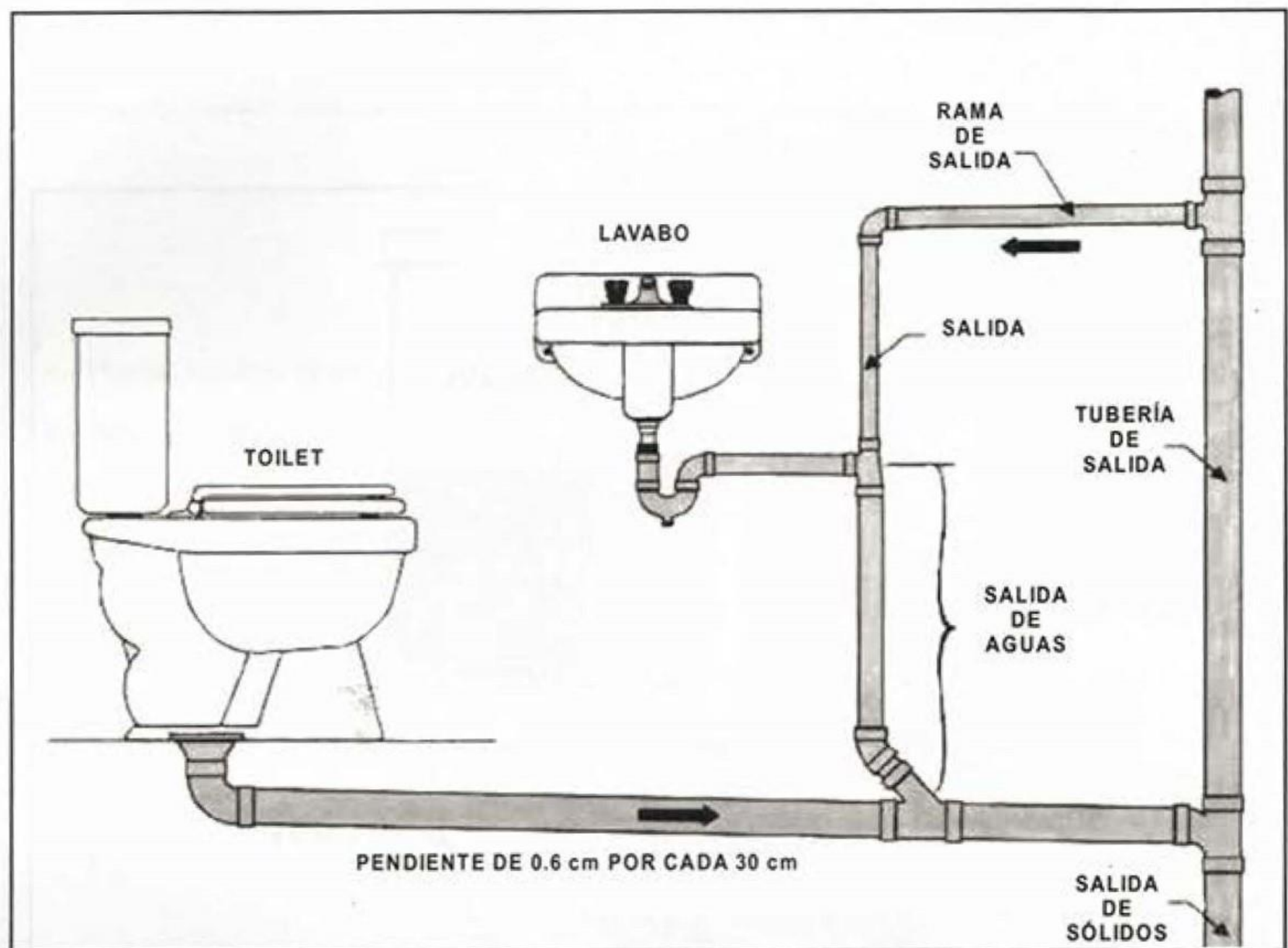
ELEMENTOS DE LA INSTALACIÓN DEL TOILET (INODORO) Y LAVABO EN UN BAÑO
