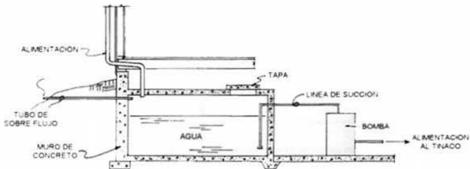
CONSTRUCCIÓN DE UNA CISTERNA
