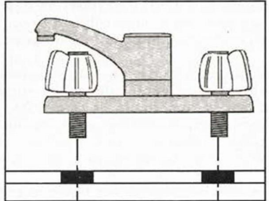
2.- INSERTAR LAS CONEXIONES DEL GRIFO EN LOS AGUJEROS, SE DEBE REFERIR A LAS INSTRUCCIONES PARTICULARES.
