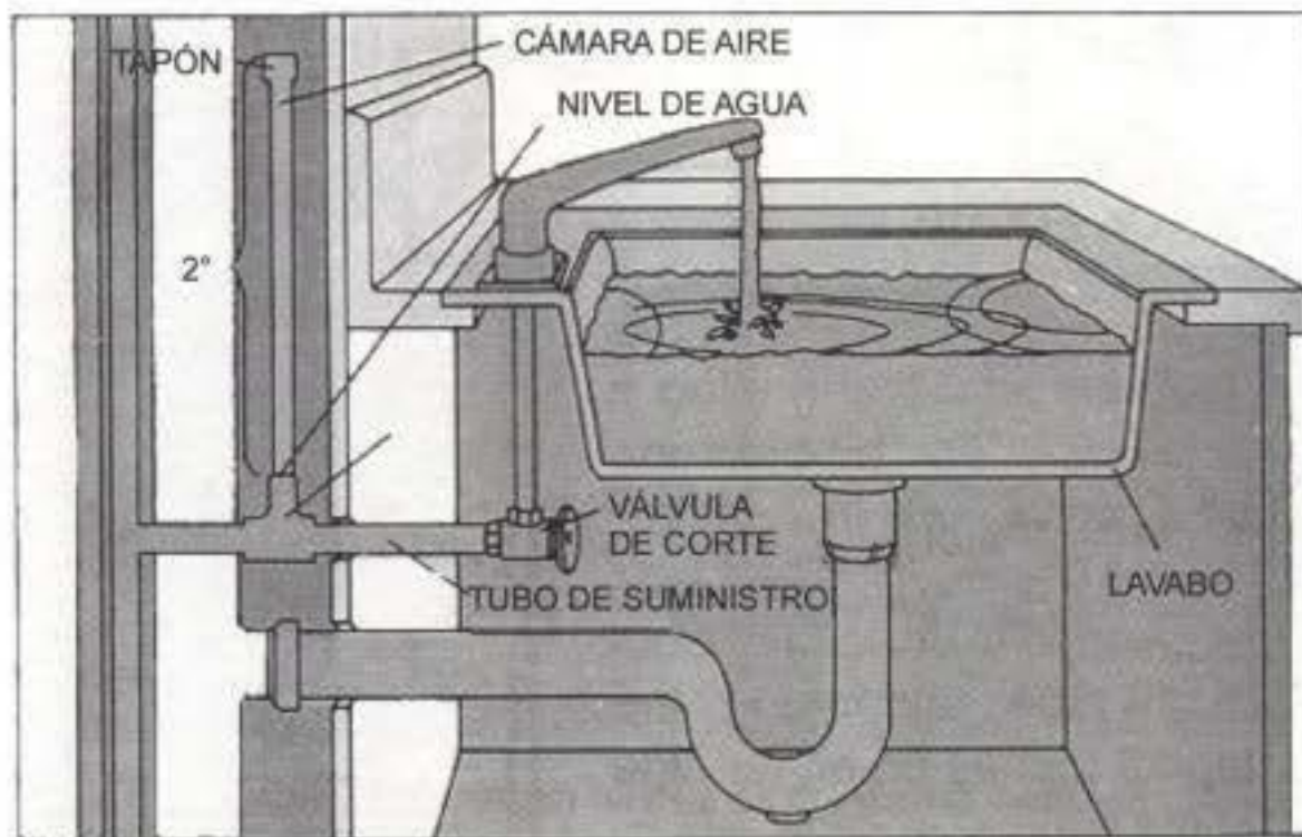
DETALLE DE INSTALACIÓN DEL LAVABO
