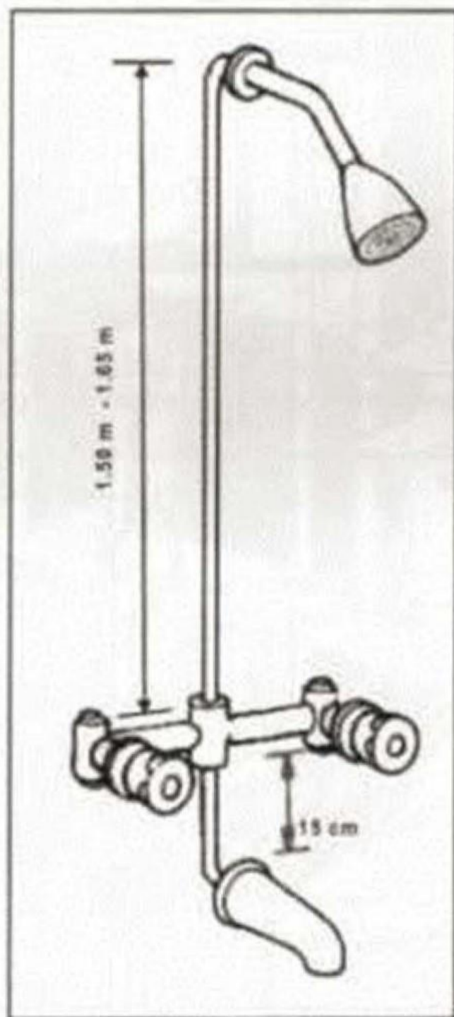
DETALLE DE INSTALACIÓN DE REGADERA Y LLAVES PARA TINA
