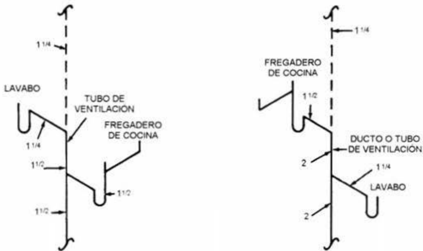
TUBO O DUCTO DE VENTILACIÓN CON SALIDA DE LAVABO Y FREGADERO AL MISMO TUBO
