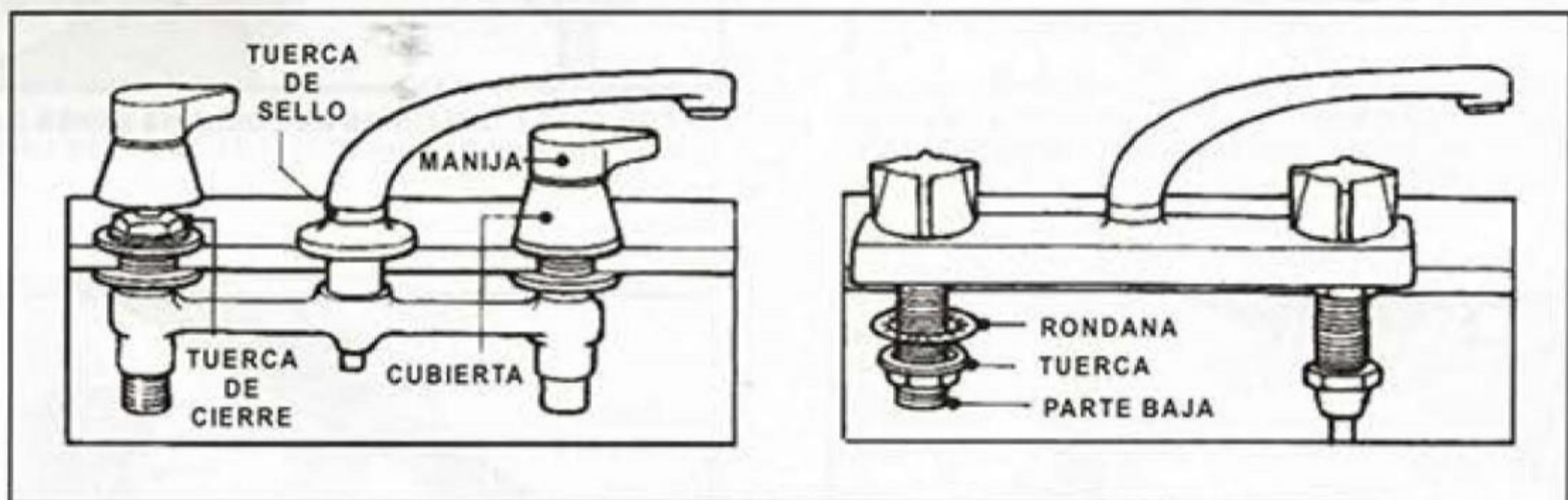
DETALLE DE MONTAJE DE UNA LLAVE O GRIFO
