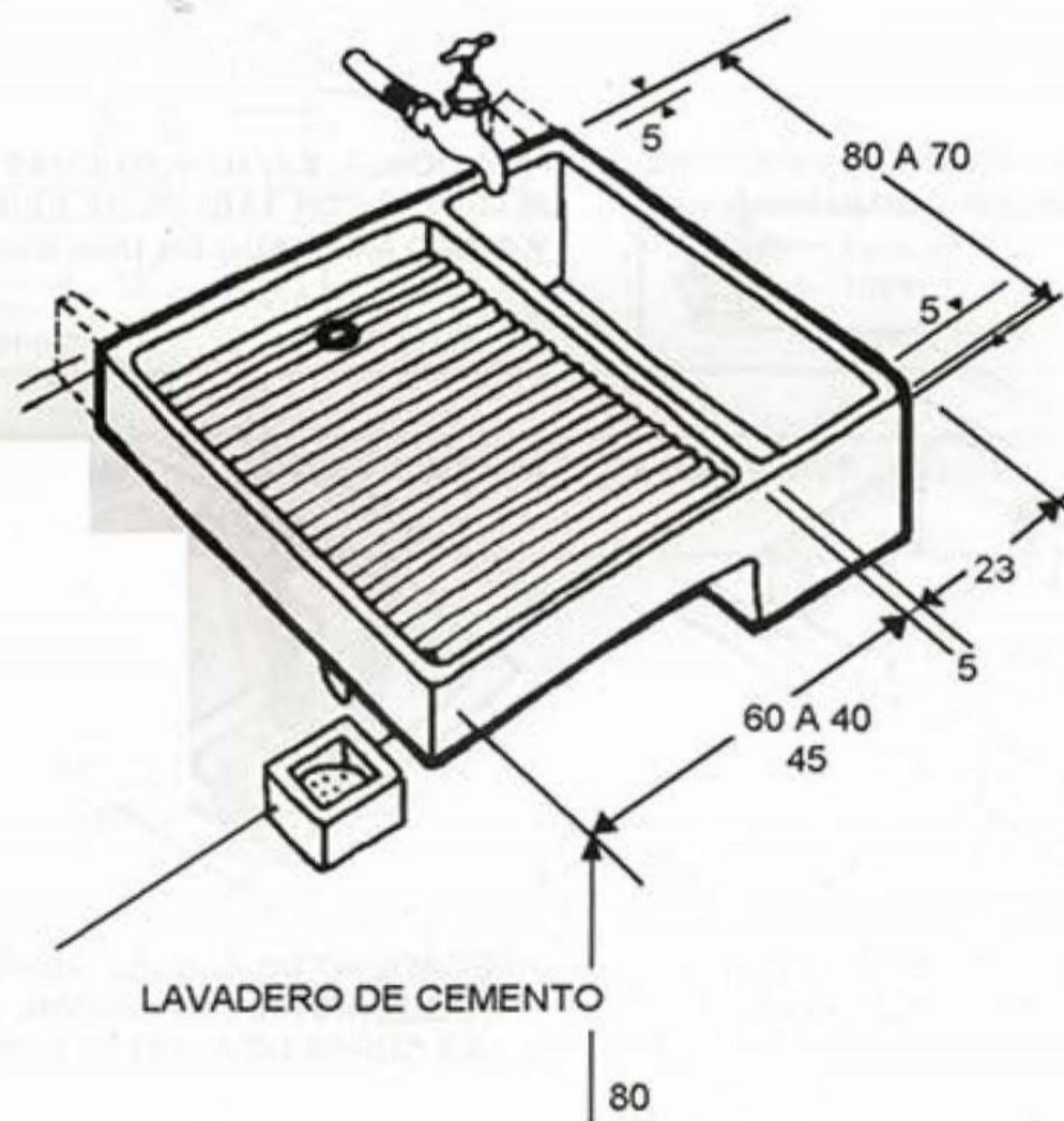
ALGUNOS TIPOS DE LAVADEROS Y FREGADEROS PREFABRICADOS
