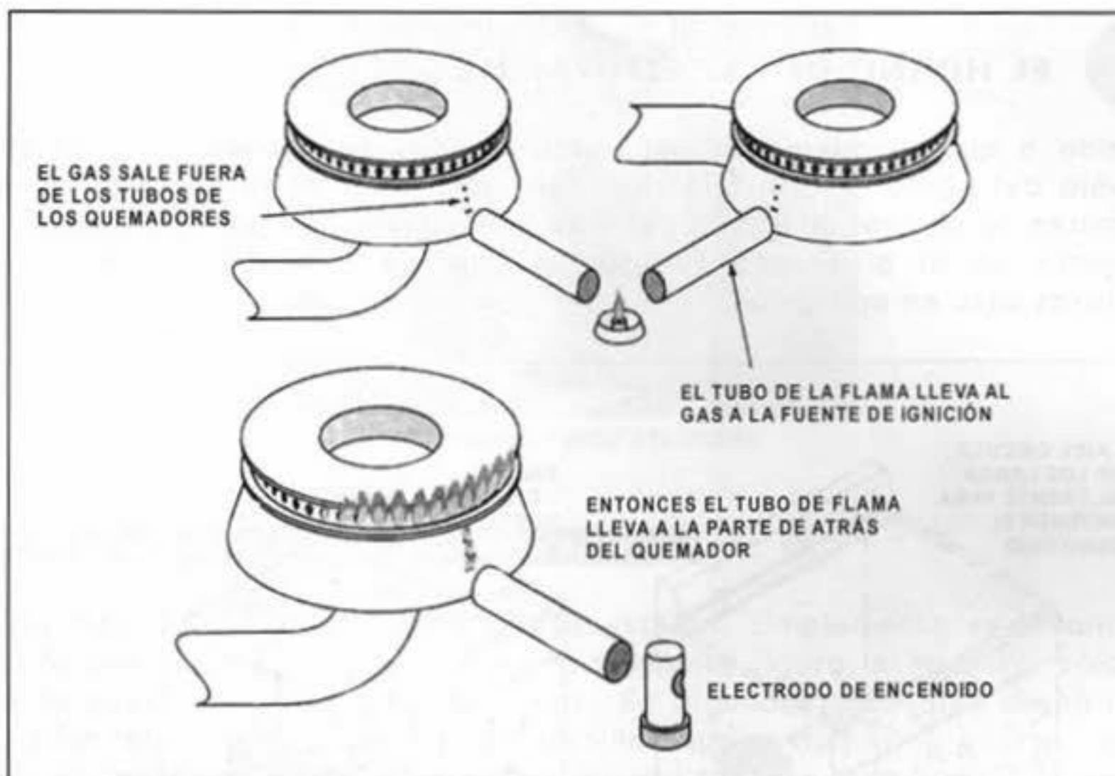
ENCENDIDO DEL QUEMADOR DE GAS
