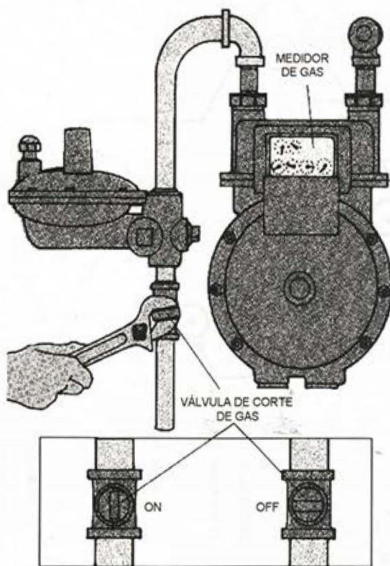
VÁLVULA DE GAS Y MEDIDOR PARA CONEXIÓN A SUMINISTRO DE GAS NATURAL
