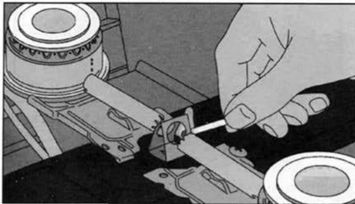
REENCENDIDO DEL PILOTO
