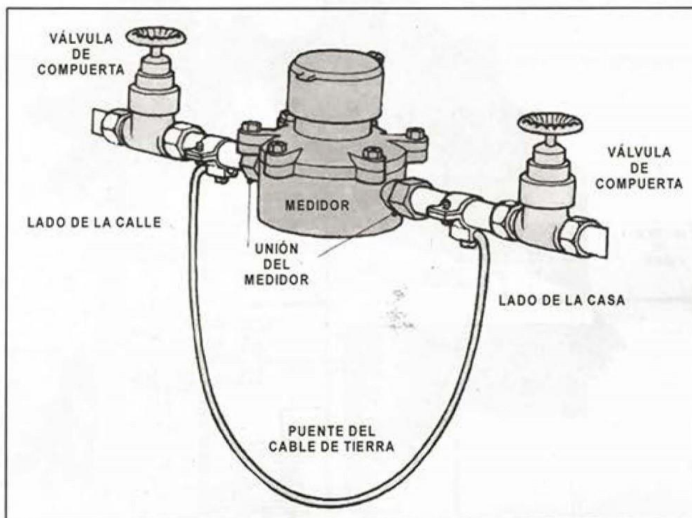
INSTALACIÓN DEL MEDIDOR DE AGUA
