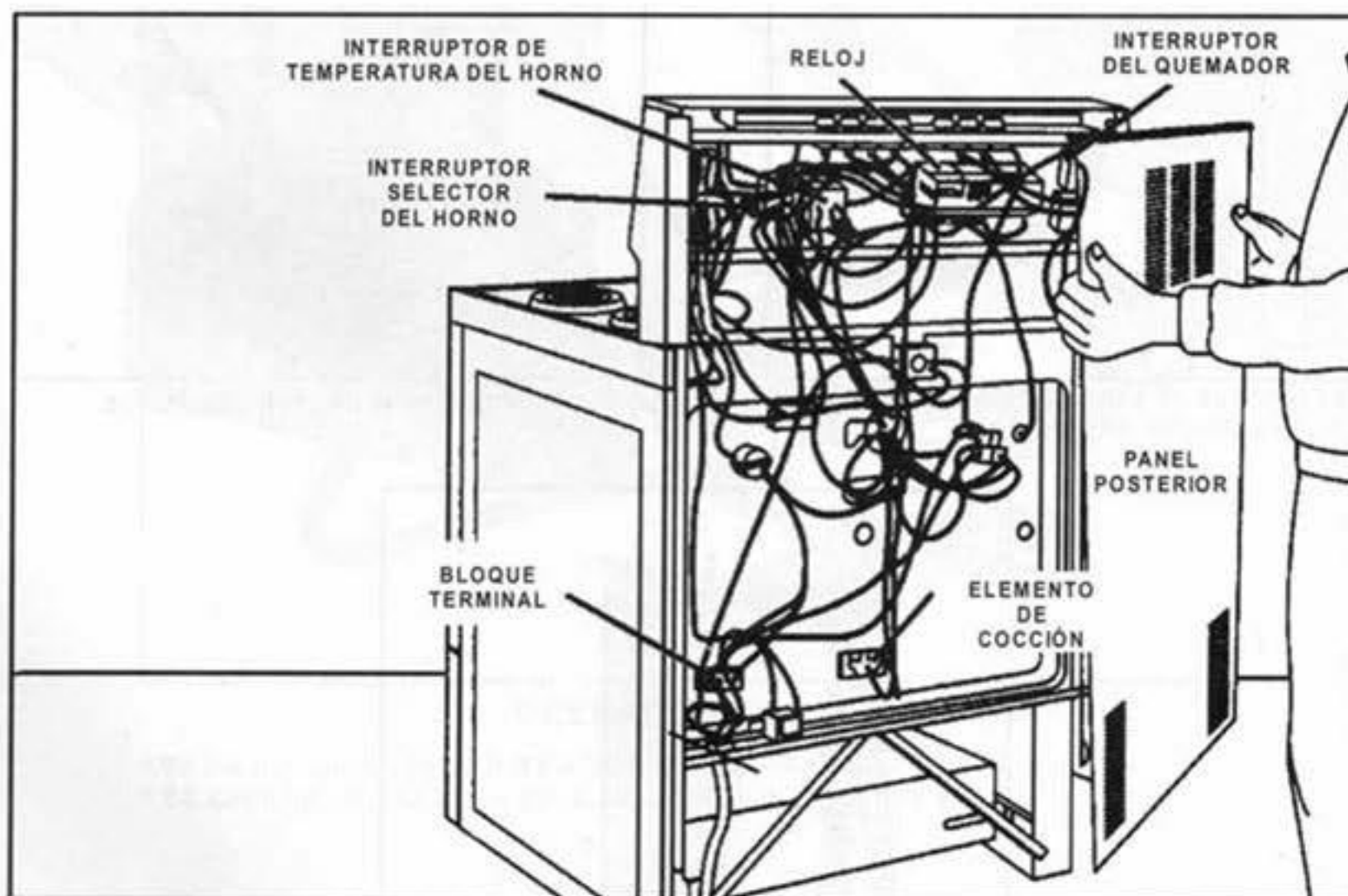
REMOCIÓN DE TORNILLOS DEL PANEL POSTERIOR PARA TENER ACCESO A LOS COMPONENTES
