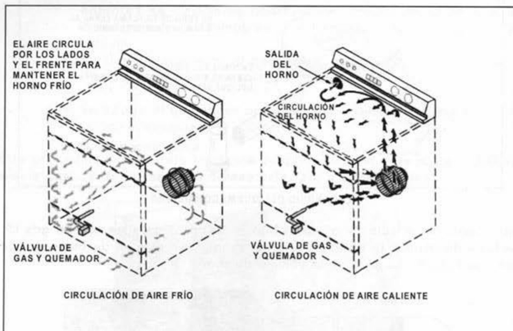
CIRCULACIÓN TÍPICA DEL AIRE POR CONVECCIÓN EN UN HORNO DE ESTUFA
