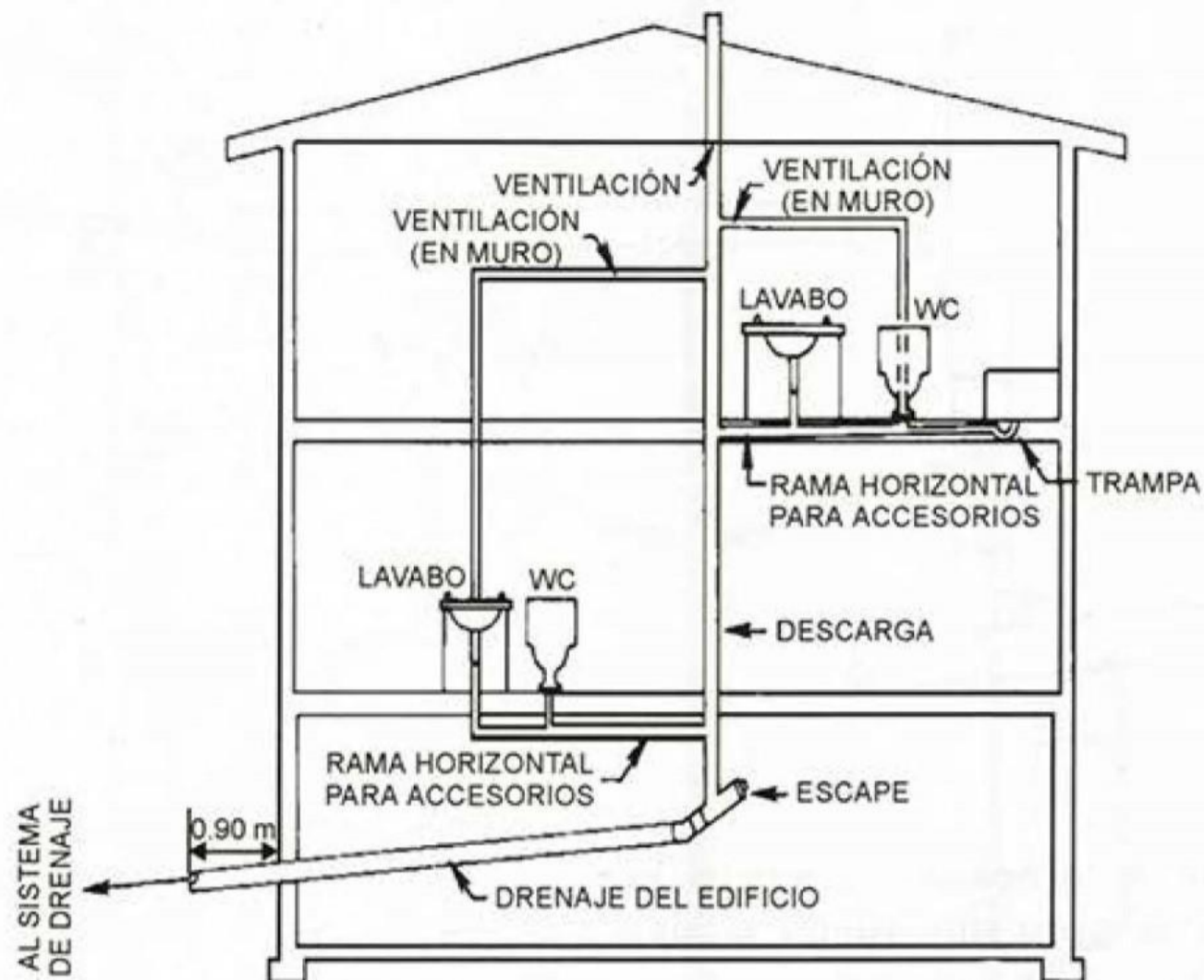
SISTEMA DE DRENAJE EN DEPARTAMENTOS
