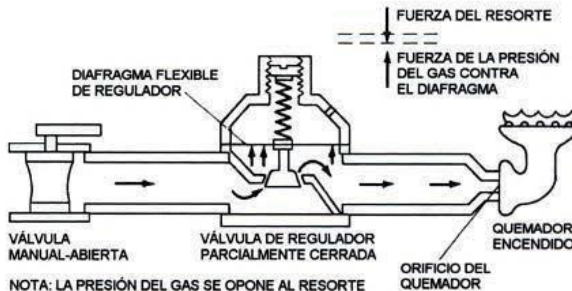
REGULADOR DE PRESIÓN DEL QUEMADOR DE GAS
