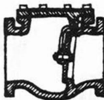
VÁLVULA CHECK OSCILANTE
