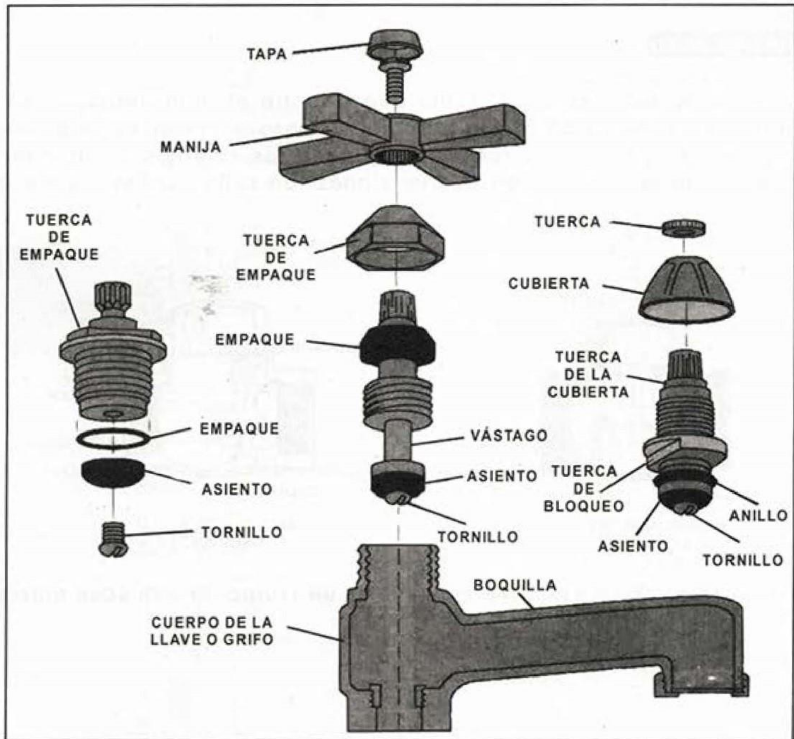
PARTES DE UNA LLAVE O GRIFO TIPO COMPRESIÓN
