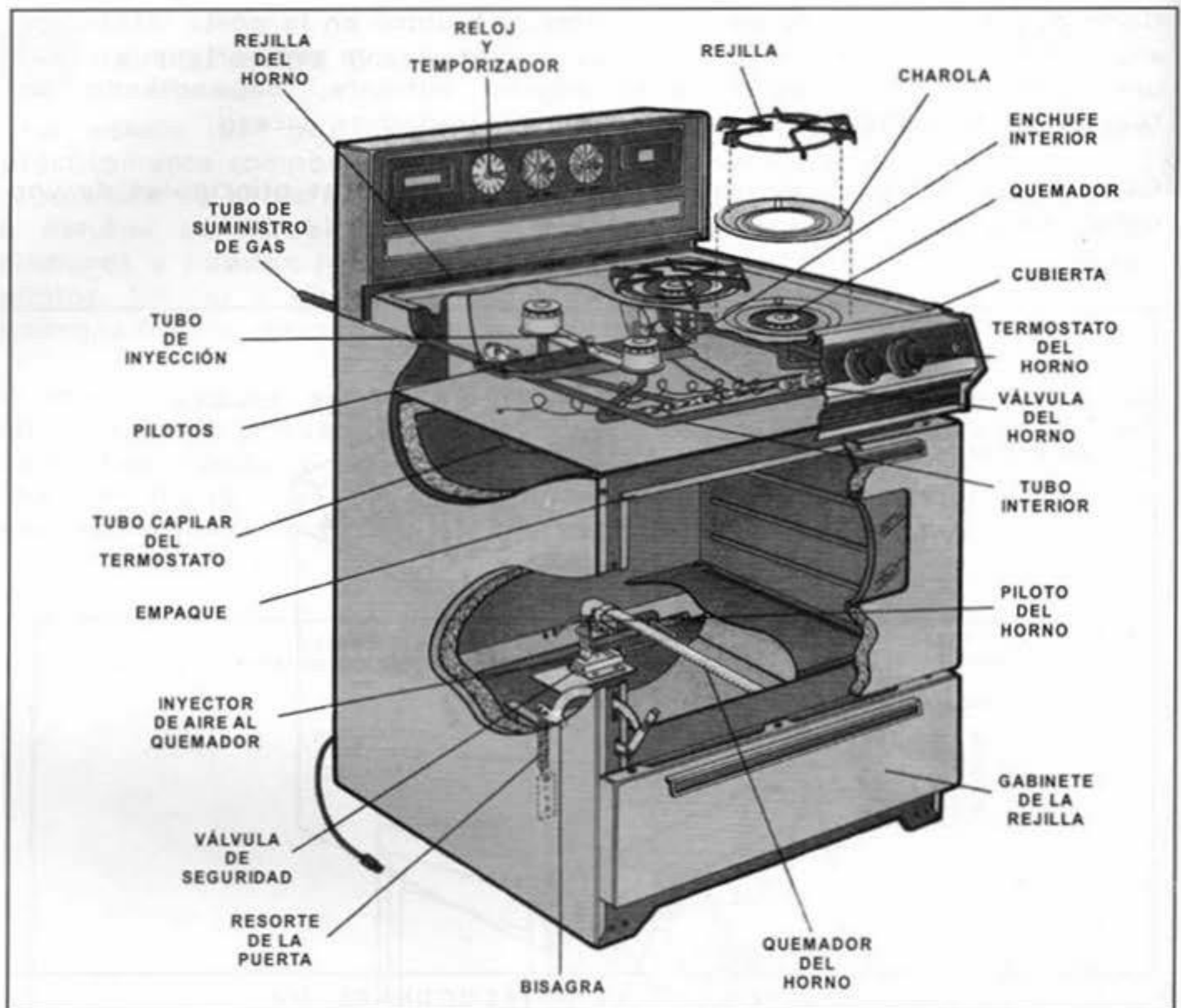
PARTES PRINCIPALES DE UNA ESTUFA DE GAS
