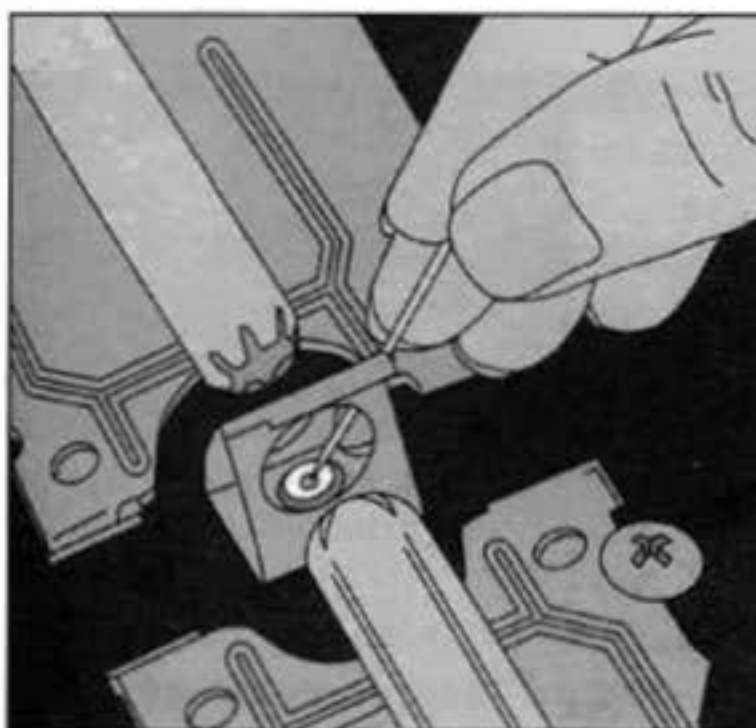
LIMPIEZA DEL PILOTO
