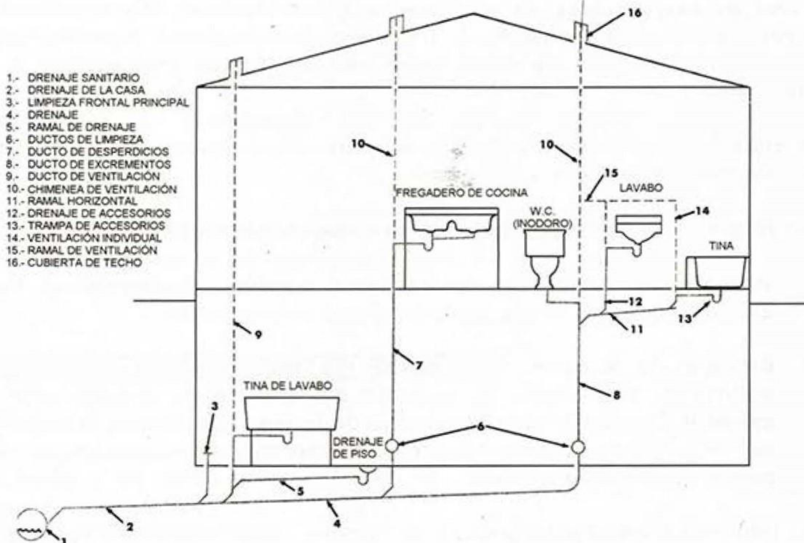
SISTEMAS DE DRENAJE SANITARIO Y DE VENTILACIÓN EN UNA CONSTRUCCIÓN
