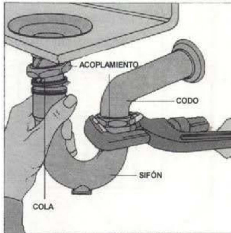
COLOCACIÓN DE UN SIFÓN
