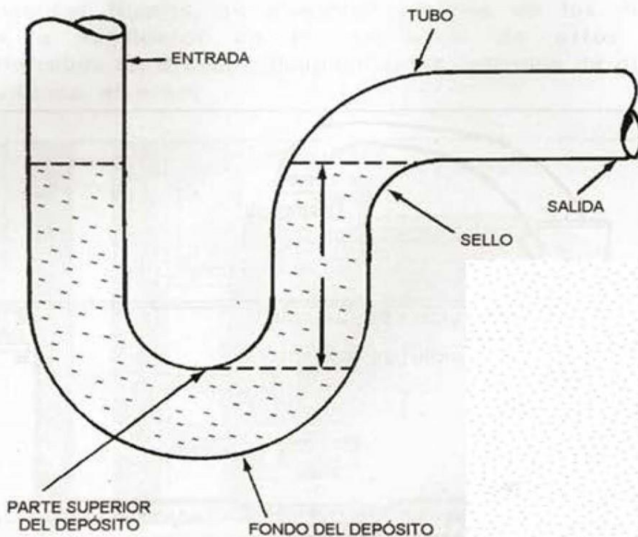
TRAMPA DE SIFÓN TIPO P
