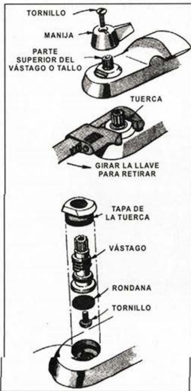
PARTES DE UNA LLAVE O GRIFO PARA BAÑO
