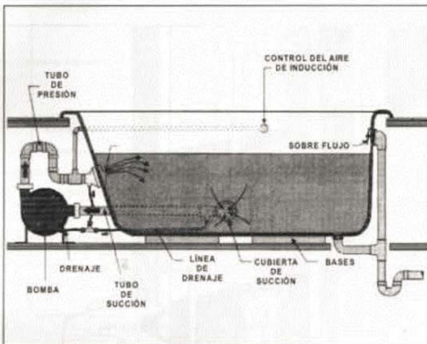
INSTALACIÓN DE UNA TINA DE BAÑO
