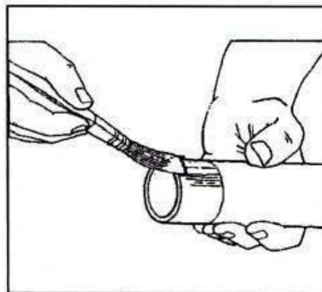
5.- APLICAR CEMENTO TANTO AL TUBO COMO AL HERRAJE
