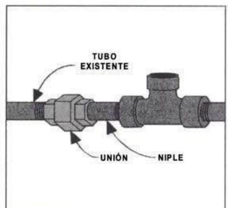
USO DE UNIONES ROSCADAS
