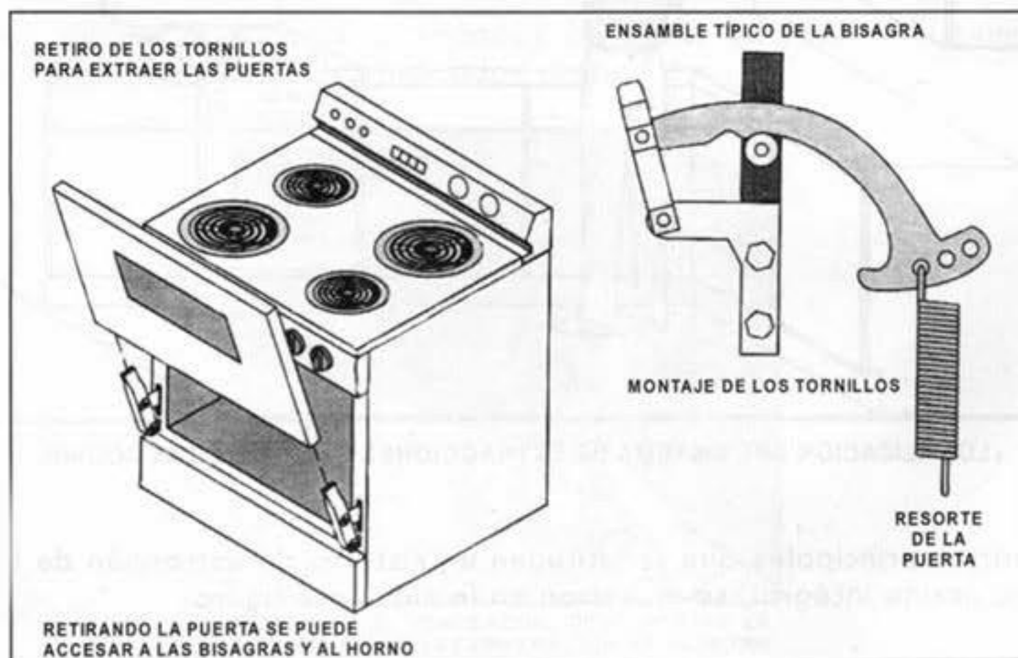
RETIRO DE LAS PUERTAS
