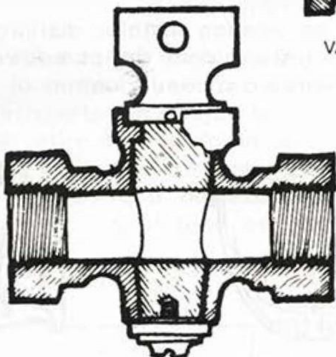
VÁLVULA O LLAVE DE CUADRO
