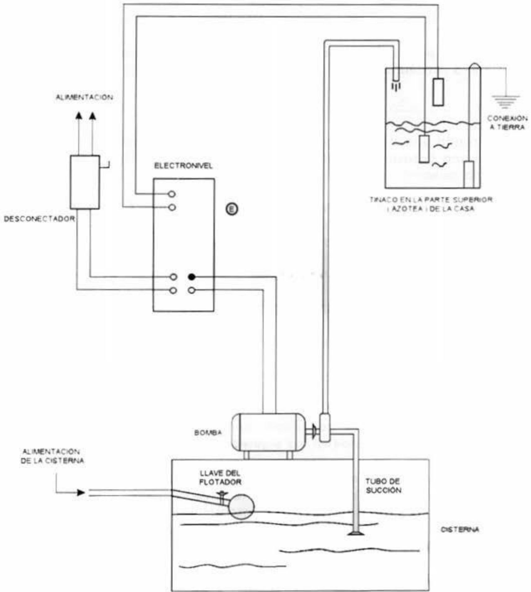
INSTALACION DE CISTERNA Y TINACO CON SISTEMA DE CONTROL POR ELECTRONIVEL
