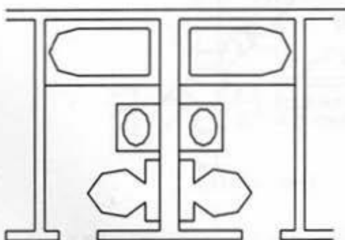
INSTALACIÓN DE PLOMERÍA ESPALDA A ESPALDA (BAÑO CON BAÑO)
