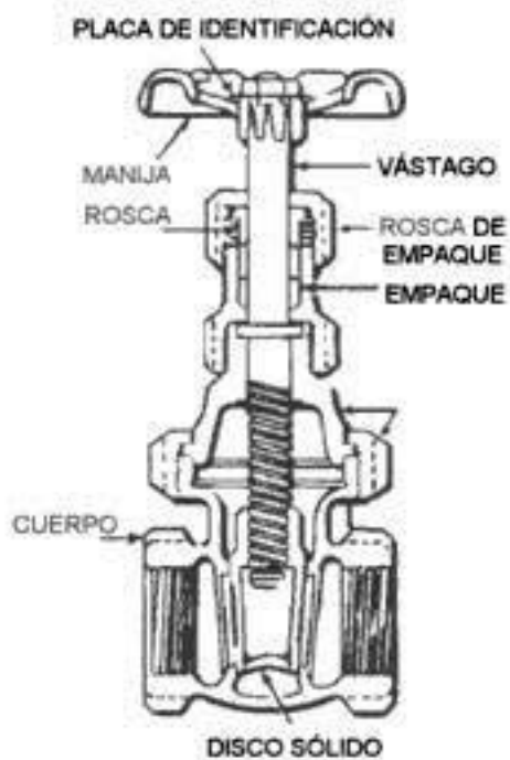
VÁLVULA DE COMPUERTA CON VÁSTAGO NO ELEVADOR
