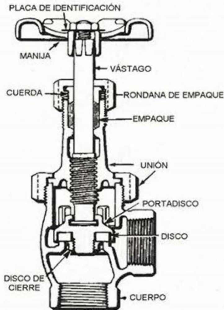
VÁLVULA DE ÁNGULO
