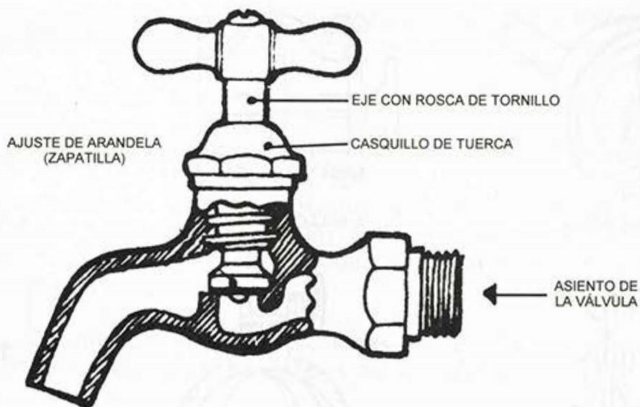
LLAVE DE NARIZ
