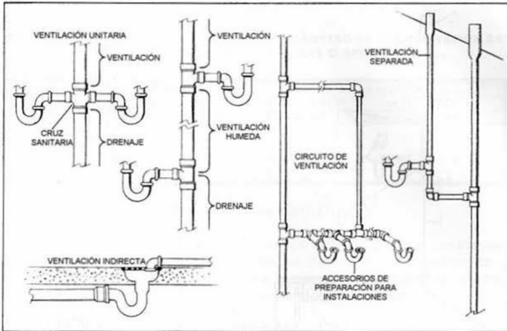
DISTINTAS POSIBILIDADES DE INSTALACIONES PARA VENTILACIÓN
