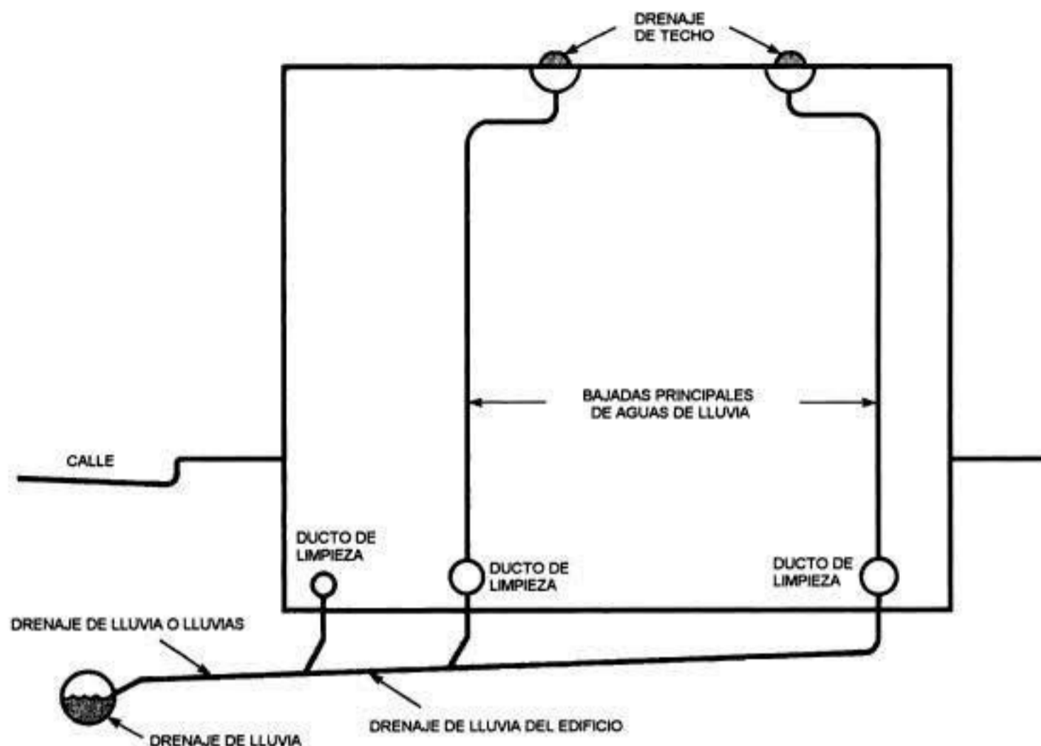
SISTEMA DE DRENAJE DE LLUVIA EN UNA CASA O EDIFICIO
