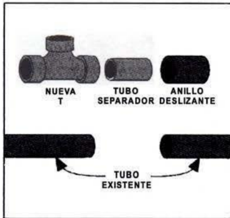
USO DE UNIONES DESLIZANTES
