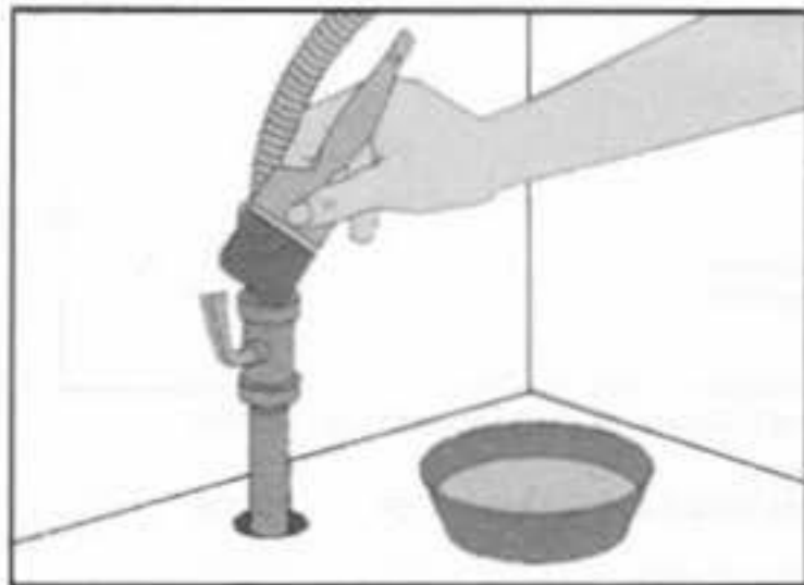
5 SE ABRE LA VÁLVULA DE CORTE Y UN QUEMADOR HASTA QUE SE SIENTA OLOR A GAS Y SE VERIFICAN FUGAS, APLICANDO AGUA CON JABÓN EN LAS UNIONES.
