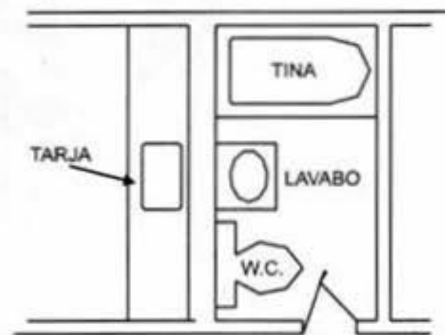
INSTALACIÓN DE PLOMERÍA ESPALDA A ESPALDA (COCINA EN BAÑO)
