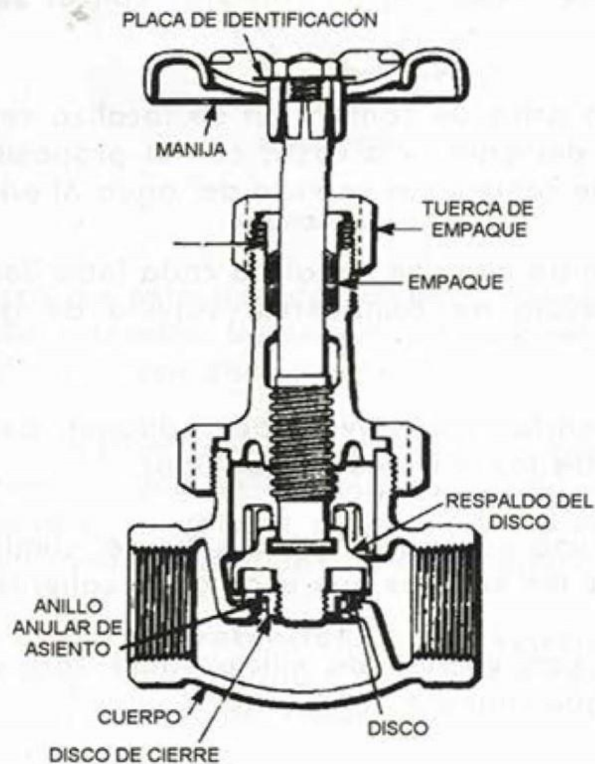
PARTES DE UNA VÁLVULA DE GLOBO
