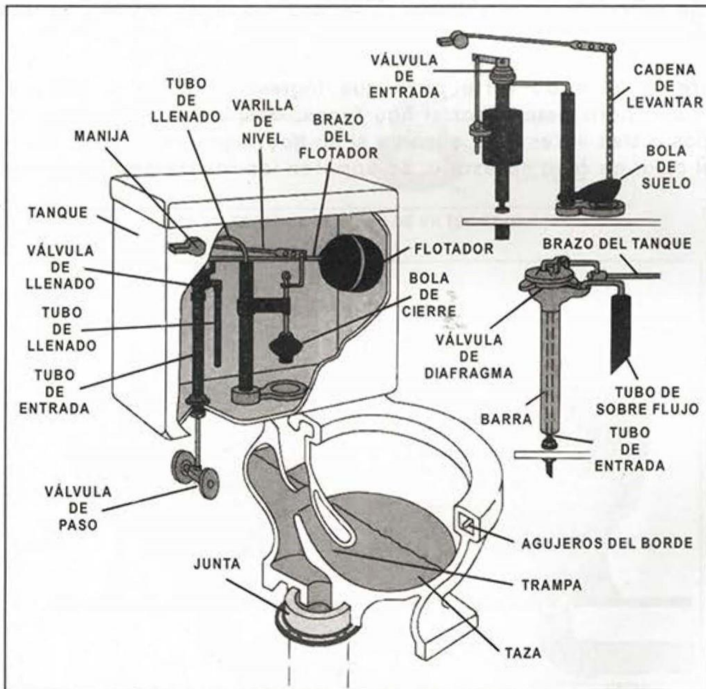
ELEMENTOS DE UN TOILET (W.C.)
