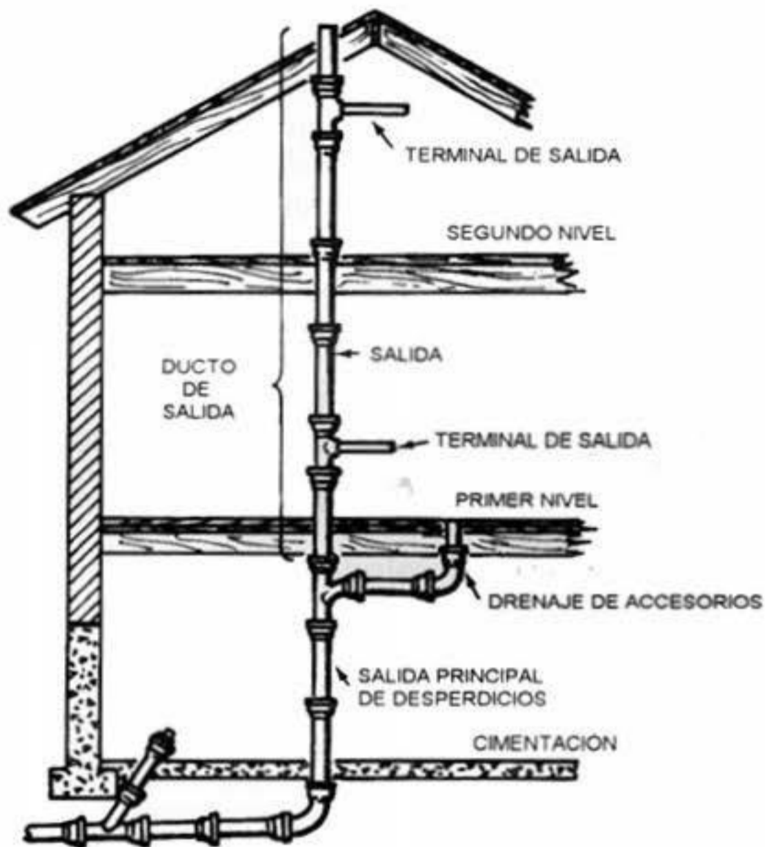
SISTEMA DE DUCTOS DE SALIDA PARA DRENAJE
