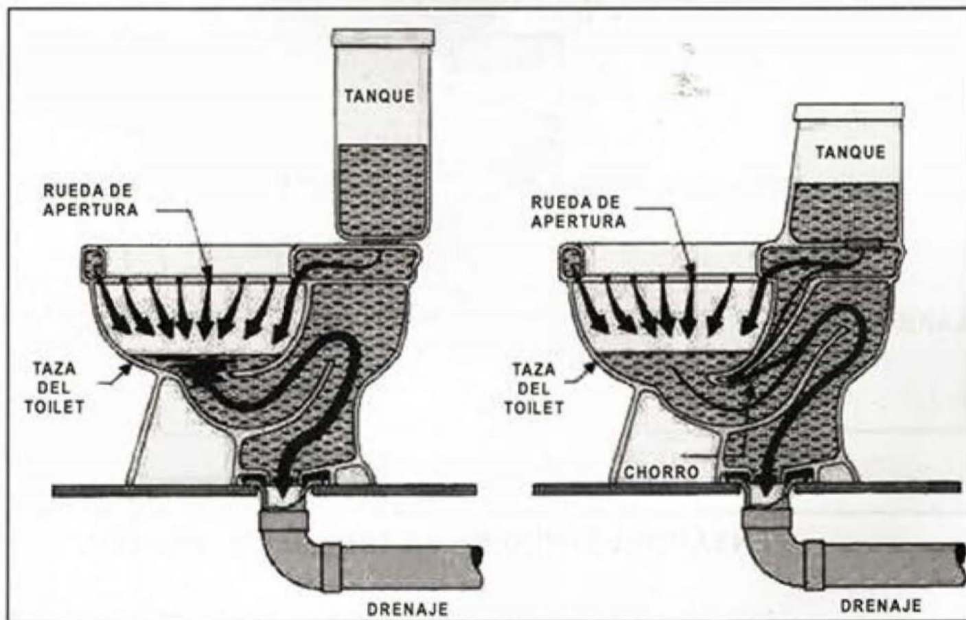
LOS NIVELES DE AGUA MOSTRADOS SON DURANTE LA DESCARGA
