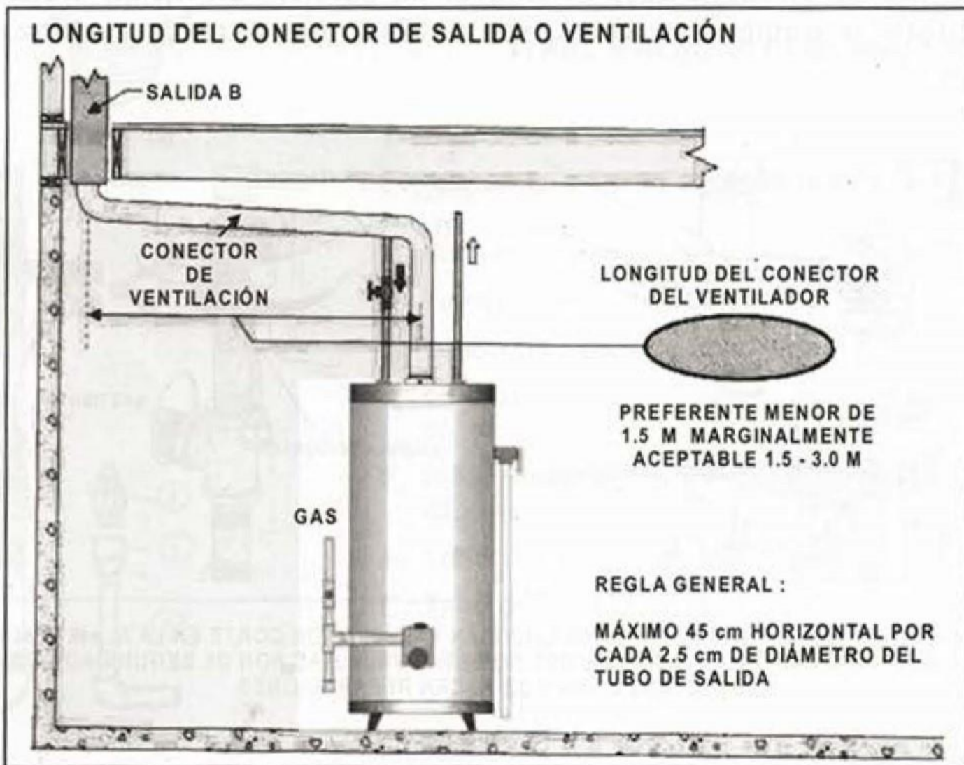
INSTALACIÓN DE UN CALENTADOR DE GAS
