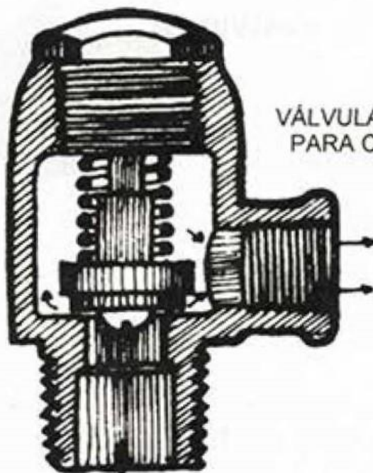
VÁLVULA O LLAVE DE CUADRO
