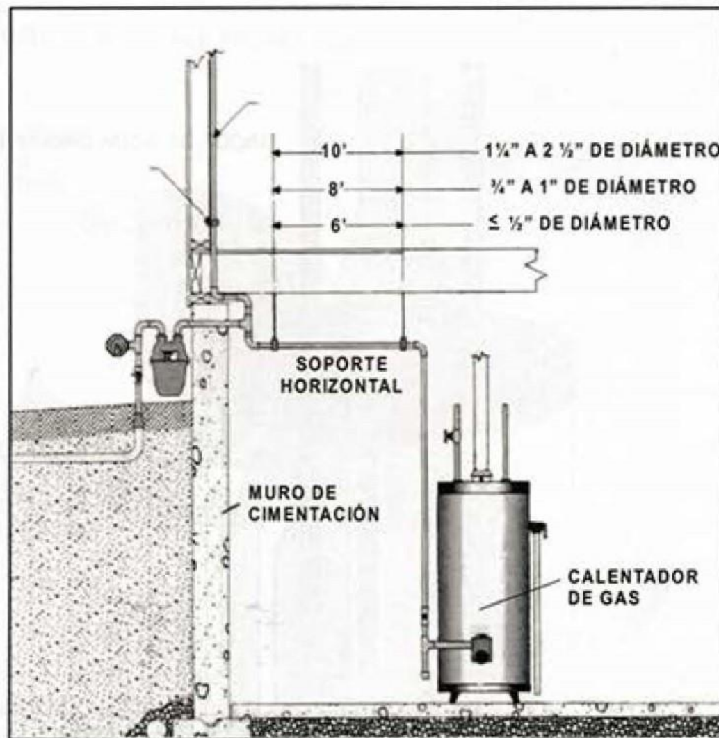
TUBERÍA PARA ALIMENTACIÓN DE GAS NATURAL
