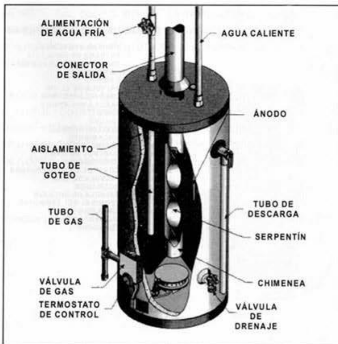
CALENTADOR DE AGUA A BASE DE GAS
