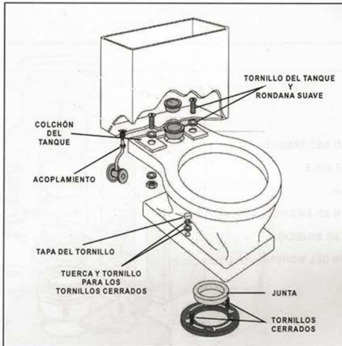
FASES DE MONTAJE DE UN TOILET (W.C.)
