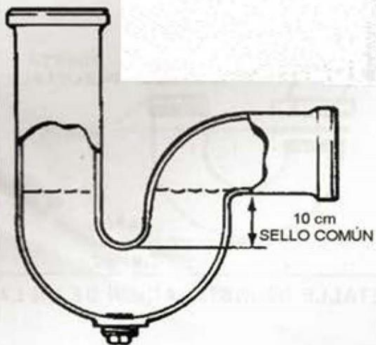
TRAMPA DE SIFÓN PROFUNDO
