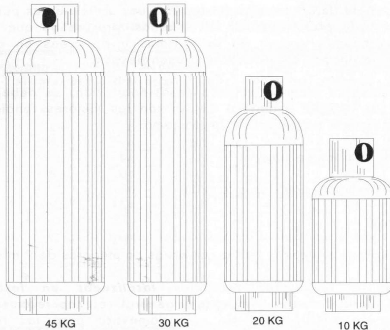
CAPACIDADES DE RECIPIENTES PORTÁTILES
