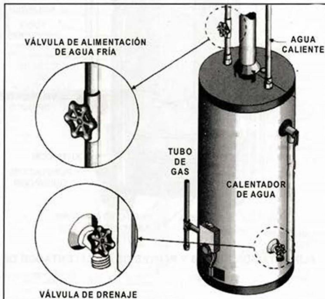
LOCALIZACIÓN DE VÁLVULAS EN UN CALENTADOR DE AGUA
