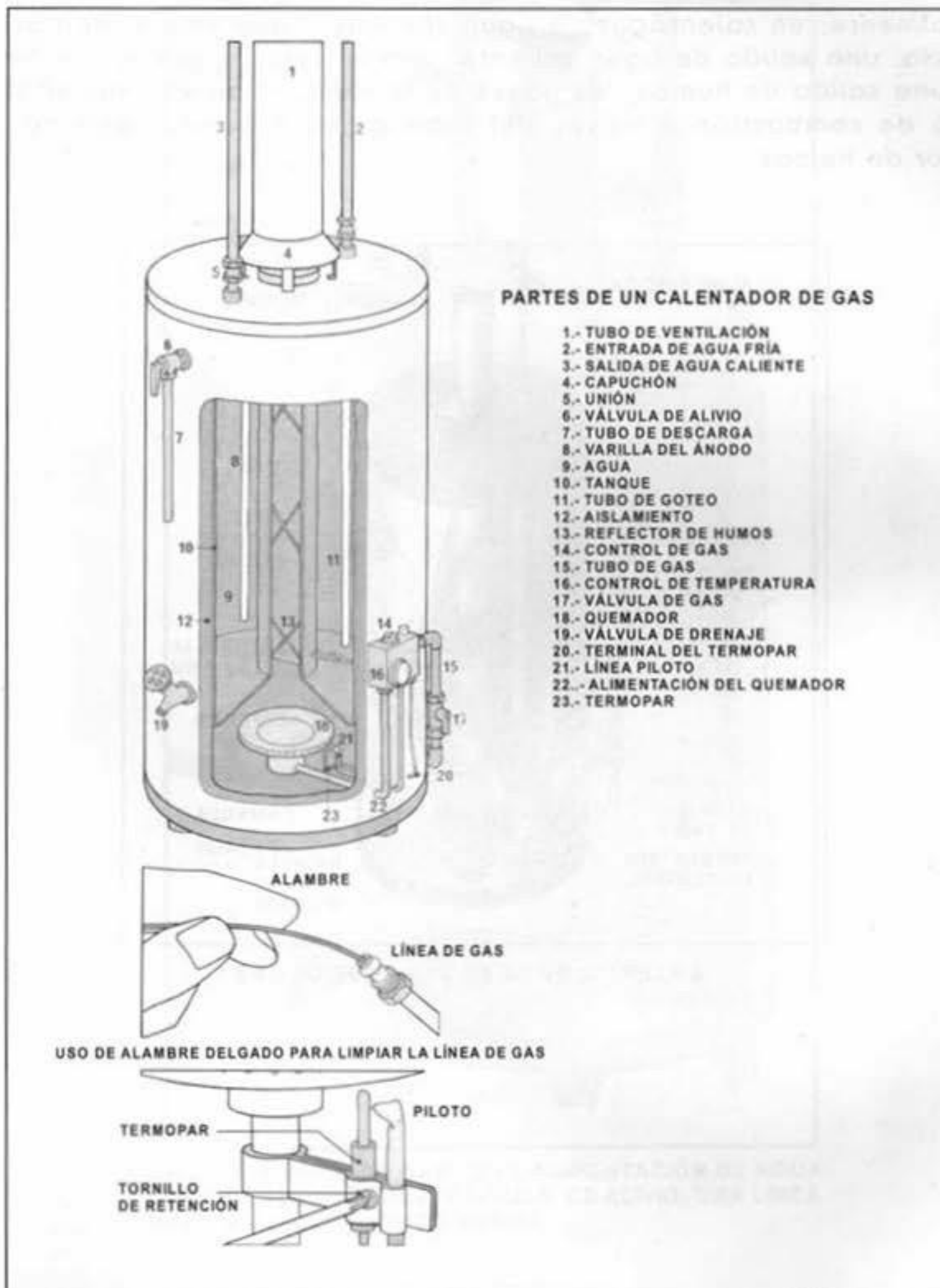
COMPONENTES DE UN CALENTADOR DE GAS
