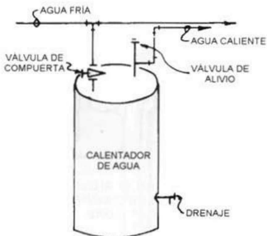
ELEMENTOS DE LA INSTALACIÓN HIDRÁULICA EN UN CALENTADOR DE AGUA
