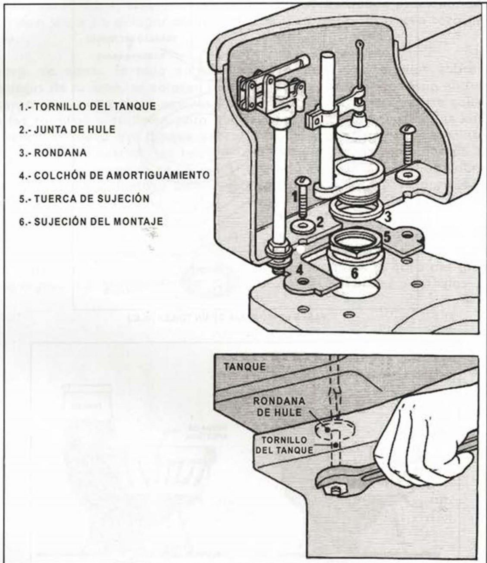
ENSAMBLE TÍPICO DE UN TANQUE DE TOILET
