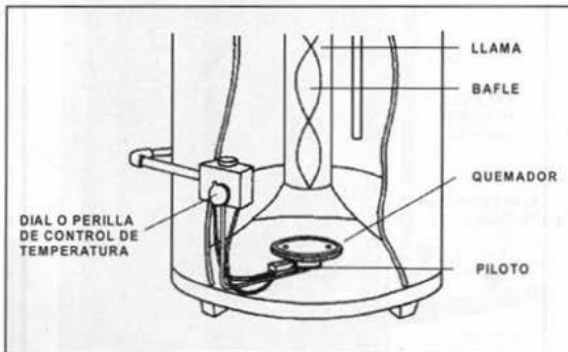
CORTE DE UN QUE MADOR MOSTRANDO EL PILOTO
