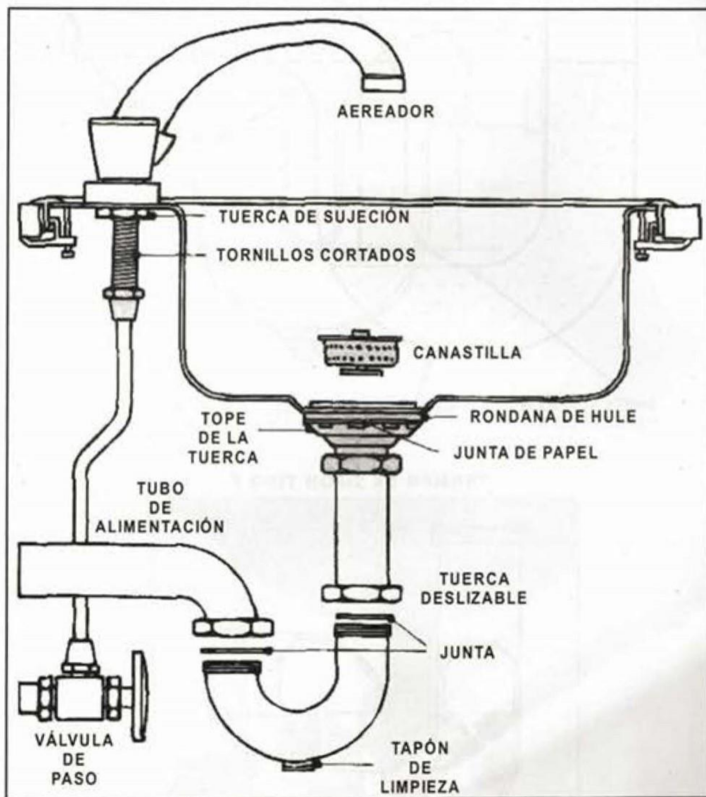
DETALLE DE INSTALACIÓN DE UN LAVABO
