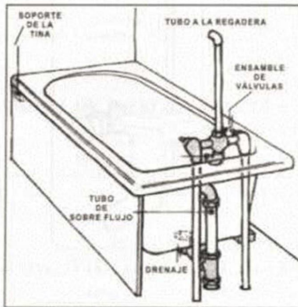
MONTAJE DE UNA TINA
