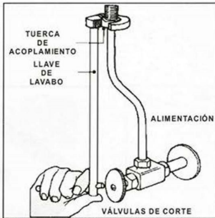
SE DESCONECTA LA ALIMENTACIÓN DE LA LLAVE DEL LAVABO
