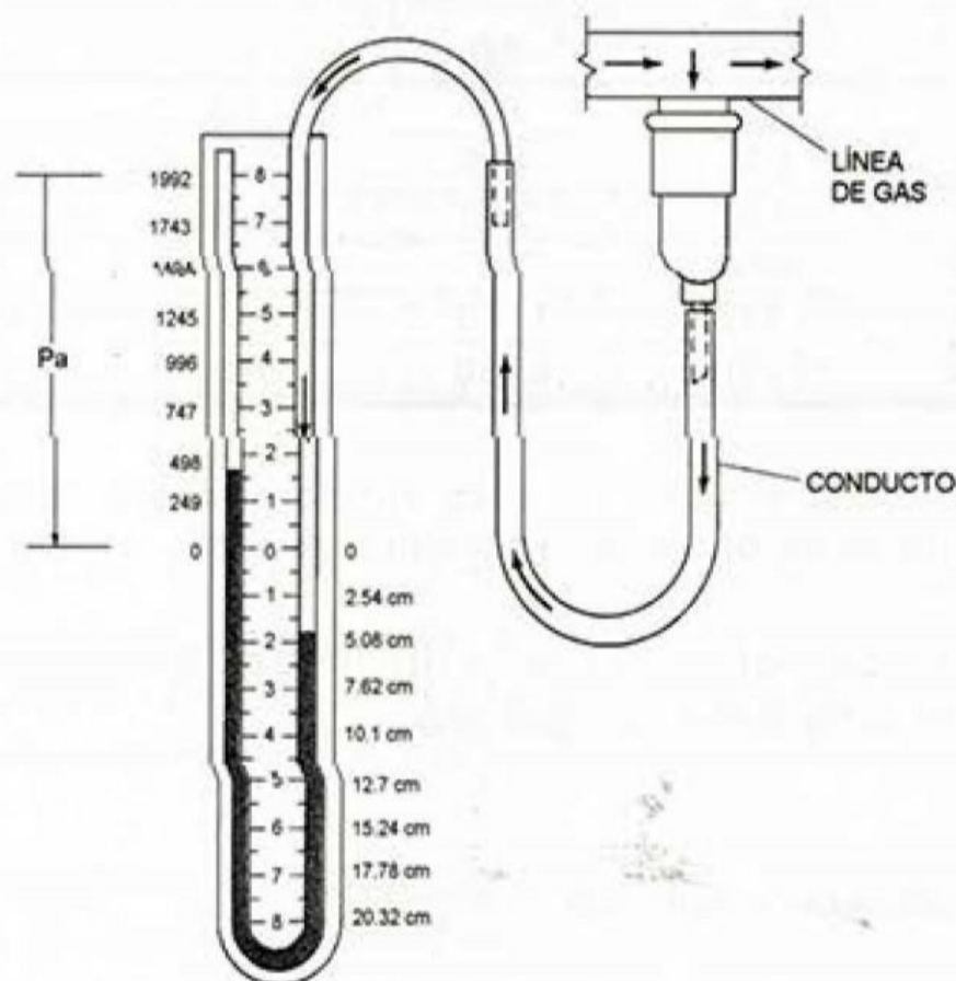
MANÓMETRO DE TUBO EN U EN QUE SE LEE 3.5 PULG (8.9 cm) EN COLUMNA DE AGUA
