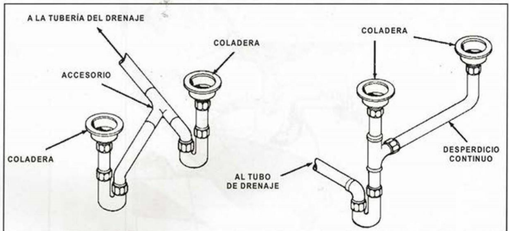
MÉTODOS DE CONEXIÓN DE LOS FREGADEROS O LAVAPLATOS DE COCINA
