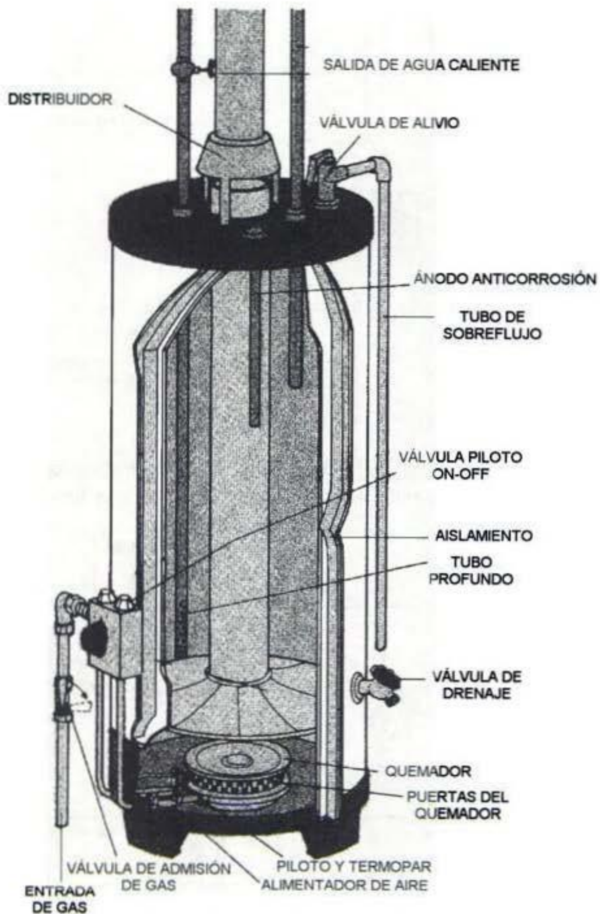
ALIMENTACIÓN DE GAS Y PARTES DE UN CALENTADOR DE GAS
