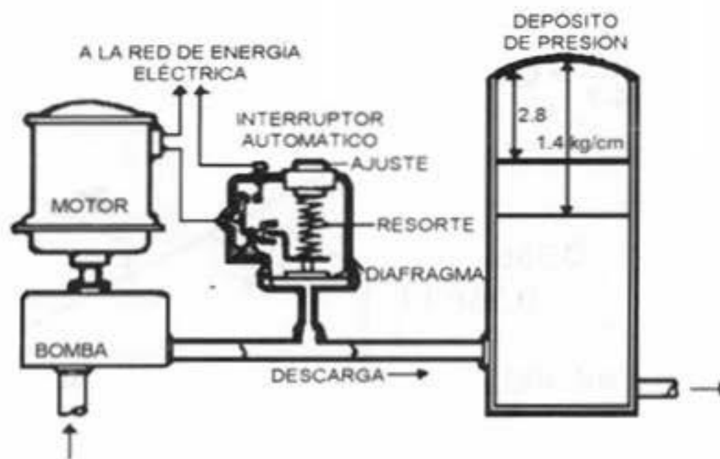
TANQUE HIDRONEUMÁTICO PARA POZO
