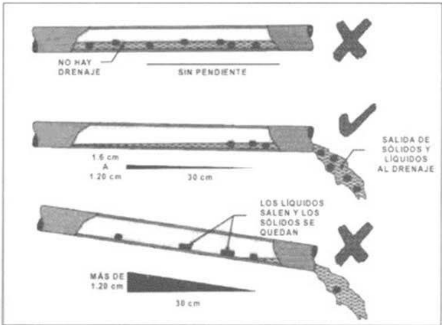
EFFECTO DE LA PENDIENTE EN LOS DRENAJES
