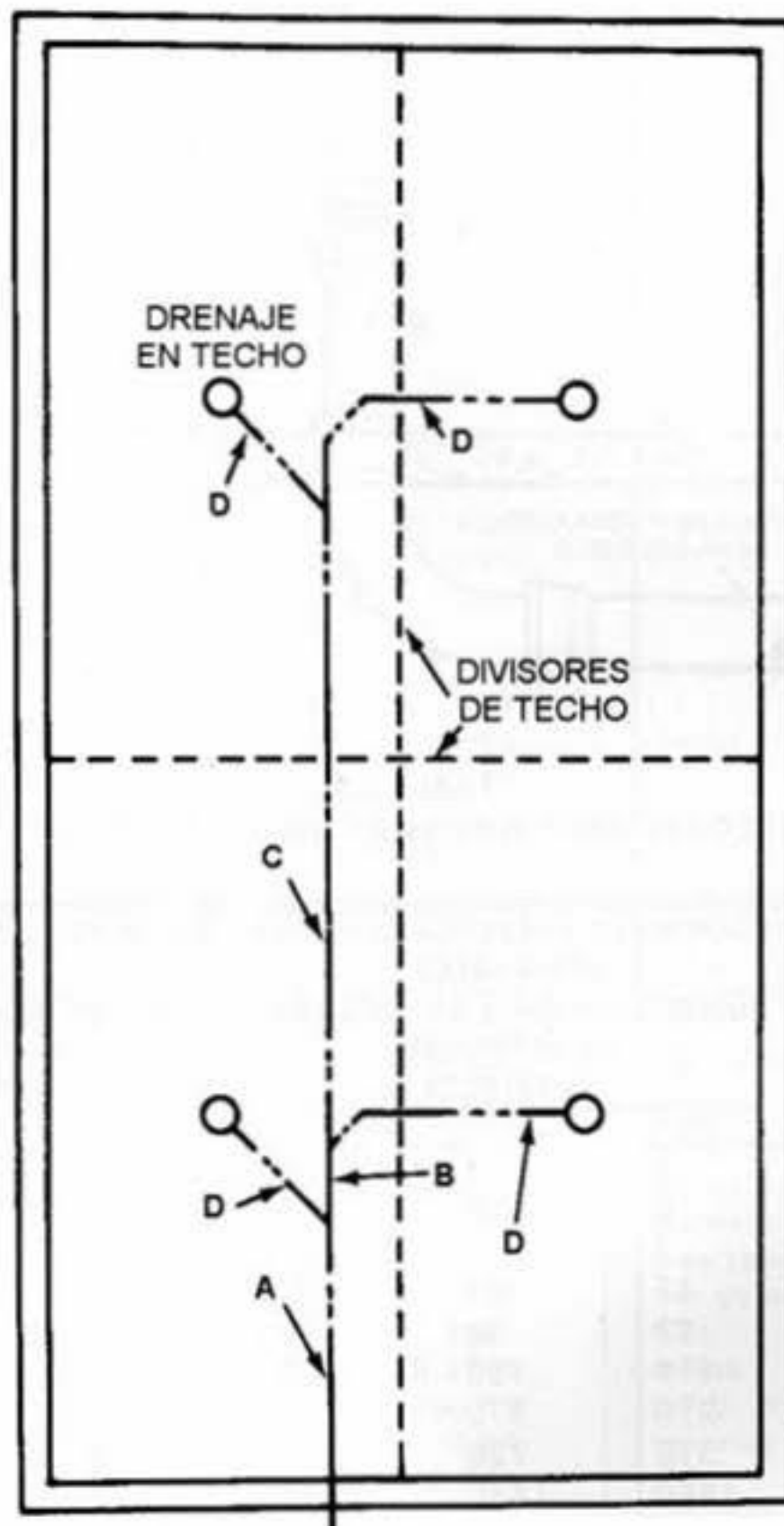
TUBERÍA DE DRENAJE DE LLUVIA EN UNA CONSTRUCCIÓN
