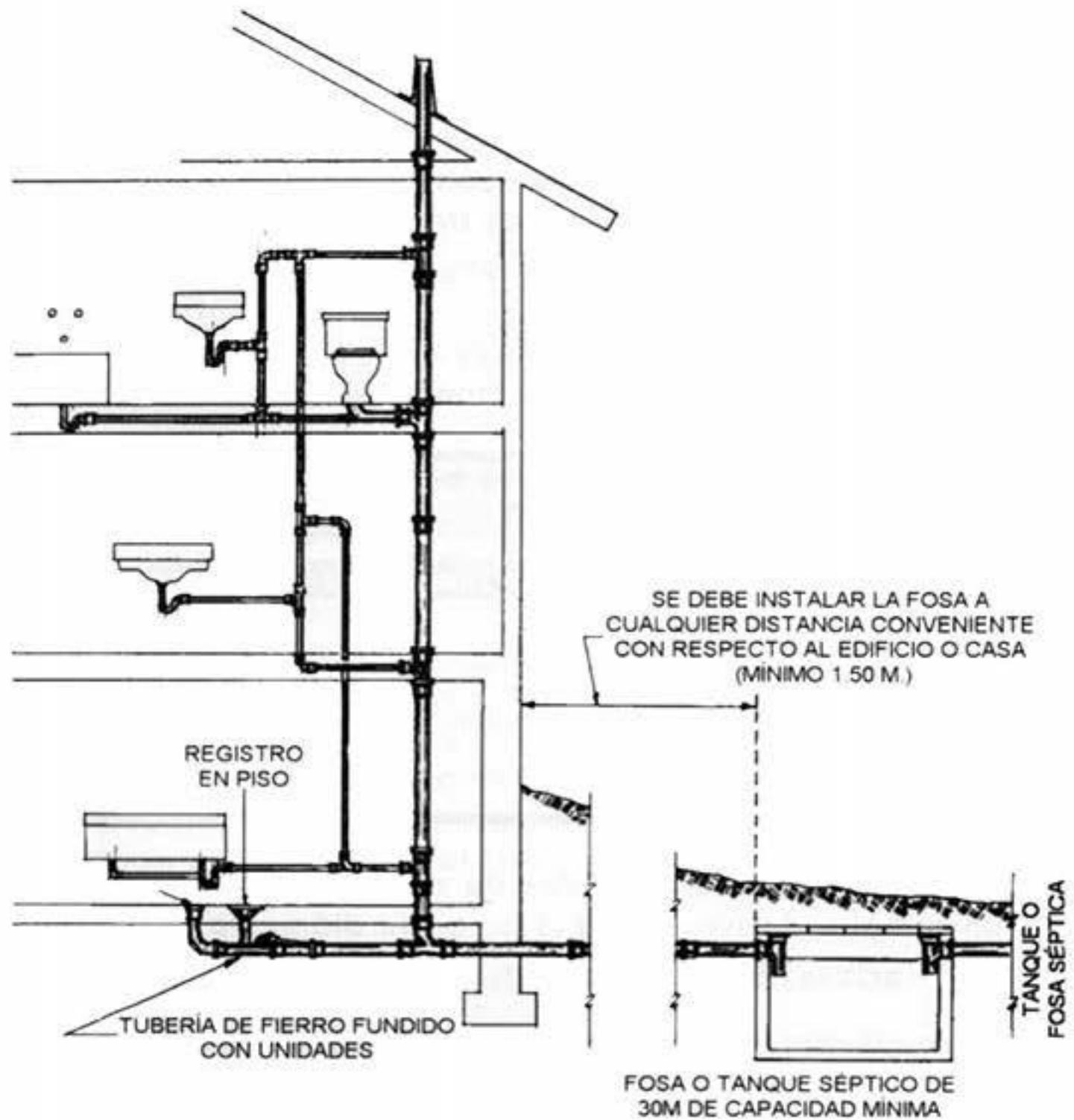
ARREGLO TÍPICO DE LA TUBERÍA Y DETALLES DEL USO DE UN TANQUE O FOSA SÉPTICA
