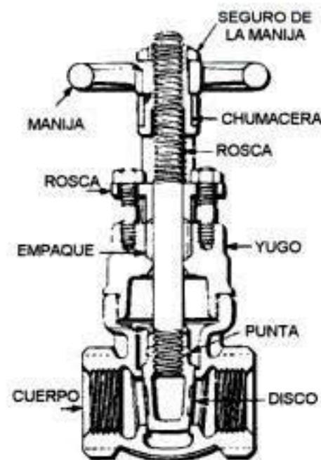
VÁLVULA DE COMPUERTA CON DISCO SECCIONADO
