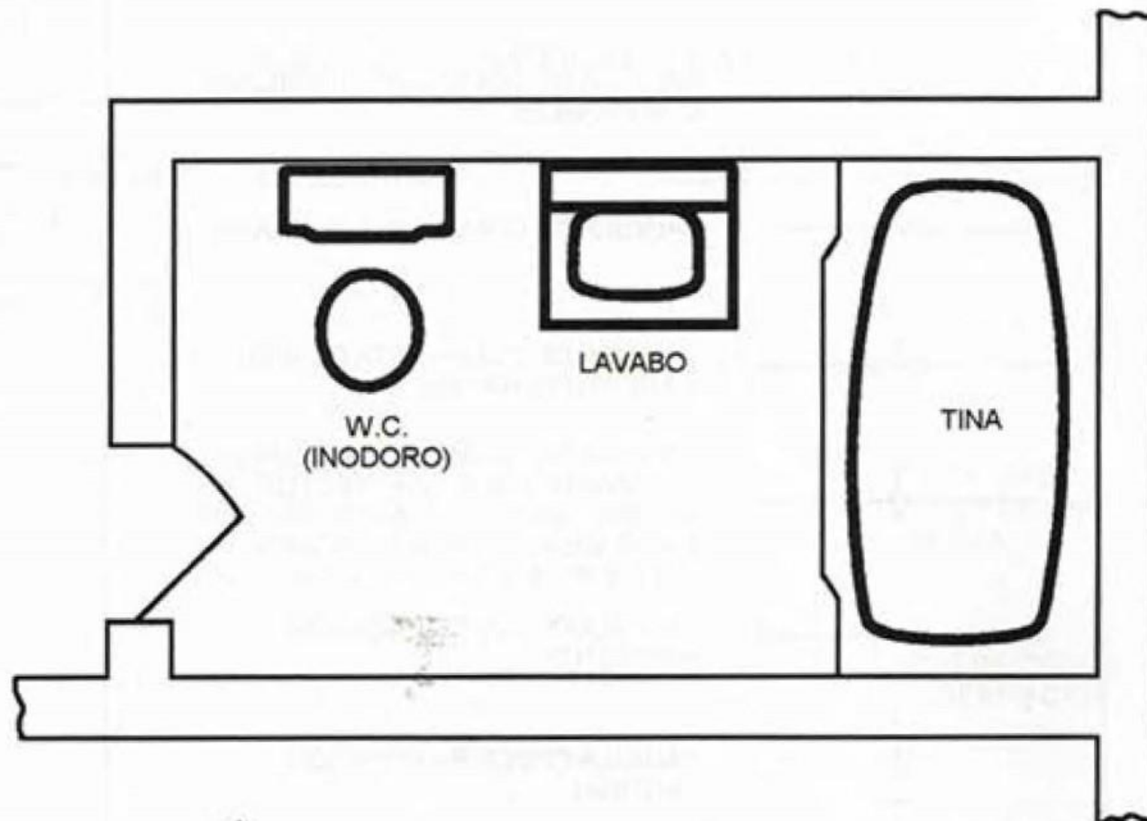
VISTA EN PLANTA DE LOS ACCESORIOS DE BAÑO
