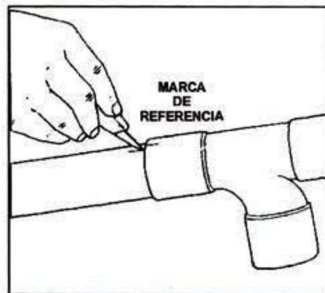
4.- MARCAR EL CONECTOR Y EL TUBO PARA REFERENCIA DE ALINEACIÓN
