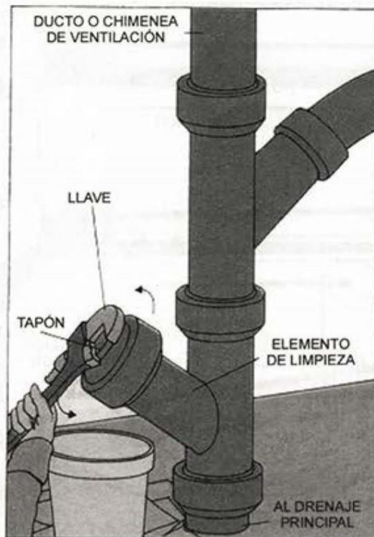
DETALLES DE DUCTOS DE VENTILACIÓN
