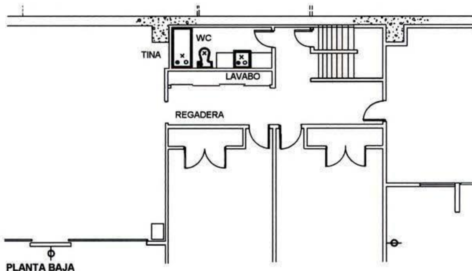
REQUERIMIENTOS DE SUMINISTRO DE AGUA Y DRENAJE
