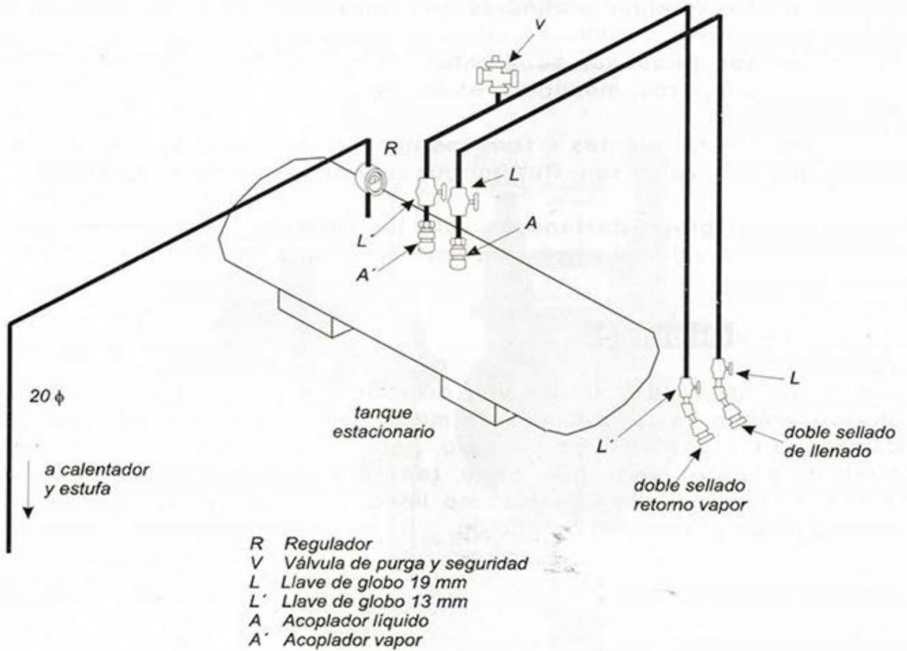
DIAGRAMA BÁSICO DE INSTALACIÓN DE UN TANQUE ESTACIONARIO
