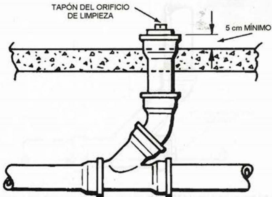
SALIDA PARA DRENAJE EN UNA CONSTRUCCIÓN
