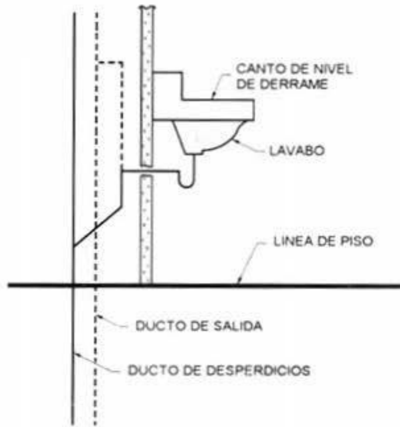
SISTEMA INDIVIDUAL DE SALIDA PARA UN LAVABO FIJO EN MURO
