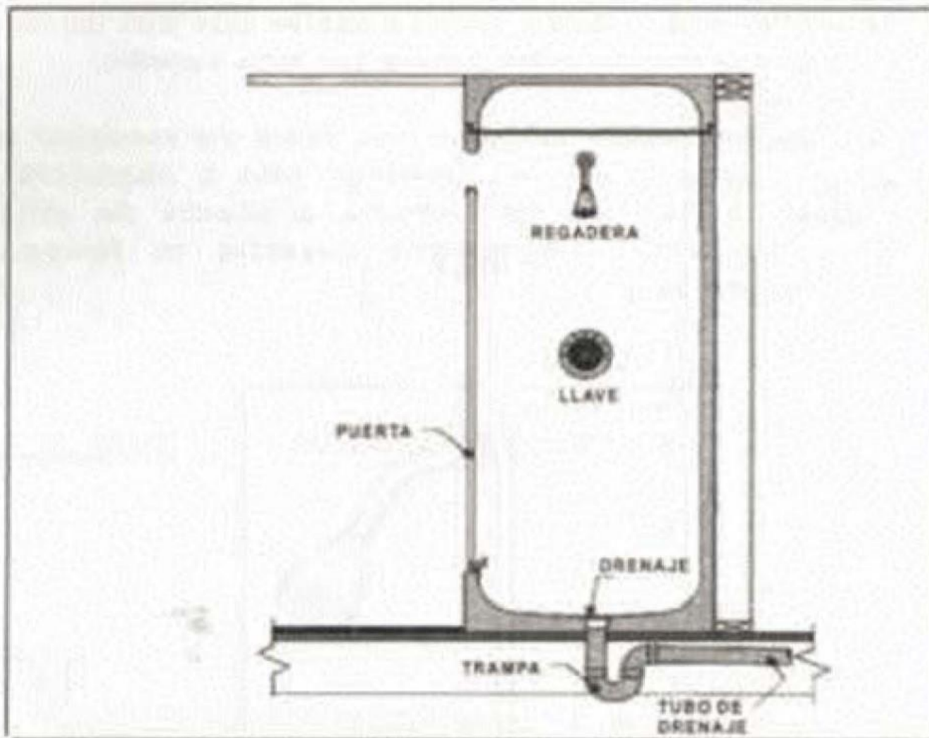
SISTEMA DE DRENAJE EN UNA REGADERA DE BAÑO
