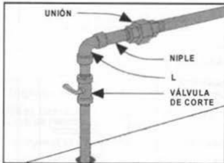
3 PARA CONEXIONES RÍGIDAS SE USAN NIPLES Y UNIONES L.
