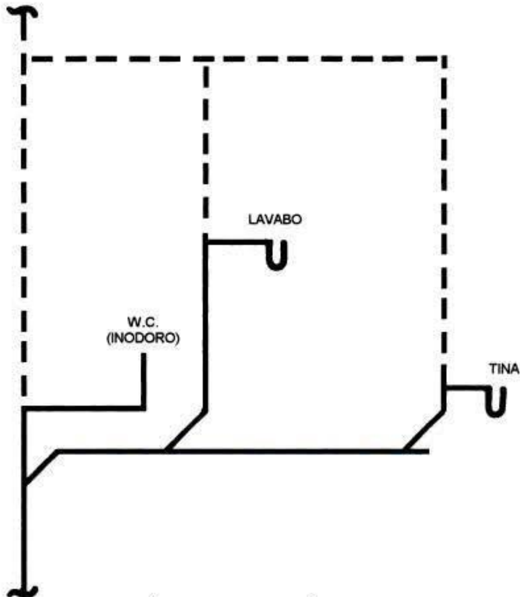
DIBUJO ESQUEMÁTICO DE LA TUBERÍA DEL DRENAJE SANITARIO Y VENTILACIÓN DEL BAÑO DE LA FIGURA ANTERIOR
