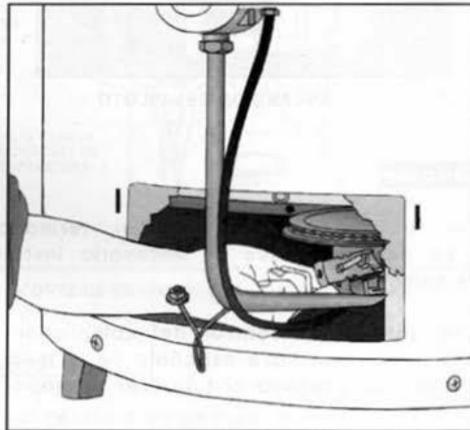
INSTALANDO UN TERMOPAR NUEVO
