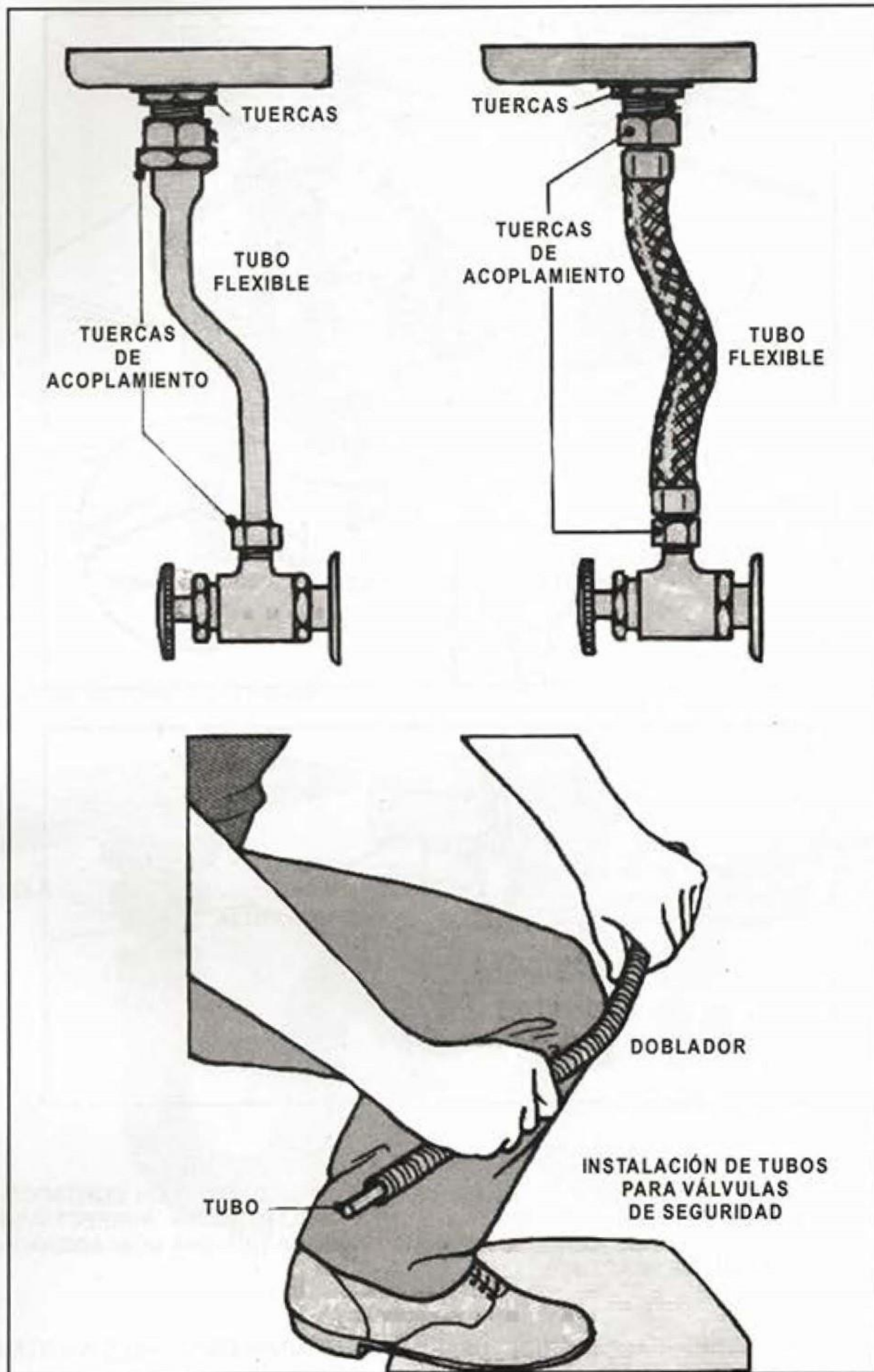
USO DE DOBLADOR DE TUBO
