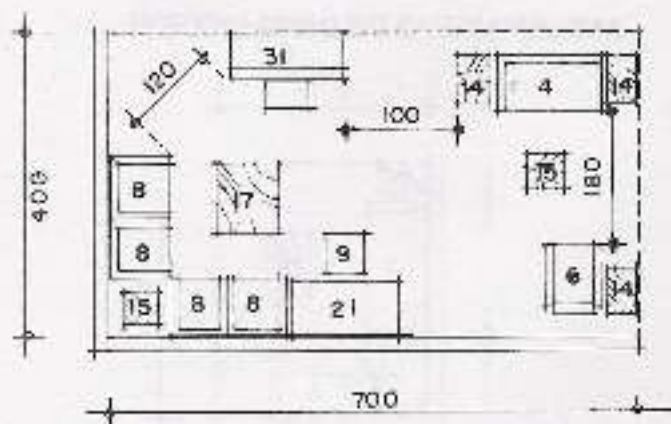
2.20. Espacio grande para dos grupos de conversación.
