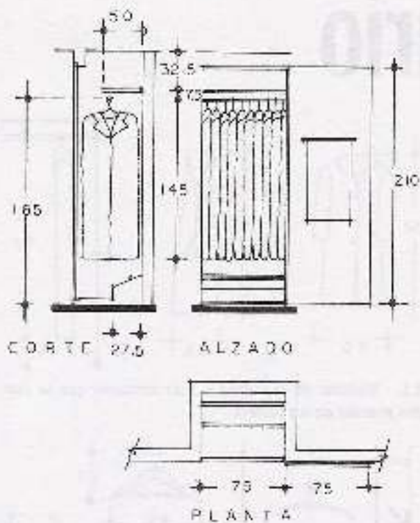
9.5. Closet sencillo para 10 trajes colgados, sapateras en la parte alta y zapatos en el piso; la puerta se utiliza para colgar corbatas y cinturones.
