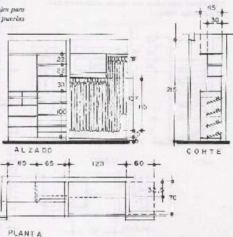
9.14. Closet matrimonial separado en dos secciones, una para camisas y pañuelos y otra para colgar ropa.
