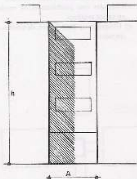
14.2. Dimensionamiento de los patios de luz en los edificios con relación a su altura.
