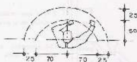
ALCANCES MÁXIMOS Y MÍNIMOS DE UNA PERSONA SENTADA.
