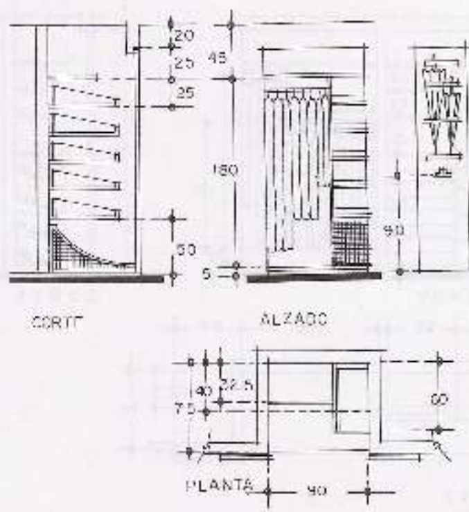
9.11. Espacio para trajes colgados, manijas y cajones: en la parte interior se aprovechan los ganchos.
