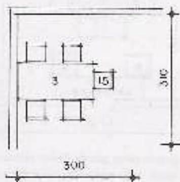
3.13. Solución con mesa pegada a la pared, 9,30 \text{ m}^2 .
