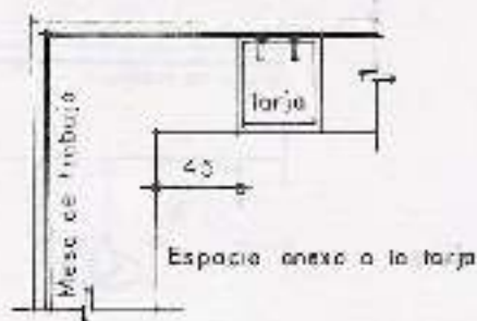
4.10. Las tarjas que no cuentan con escudero integral requieren de un espacio mínimo de 45 cm.
