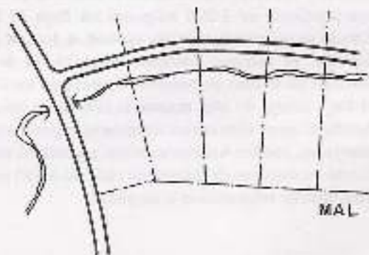
15.7. La ubicación de lotes en curvas de nivel paralelas a la calle aprovechando el drenaje natural del terreno.
