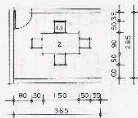
3.14. Mesa para cuatro personas y distancias mínimas de movimiento, 10,40 \text{ m}^2 .
