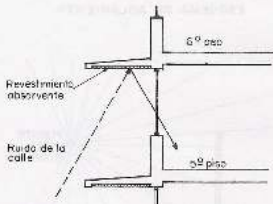
13.25. El ruido reflejado en los elementos de protección puede ser cañado con un revestimiento absorbente.
