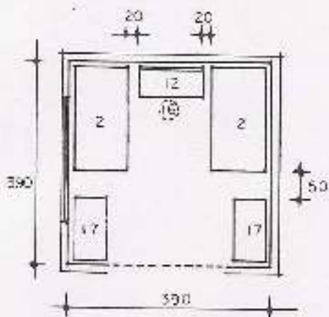
5.24. Otra variante en la misma área: el tocador sustituye las mesas de noche. 15,21 \text{ m}^2 .
