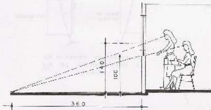
4.5. Las ventanitas deben permitir la supervisión del patio o el lugar de juego de los niños (líneas visuales).
