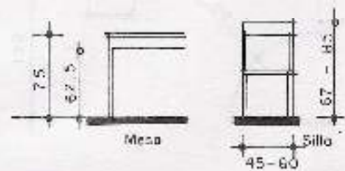
3.6. Dimensiones límite de los muebles del comedor.
