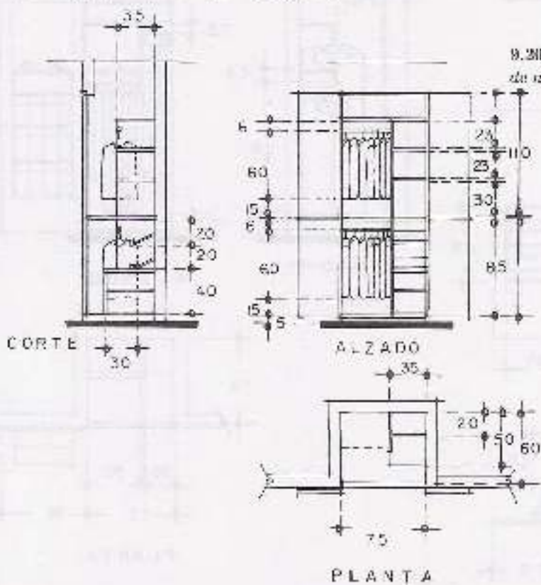
9.19. Unidad separada horizontalmente para colgar trajes cortos.
