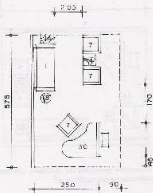
2.25. Un grupo primario en paralelo y plano de cola (30); el ancho del espacio se reduce al mínimo.
