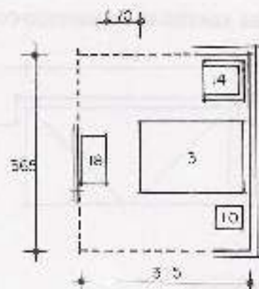
5.19. Cama matrimonial con salón individual. 11.49 m 2
