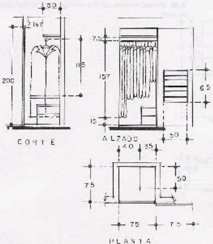
9.16. Closet sencillo con puerta abatible.
