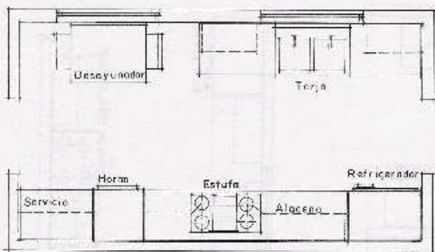
4.26. Disposición en paralelo de una planta rectangular. El ancho se reduce al mínimo. Permite incluir desayunador para 2 ó 3 personas.
