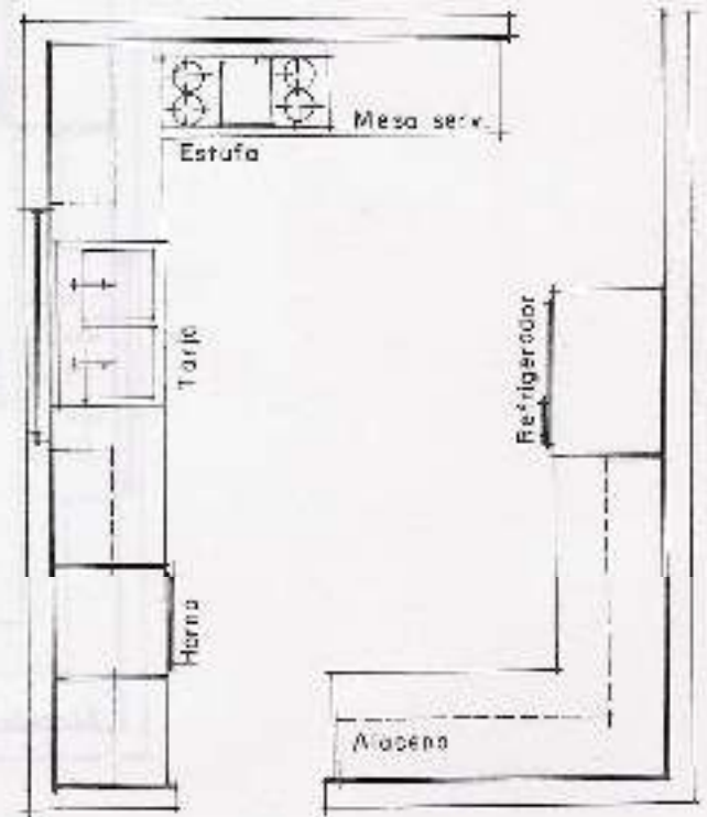
4.25. Solución en doble "U".
