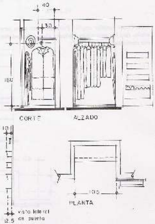
9.12. Closet sencillo sin manijas. Las cajas de la parte interior de la puerta se usan para calzoncillos y zapatos.
