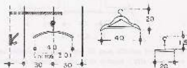
9.2. Tipos de percheros para ropa y sus medidas.
