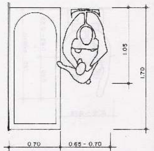
6.6. Areas aconsejadas.
