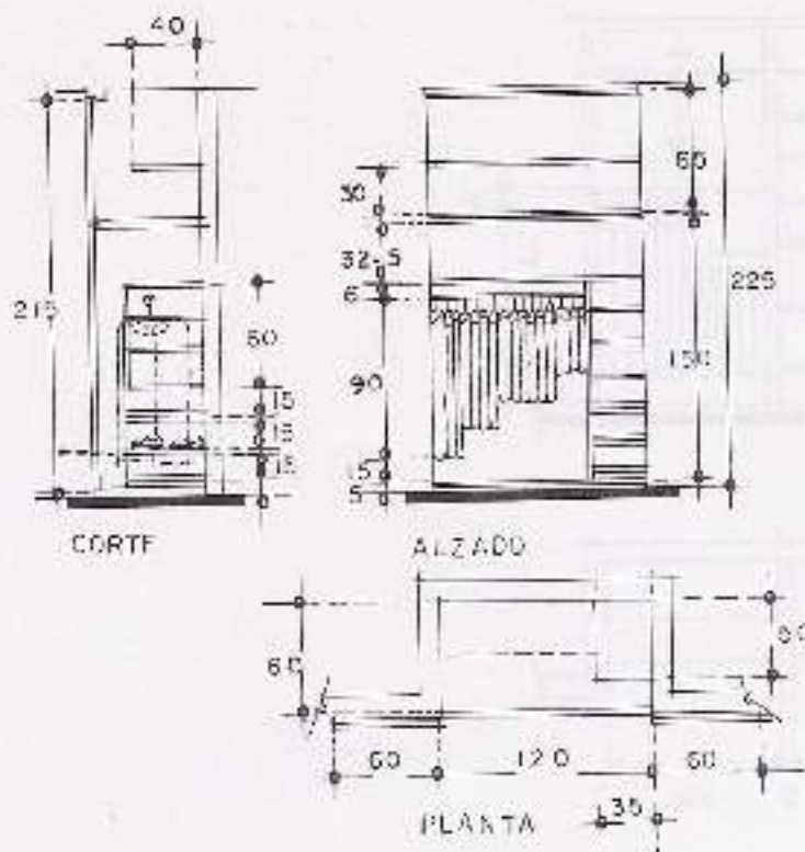
9.10. Closet para niños, con cajones, manijas y espacio para colgar trajes.
