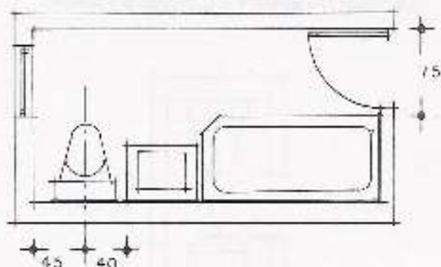
6.19. Baño con tina, lavabo y W.C. alineados.
