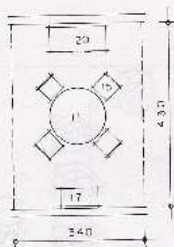
3.19. Mesa redonda para cuatro personas con muebles de almacenamiento. Pueden sentarse seis personas.
