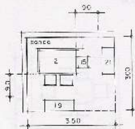
3.18. Banco en esquina y tres sillas. Ahorra de espacio que permite incluir los muebles de almacenamiento.
