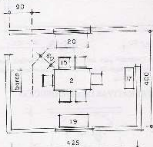
3.20. Comedor grande en un área de 17.00 m 2 .
