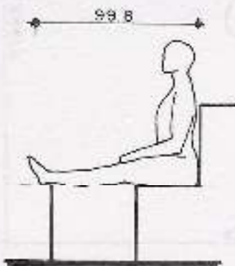
1.17.(A) Distancia máxima para la colocación de taburetes o elevar los pies a la altura de la superficie del asiento.
