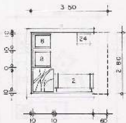
2.14. Solución en escuadra con T.V. y mesa esquinera; superficie de 9.80 m 2 .
