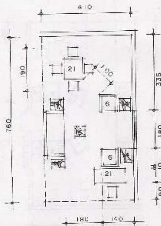
2.26. Un grupo grande cerrado por una circulación central que conecta al escritorio (21) y a la mesa de juego. 31 m 2 .
