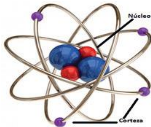
Zonas específicas del átomo
