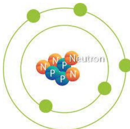
Los neutrones son partículas sin carga eléctrica.
