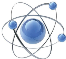
Estructura del átomo.
