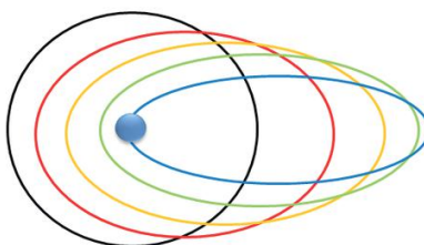
Los electrones pueden girar en órbitas elípticas.
