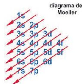
Esquema del llenado de los orbitales atómicos.
