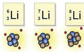
Isótopos del litio
