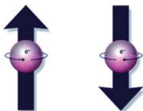
Los electrones pueden rotar alrededor de su eje.
