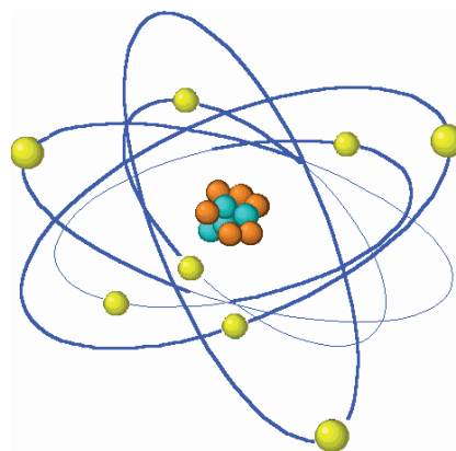
El átomo posee un núcleo positivo muy pequeño, alrededor del cual se mueven los electrones.
