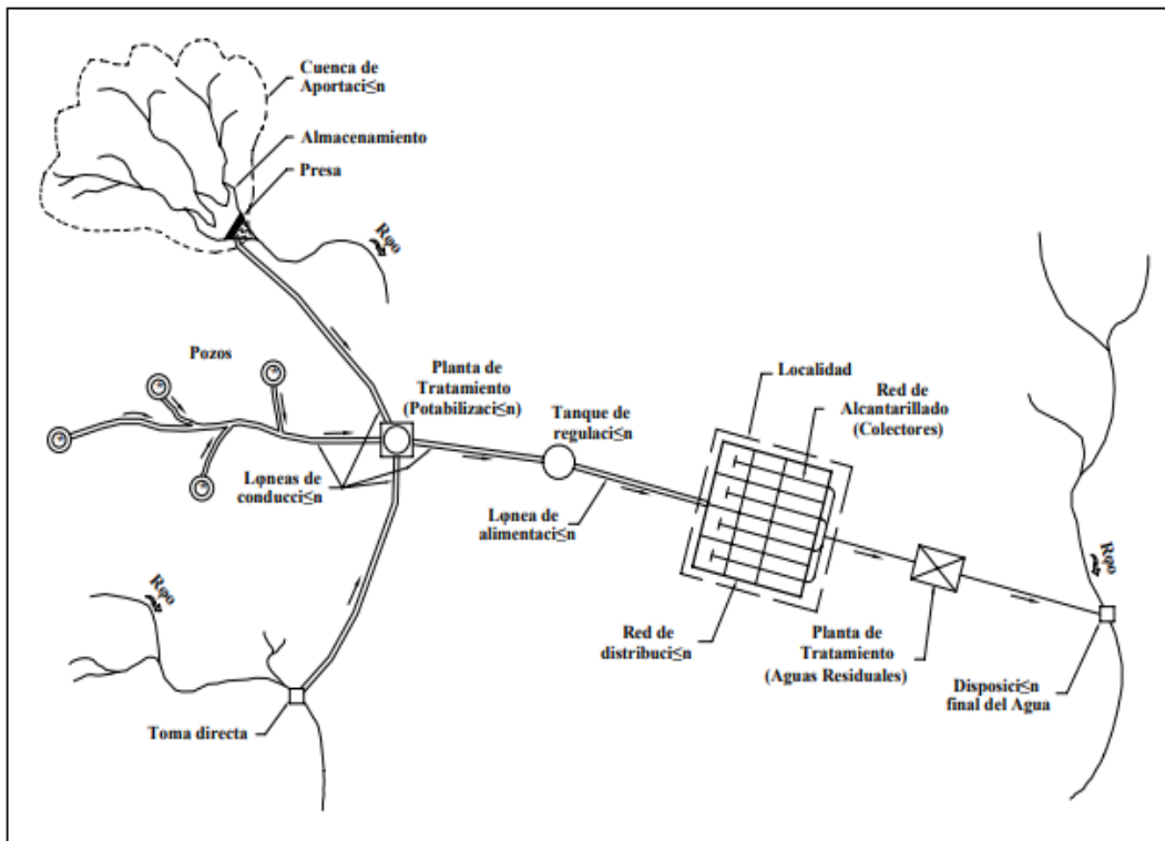
Figura 1.1 Configuración típica de un sistema de abastecimiento de agua en localidades urbanas
